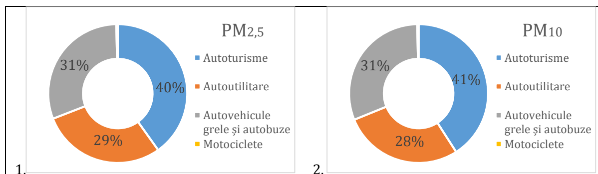
Figura nr. 3-14 - Contribuția diferitelor categorii de autovehicule la emisiile de poluanți în atmosferă
