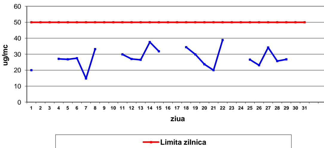
Evoluție pulberi in suspensie - PM10 concentratii zilnice in luna iulie 2016
