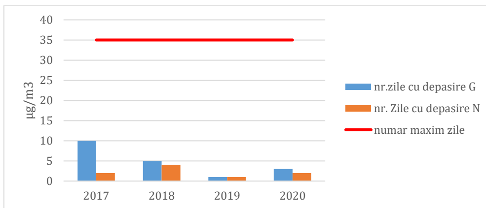
Fig. nr.5-.Evoluția numărului anual de zile pentru care concentrația medie zilnică a depășit valoarea de 50 µg/m 3 , pentru PM 10 , pentru perioada 2017 – 2020
