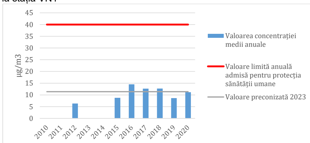
Fig. nr. 3-Evoluția concentrației medii anuale pentru NO 2 , pentru perioada 2010 – 2020, la stația VN1
