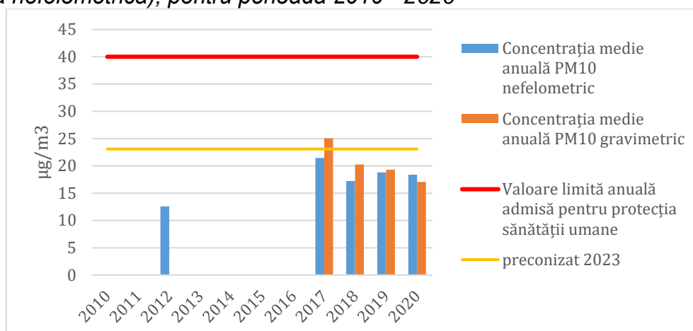
Fig. nr. 4- Evoluția concentrației medii anuale pentru PM10 (metoda gravimetrică+ metoda nefelometrică), pentru perioada 2010 - 2020
