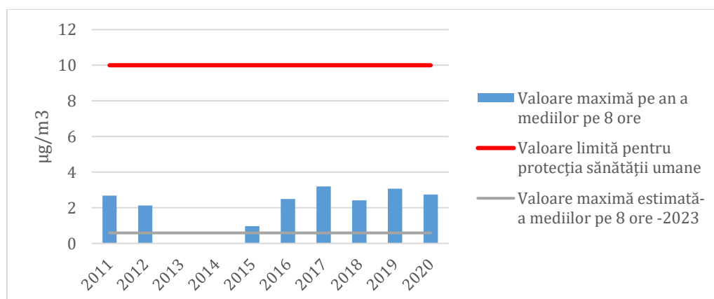
Fig. nr. 7-Evoluția valorilor maxime a mediilor pe 8 ore, pe an, pentru CO, pentru perioada 2011 – 2020, și a valorii estimate pentru 2023- la stația VN
