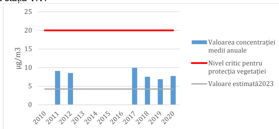
Fig. nr. 6-Evoluția concentrației medii anuale pentru SO 2 , pentru perioada 2010 – 2020, la stația VN1
