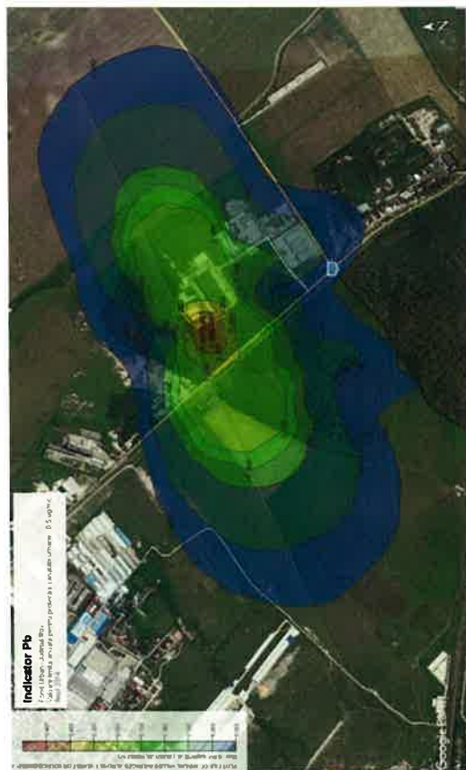
Figura nr. 3-15 Creșterea nivel Fond urban – industrie – indicator Pb, medie anuală
