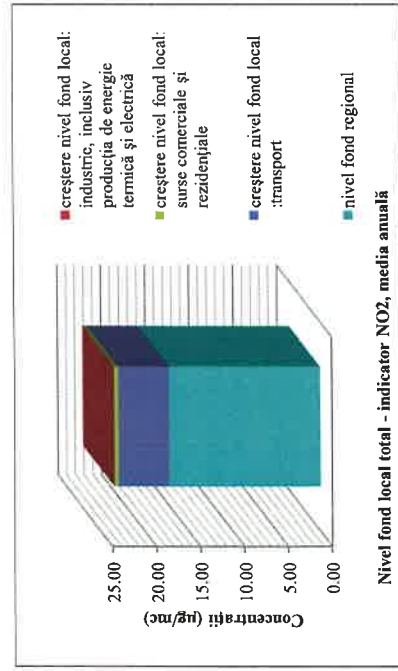
Figura nr. 3-63 Nivel Fond local total – indicator NO2
