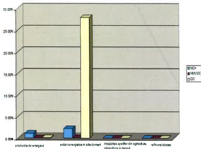
2014 AN DE REFERINȚĂ Contribuția sectoarelor de activitate din energie la emisiile de poluanți precursori ai ozonului
