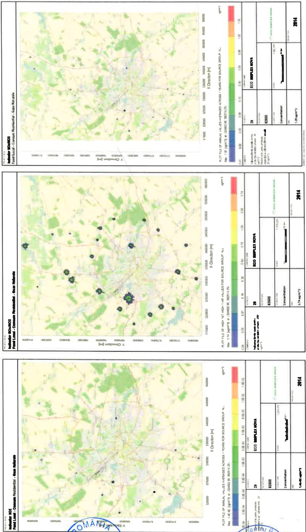
Figura nr. 3-53 Creștere nivel Fond local – consum rezidențial GN – indicator SO2, medie anuală Figura nr. 3-54 Creștere nivel Fond local – consum rezidențial GN – indicator NO2, medie orară Figura nr. 3-55 Creștere nivel Fond local – consum rezidențial GN – indicator NO2, medie anuală
