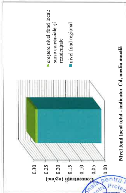
Figura nr. 3-68 Nivel fond local total – indicator Cd
