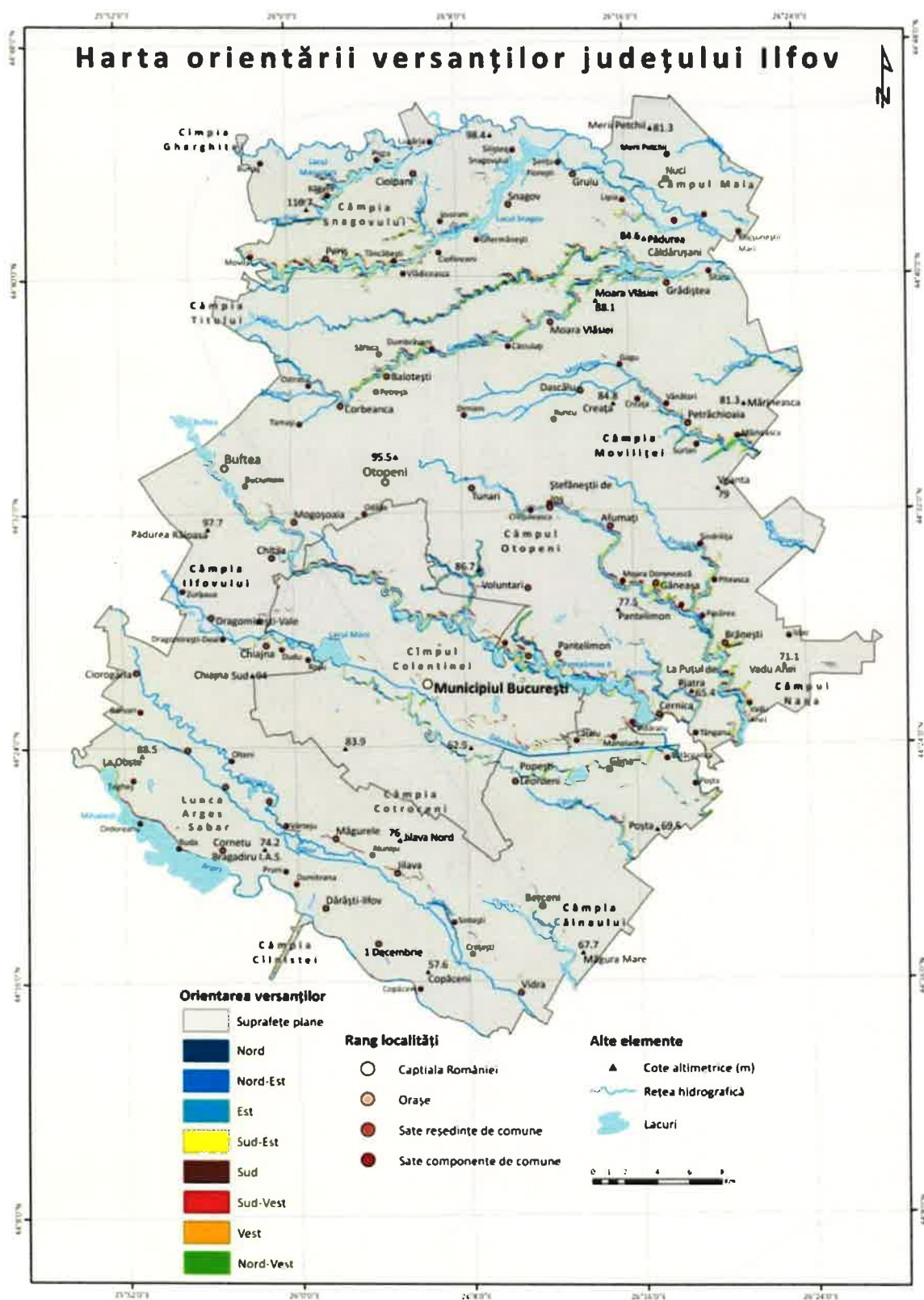
Figura nr. 2-22 Harta orientării versanților județului Ilfov
