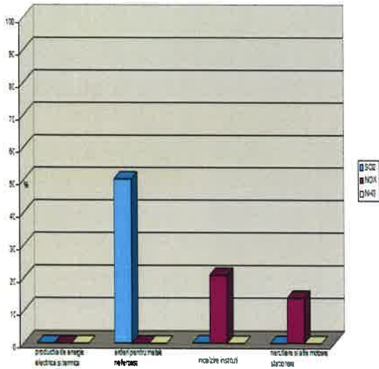
Contribuția sectoarelor de activitate din energie la emisiile de poluanți cu efect de acidifiere
