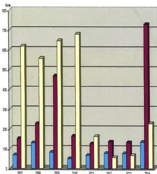
Evoluția emisiilor de poluanți cu efect de acidifiere
