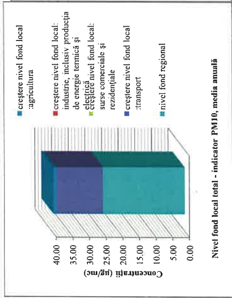
Figura nr. 3-66 Nivel fond local total – indicator PM10
