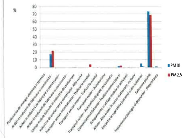
Contribuția sectoarelor de activitate din energie la emisiile de particule primare în suspensie
