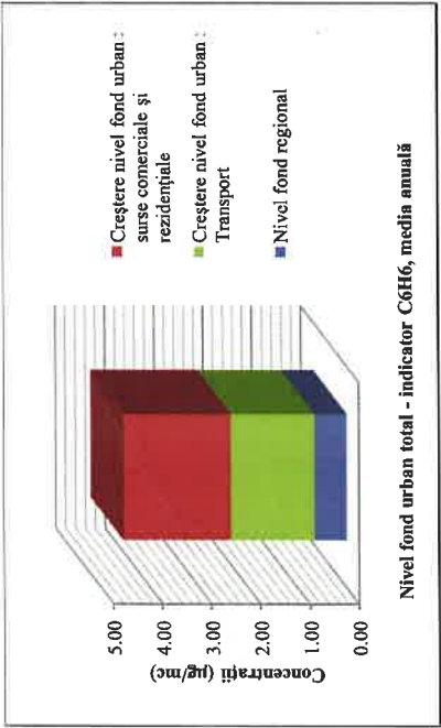
Figura nr. 3-40 Nivel fond urban total – indicator C6H6
