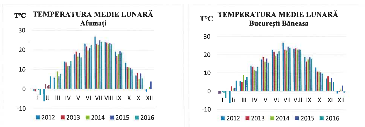
Figura nr. 2-23 Temperatura medie lunară la stațiile Afumați și București Băneasa
