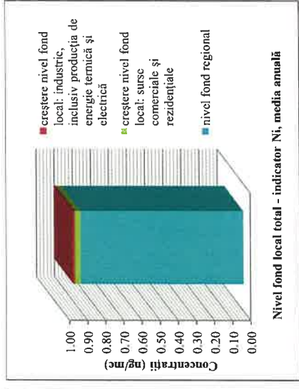
Figura nr. 3-69 Nivel fond local total – indicator Ni
