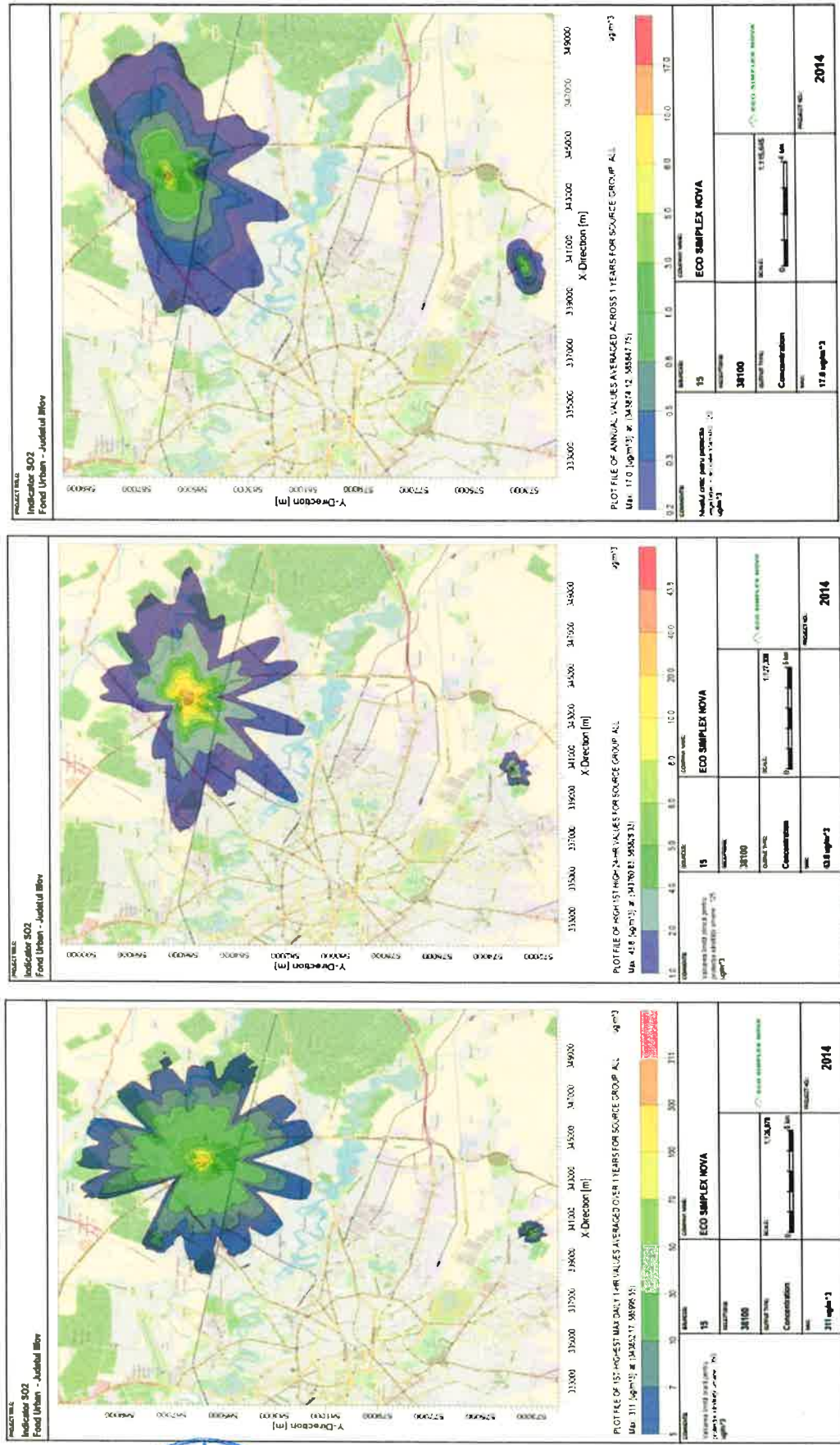
Figura nr. 3-1 Creștere nivel Fond urban – industrie – indicator SO2, medie orară Figura nr. 3-2 Creștere nivel Fond urban – industrie – indicator SO2, medie zilnică Figura nr. 3-3 Creștere nivel Fond urban – industrie – indicator SO2, media anuală
