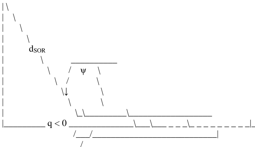
Figura 2.7.r: Geometria la sol aeronavă-observator pentru estimarea corecției de directivitate
