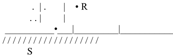
Figura 2.5.j: Diferența traiectoriei în prezența unei difracții: secțiunea transversală actuală (partea superioară), secțiunea transversală nedesfășurată (partea inferioară) În cazul reflexiilor multiple se adaugă reflexiile datorate fiecărei reflexii.
