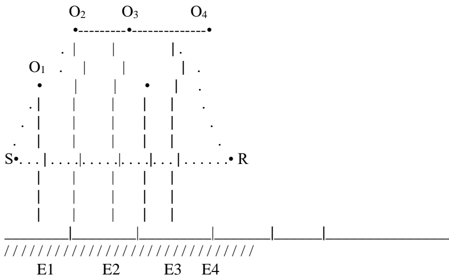
Figura 2.5.f: Exemplu de calcul al diferenței de cale în condiții favorabile, în cazul difracțiilor multiple
