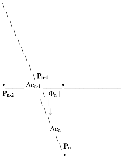
Figura 2.7.v: Parametrii geometrici care definesc condițiile algoritmului de trasare
