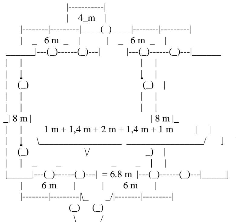
Figura a: exemplu de amplasare a receptoarelor în jurul unei clădiri conform procedurii pentru cazul 1.
