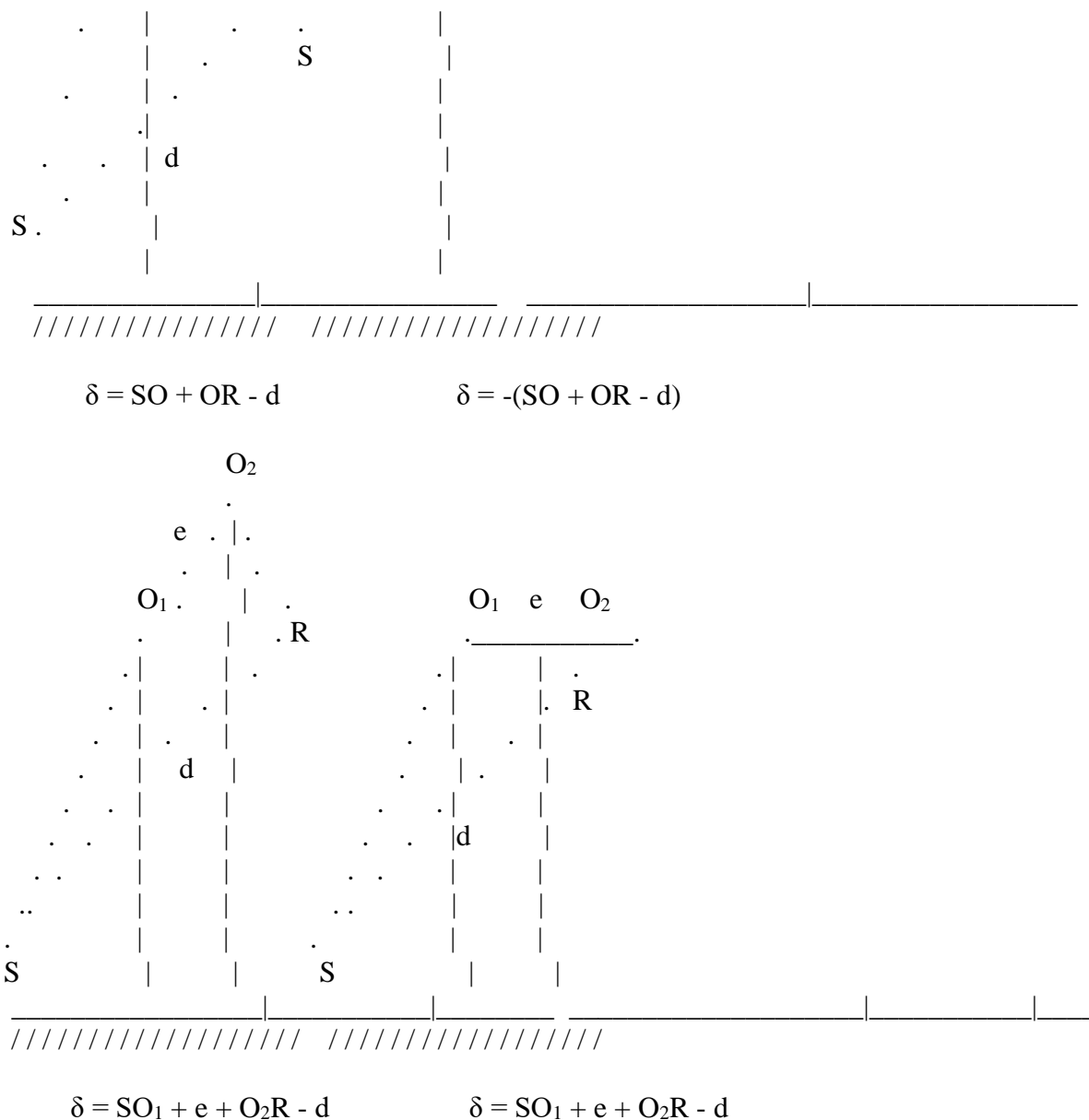
Figura 2.5.d: Calculul diferenței traiectoriei în condiții omogene. O, O1 și O2 sunt punctele de difracție
