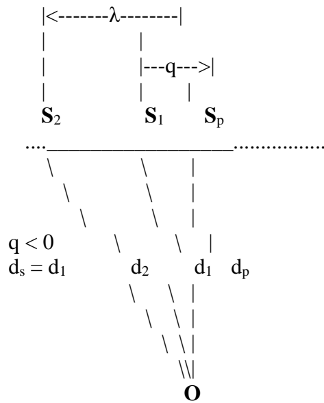
Figura 2.7.j: Geometria segmentului traiectului de zbor pentru poziția observatorului în spatele segmentului
