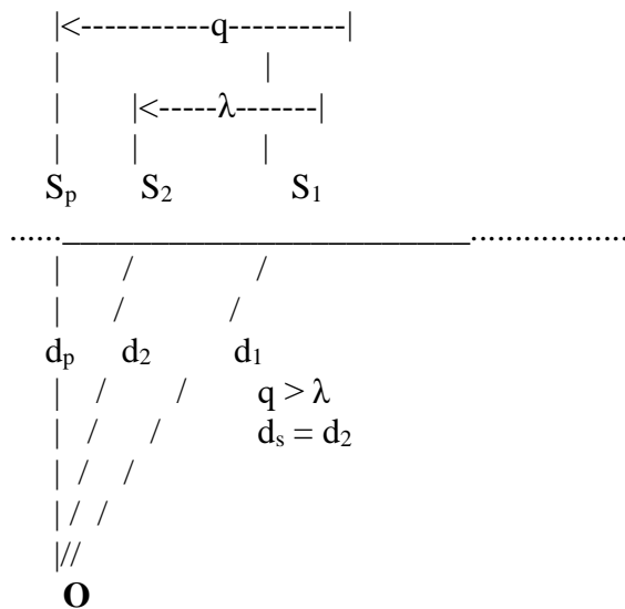
Figura 2.7.l: Geometria segmentului traiectului de zbor pentru poziția observatorului înaintea segmentului
