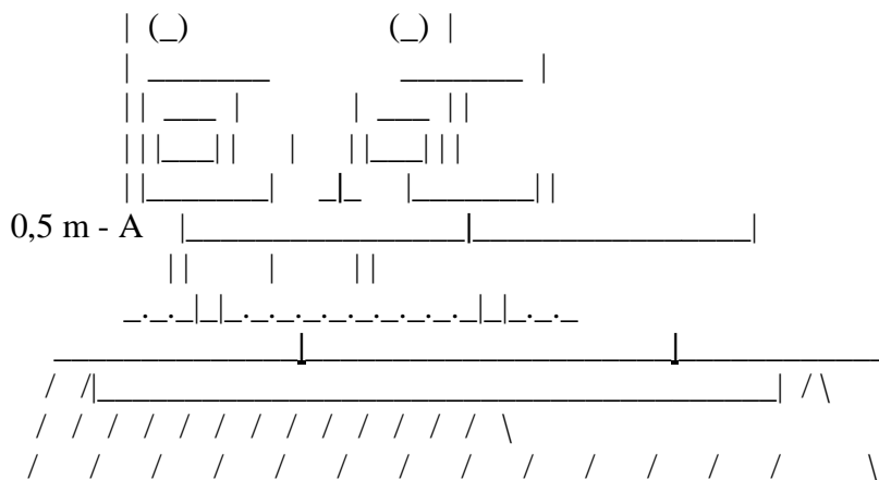
Figura [2.3.a]: Amplasarea surselor de zgomot echivalente
