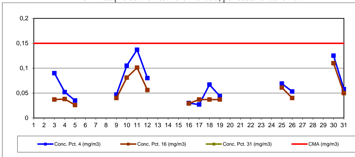
TSP in stațiile de monitorizare manuală, perioada: ianuarie 2017
