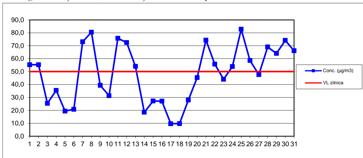
PM10 grav – Stația MM3, concentrații medii zilnice, perioada: ianuarie 2017
