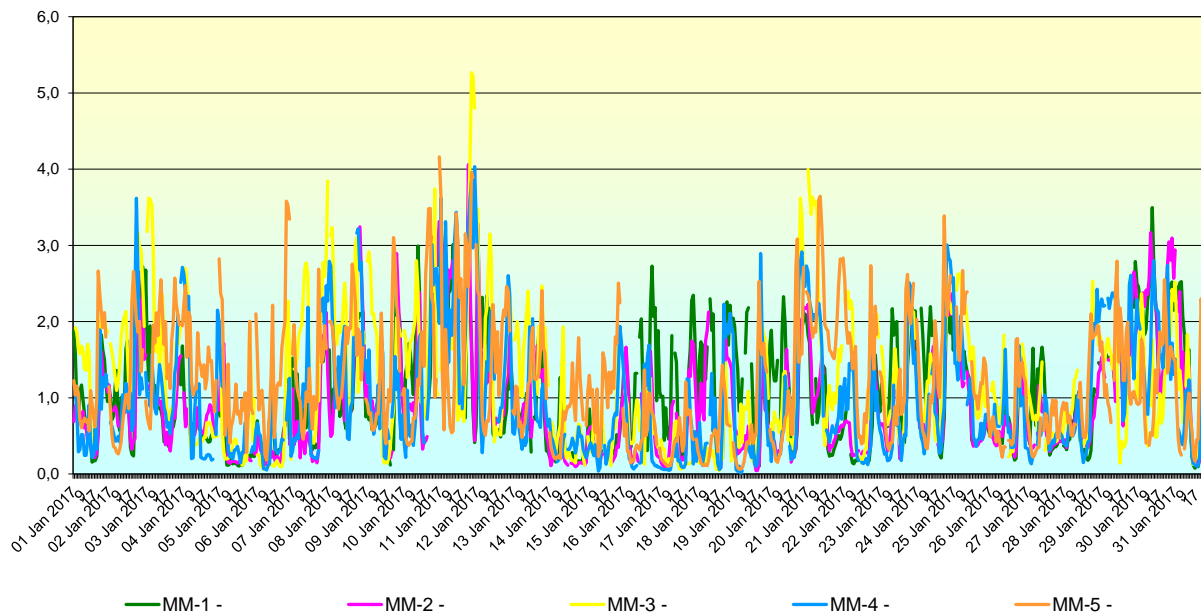
CO (mg/m3), medii orare, perioada: Jan 2017
