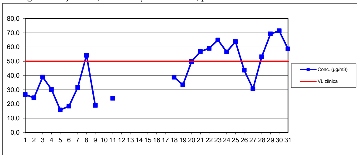
PM10 grav – Stația MM4, concentrații medii zilnice, perioada: ianuarie 2017
