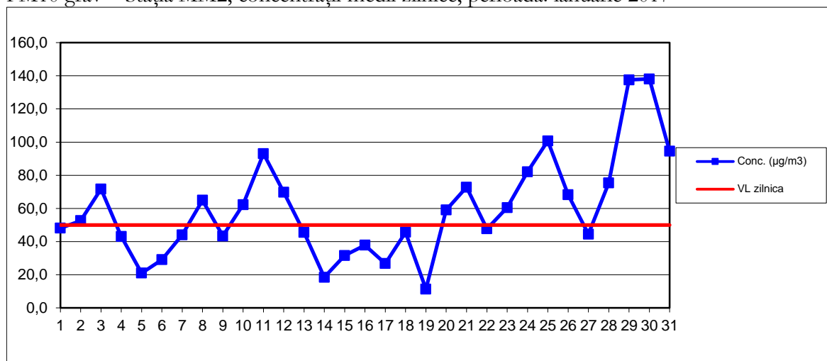
PM10 grav – Stația MM2, concentrații medii zilnice, perioada: ianuarie 2017
