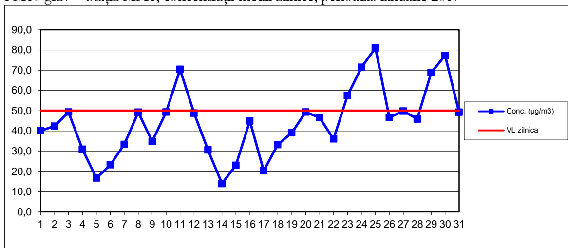
PM10 grav – Stația MM1, concentrații medii zilnice, perioada: ianuarie 2017
