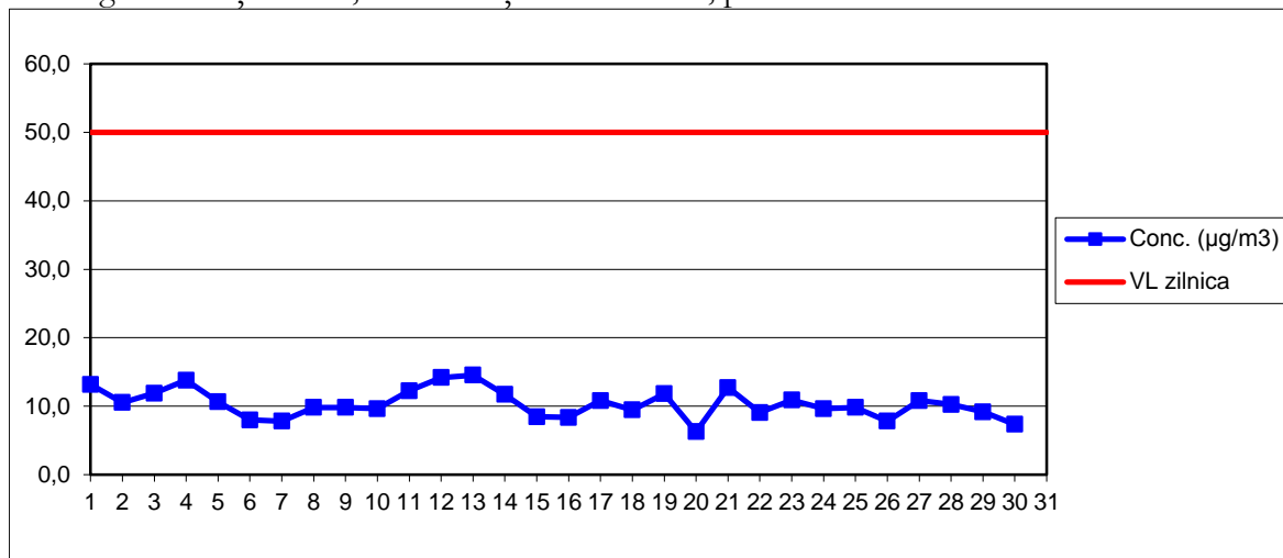
PM10 grav – Stația MM1, concentrații medii zilnice, perioada: iunie 2017
