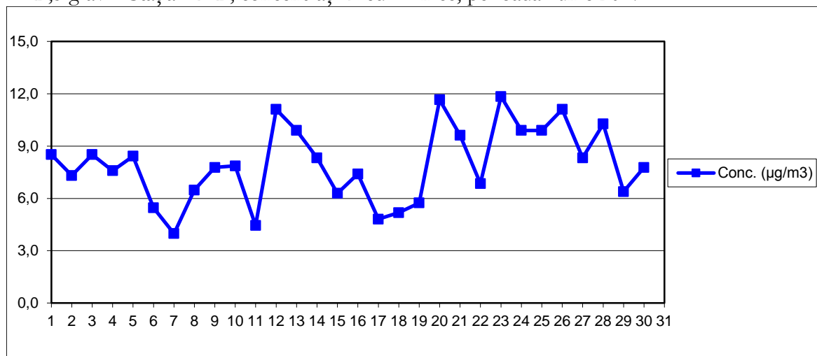
PM2,5 grav – Stația MM2, concentrații medii zilnice, perioada: iunie 2017
