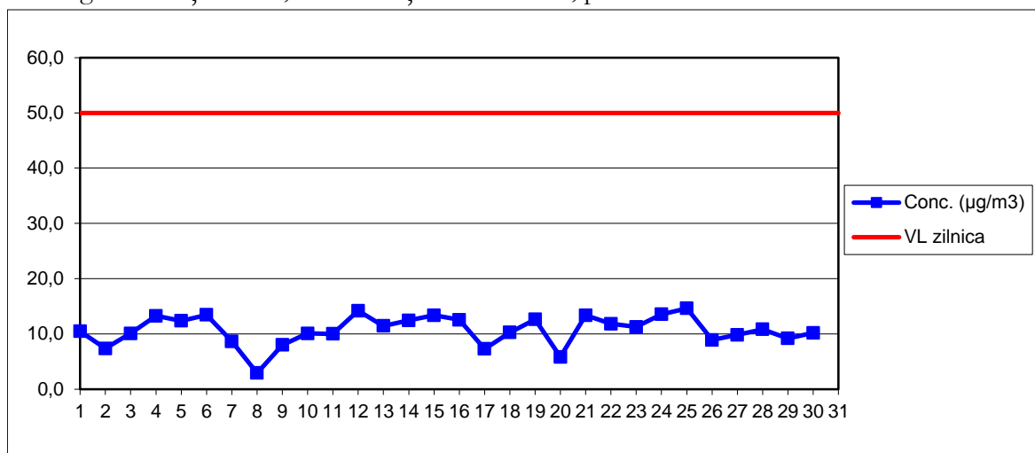
PM10 grav – Stația MM3, concentrații medii zilnice, perioada: iunie 2017
