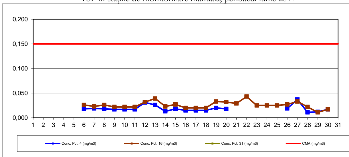
TSP in stațiile de monitorizare manuală, perioada: iunie 2017
