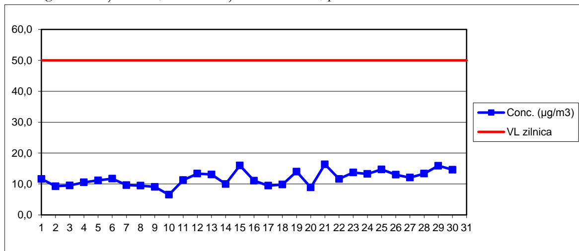
PM10 grav – Stația MM5, concentrații medii zilnice, perioada: iunie 2017
