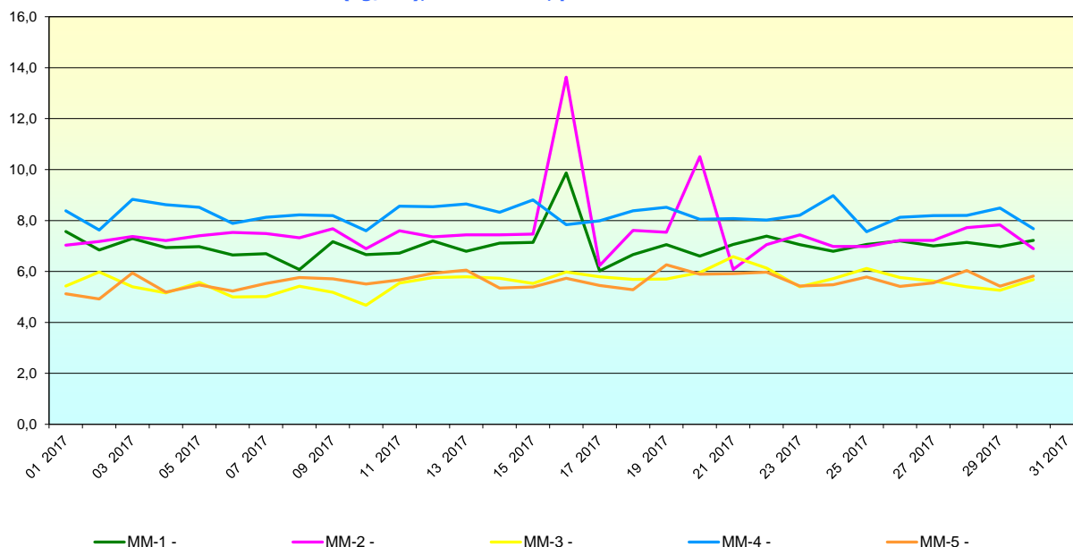
SO2 (ug/m3), medii zilnice, perioada: Iunie 2017
