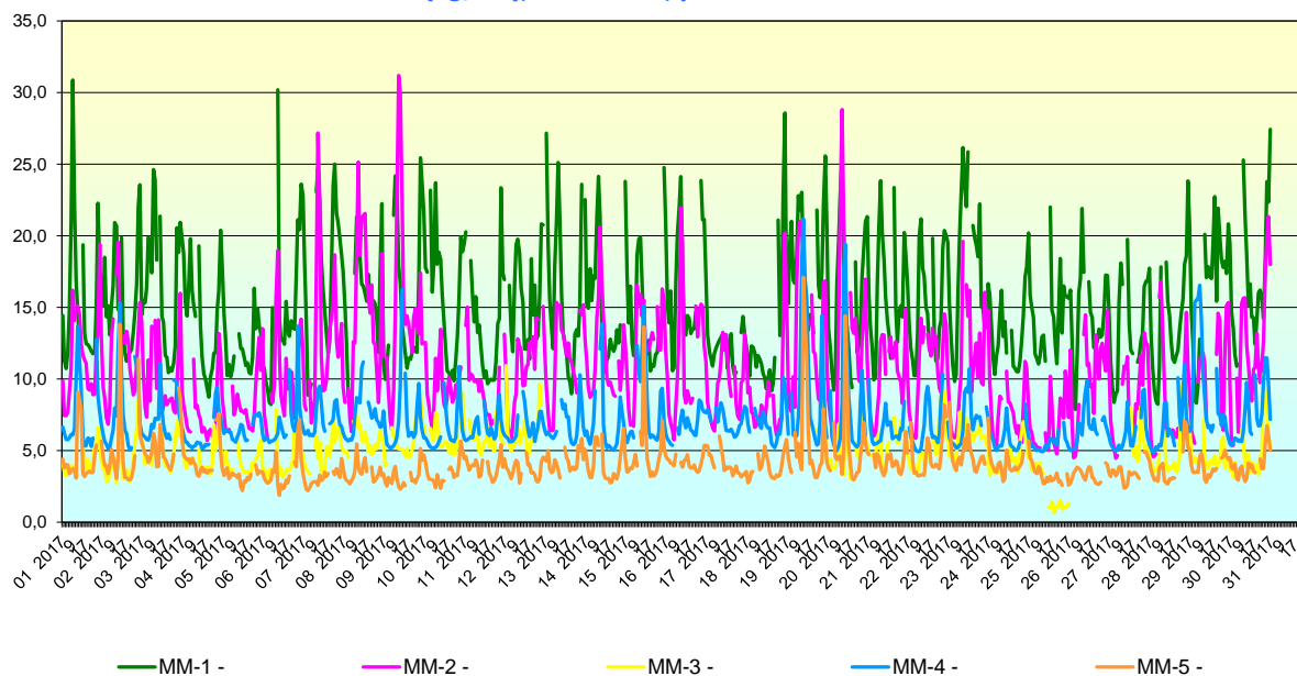
NO2 (ug/m3), medii orare, perioada: Iunie 2017
