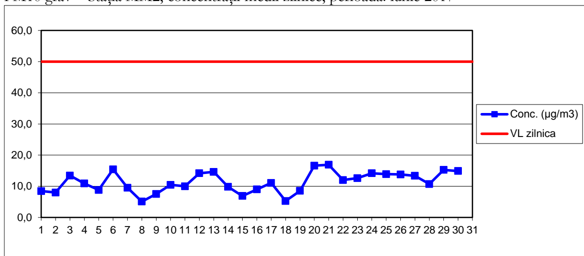
PM10 grav – Stația MM2, concentrații medii zilnice, perioada: iunie 2017
