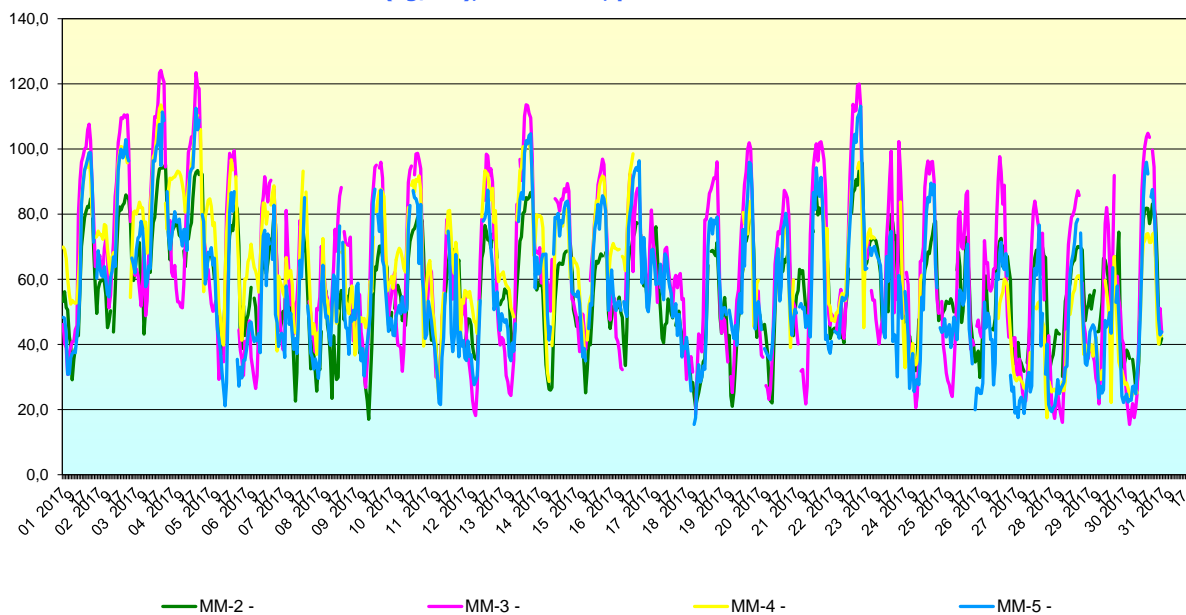
O3 (ug/m3), medii orare, perioada: Iunie 2017
