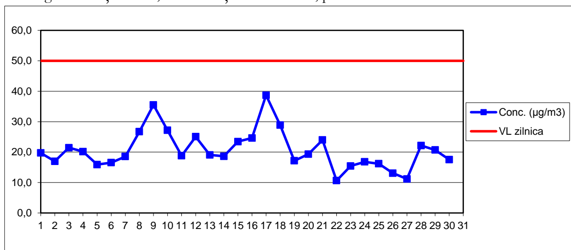
PM10 grav – Stația MM5, concentrații medii zilnice, perioada: noiembrie 2017
