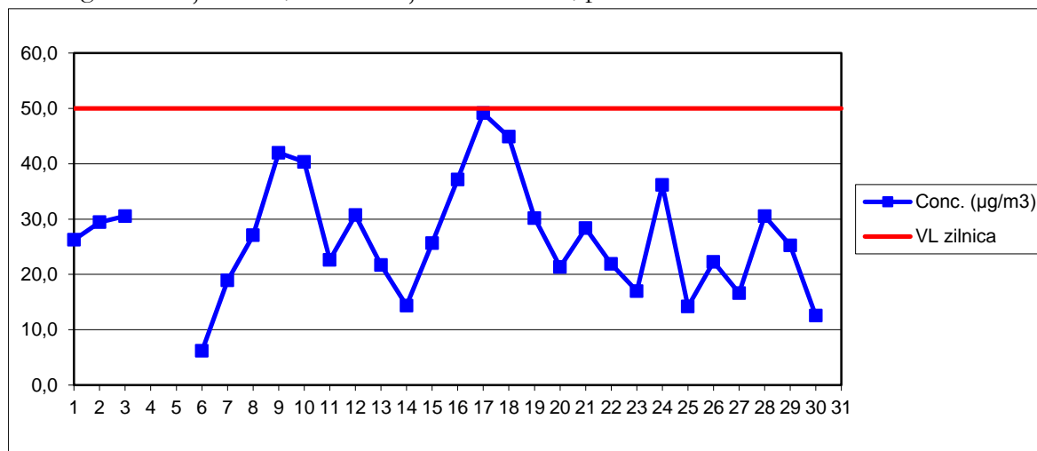
PM10 grav – Stația MM5, concentrații medii zilnice, perioada: noiembrie 2017
