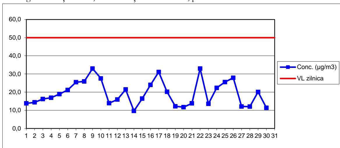
PM10 grav – Stația MM3, concentrații medii zilnice, perioada: noiembrie 2017
