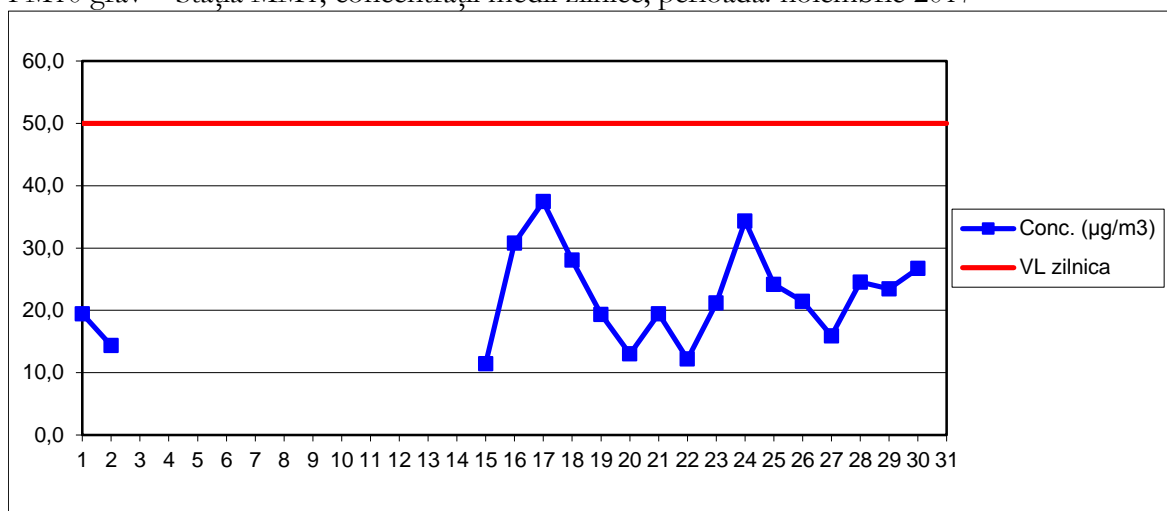
PM10 grav – Stația MM1, concentrații medii zilnice, perioada: noiembrie 2017
