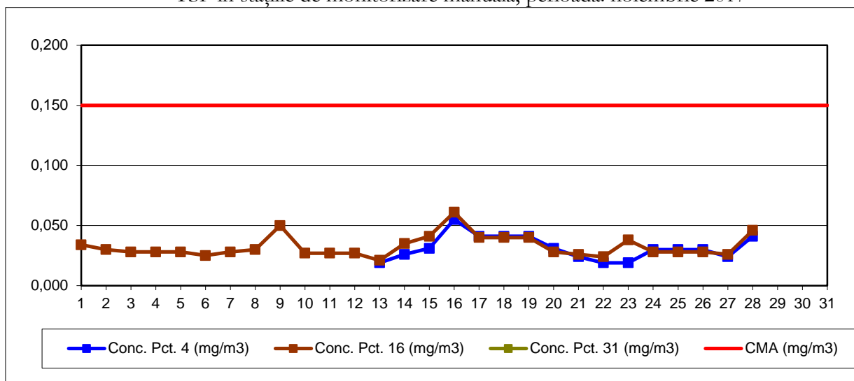
TSP în stațiile de monitorizare manuală, perioada: noiembrie 2017
