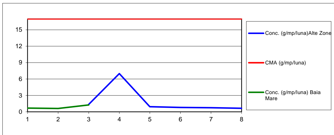
Pulberi sedimentabile - noiembrie 2017
