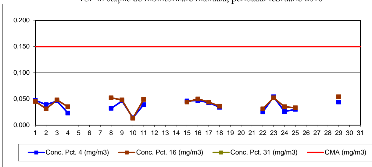
TSP în stațiile de monitorizare manuală, perioada: februarie 2016
