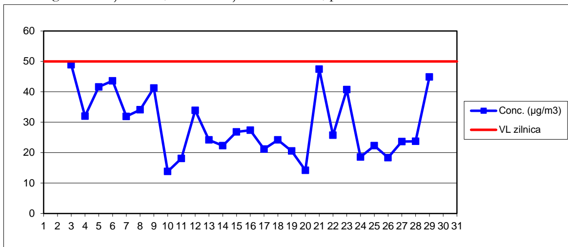
PM10 grav – Stația MM3, concentrații medii zilnice, perioada: februarie 2016
