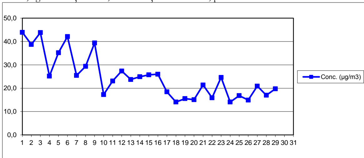
PM2,5 grav – Stația MM2, concentrații medii zilnice, perioada: februarie 2016
