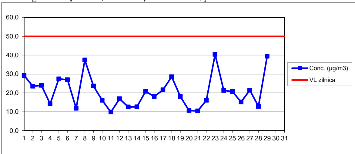
PM10 grav – Stația MM1, concentrații medii zilnice, perioada: februarie 2016
