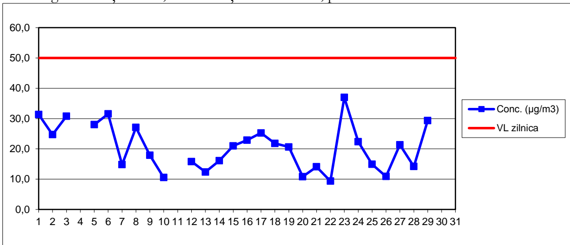
PM10 grav – Stația MM2, concentrații medii zilnice, perioada: februarie 2016
