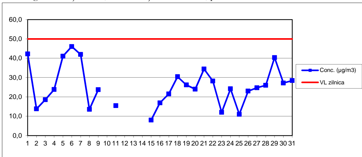
PM10 grav – Stația MM3, concentrații medii zilnice, perioada: martie 2016
