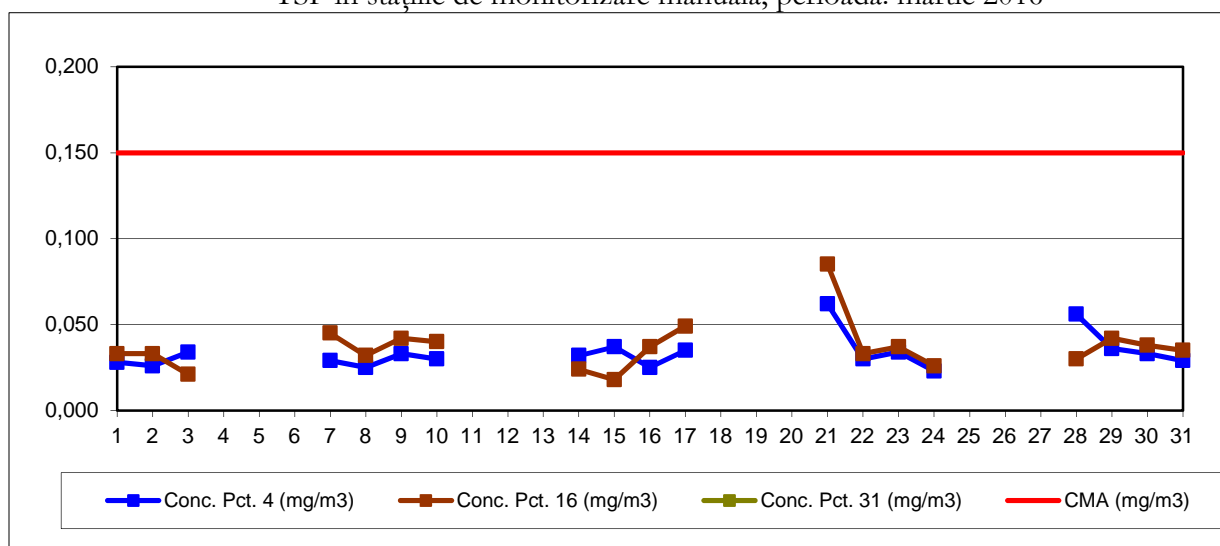
TSP in stațiile de monitorizare manuală, perioada: martie 2016
