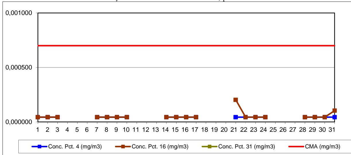
Pb din TSP in stațiile de monitorizare manuală, perioada: martie 2016
