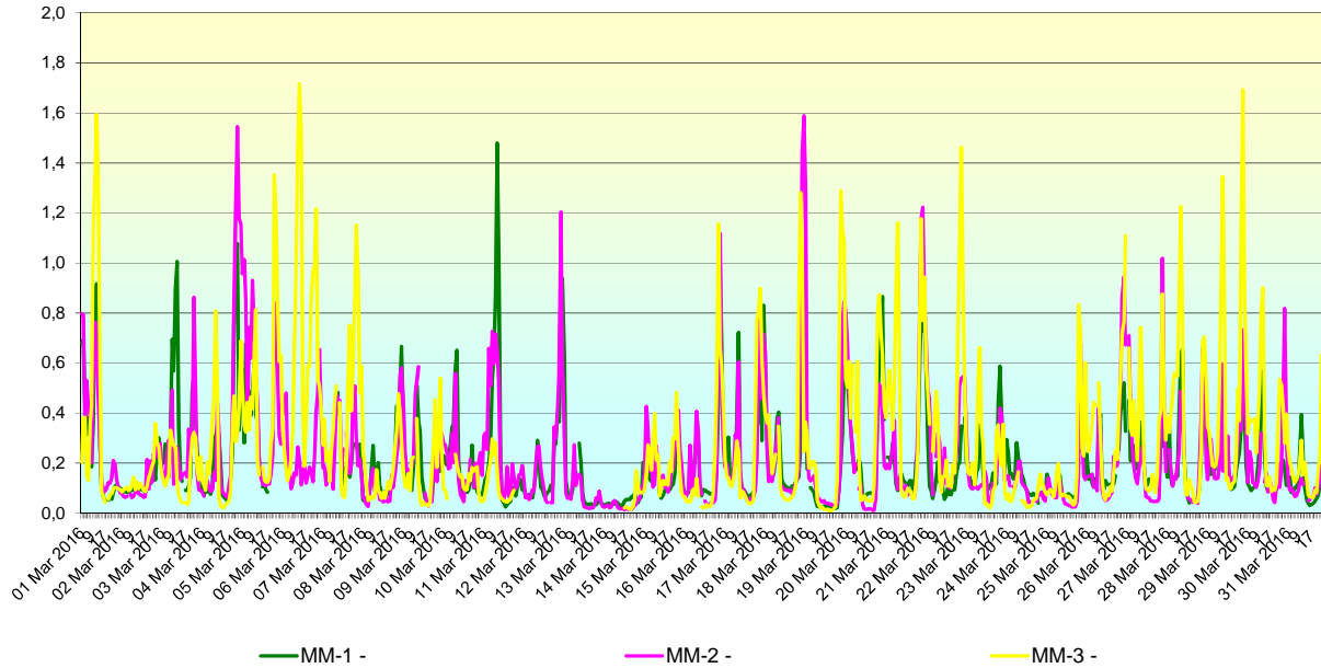
CO (mg/m3), medii orare, perioada: Mar 2016
