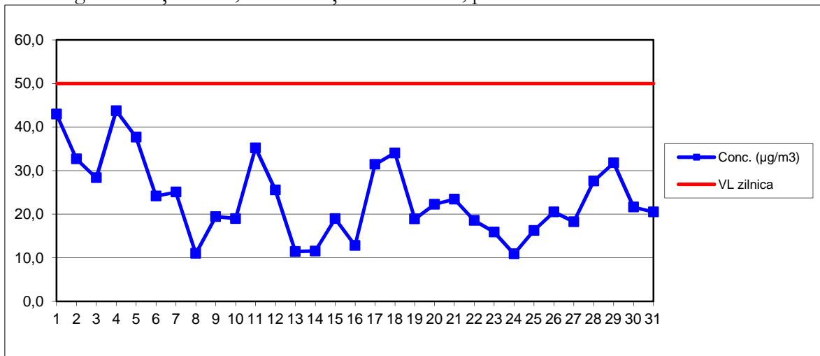
PM10 grav – Stația MM1, concentrații medii zilnice, perioada: martie 2016
