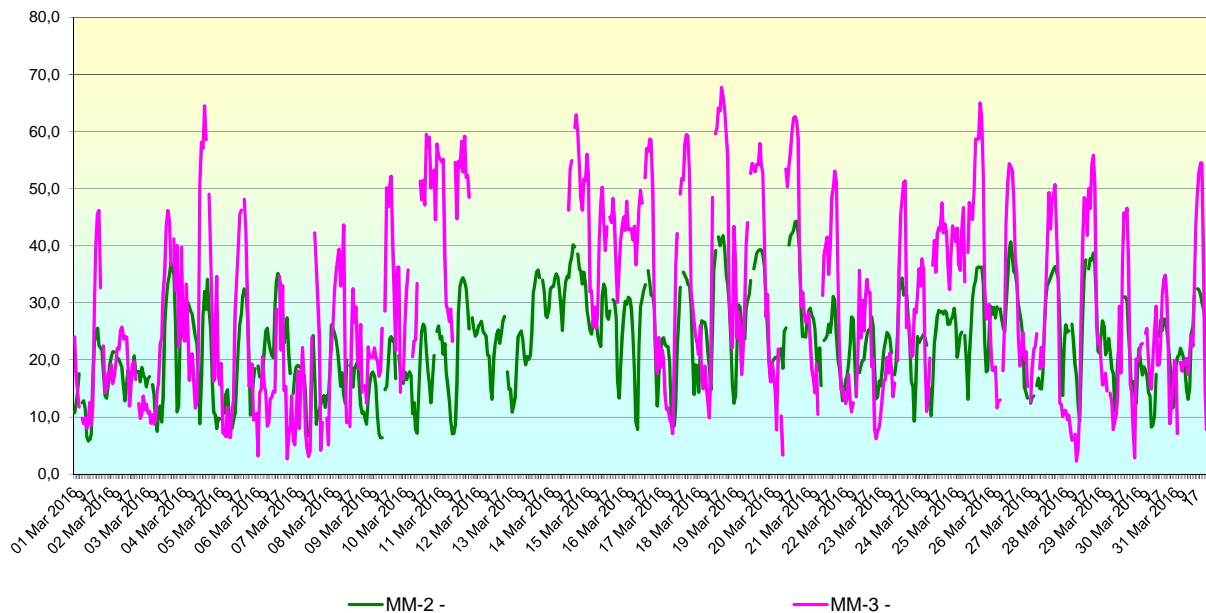
O3 ( \mu\text{g}/\text{m}^3 ), medii orare, perioada: Mar 2016
