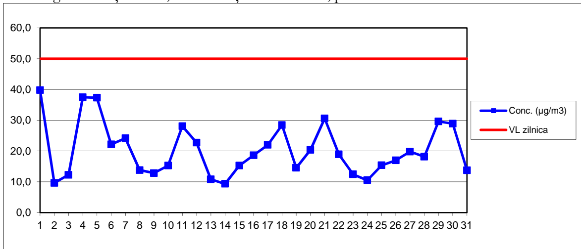
PM10 grav – Stația MM2, concentrații medii zilnice, perioada: martie 2016
