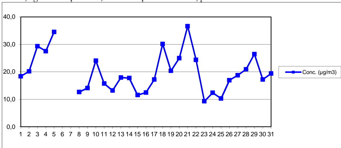
PM2,5 grav – Stația MM2, concentrații medii zilnice, perioada: martie 2016
