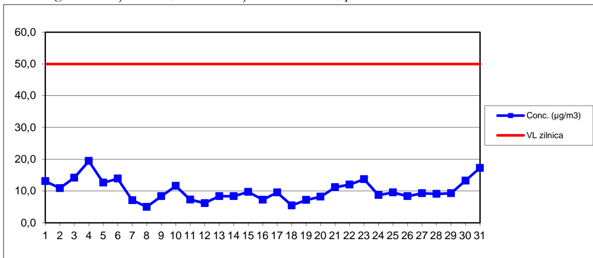
PM10 grav – Stația MM3, concentrații medii zilnice, perioada: mai 2016
