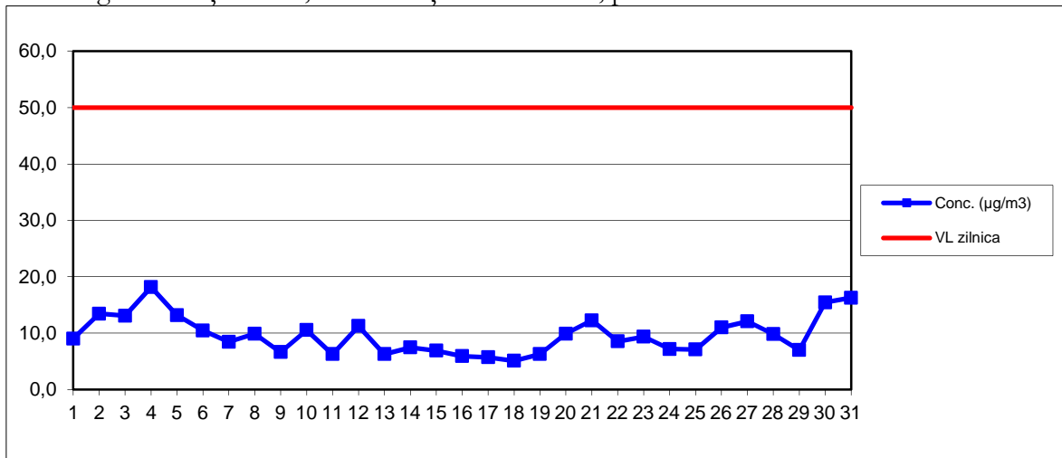
PM10 grav – Stația MM1, concentrații medii zilnice, perioada: mai 2016
