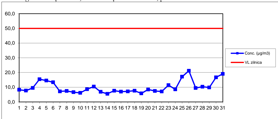
PM10 grav – Stația MM2, concentrații medii zilnice, perioada: mai 2016
