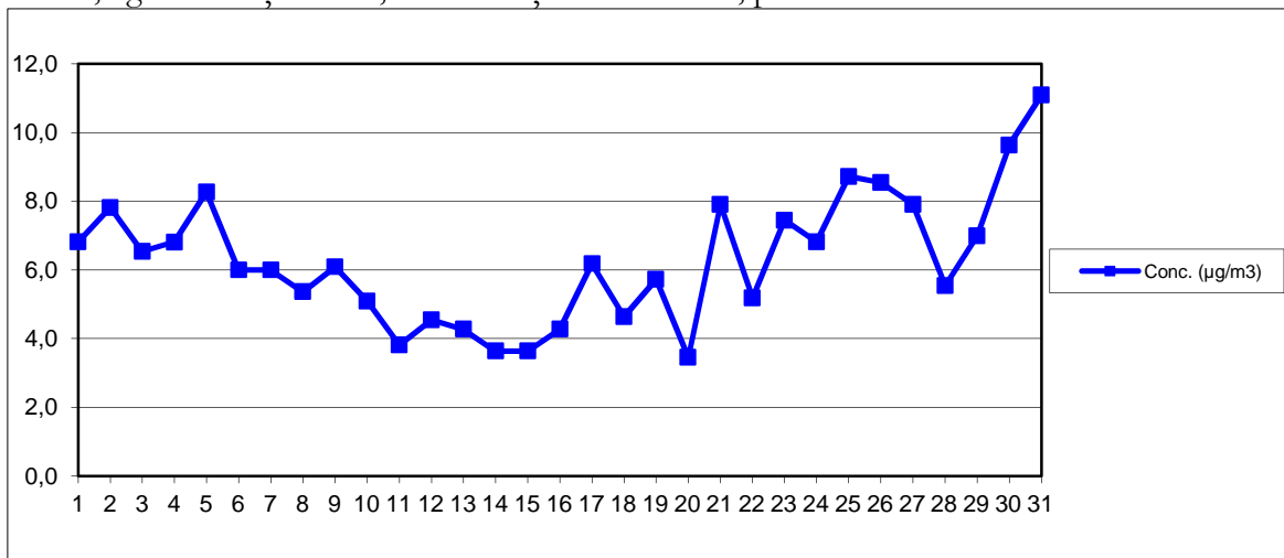
PM2,5 grav – Stația MM2, concentrații medii zilnice, perioada: mai 2016
