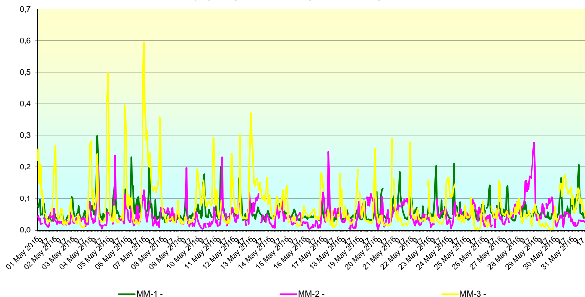
CO (mg/m3), medii orare, perioada: May 2016
