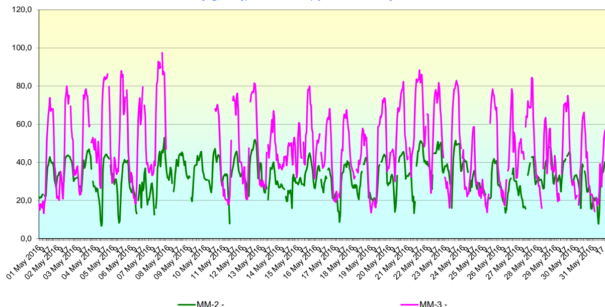
O3 (ug/m3), medii orare, perioada: May 2016
