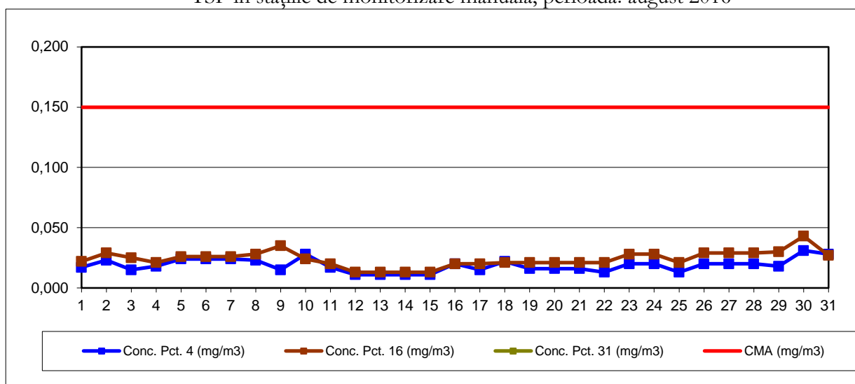
TSP in stațiile de monitorizare manuală, perioada: august 2016
