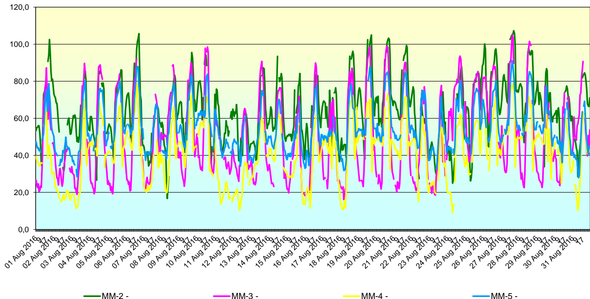
O3 ( \mu\text{g}/\text{m}^3 ), medii orare, perioada: Aug 2016
