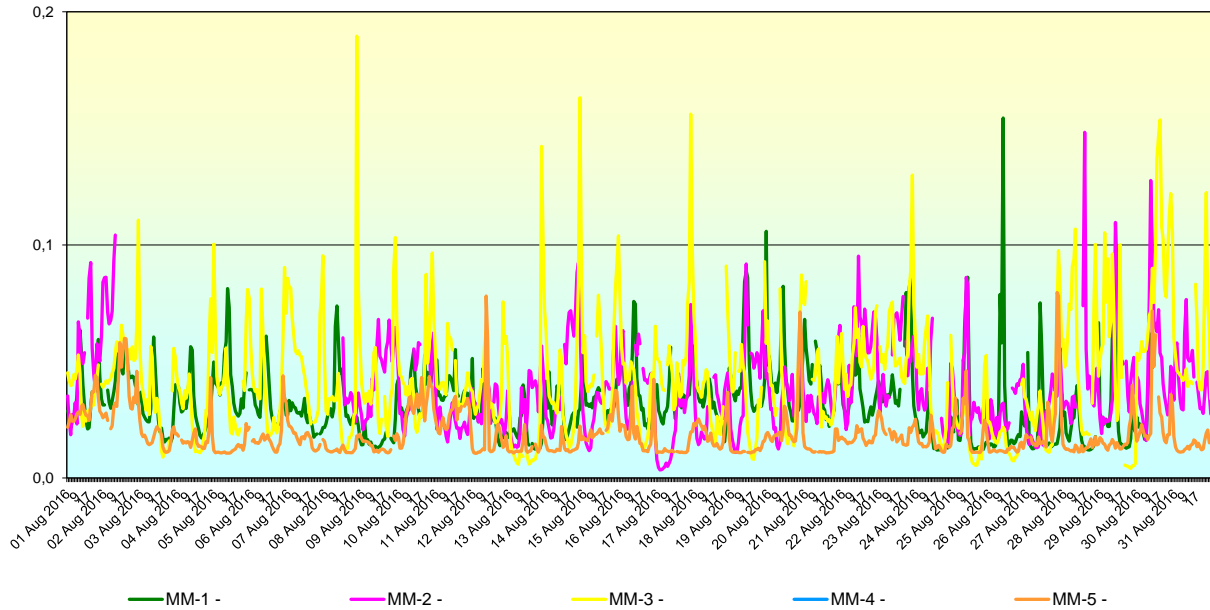
CO (mg/m3), medii orare, perioada: Aug 2016
