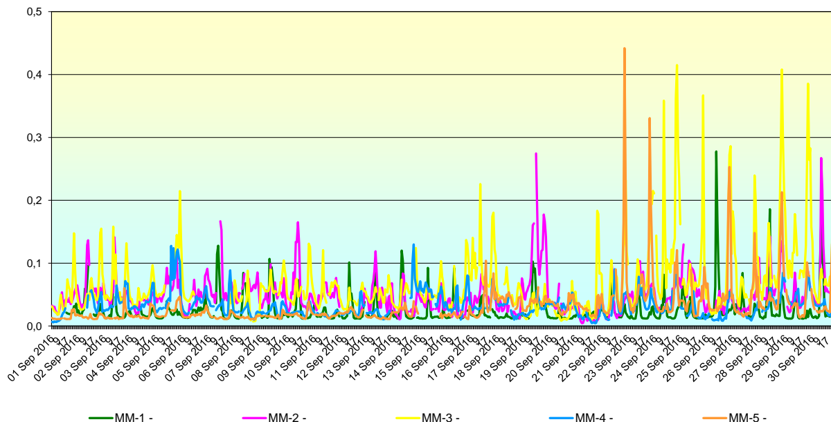
CO (mg/m3), medii orare, perioada: Sep 2016
