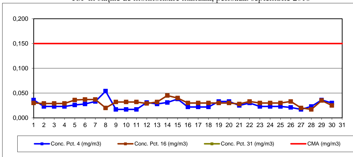
TSP în stațiile de monitorizare manuală, perioada: septembrie 2016
