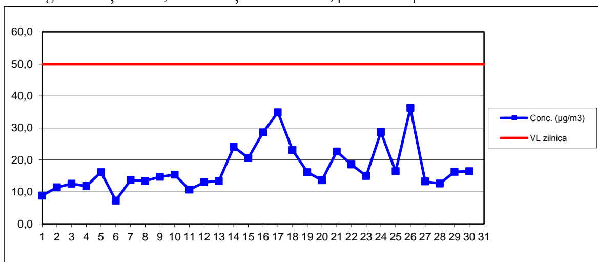
PM10 grav – Stația MM5, concentrații medii zilnice, perioada: septembrie 2016
