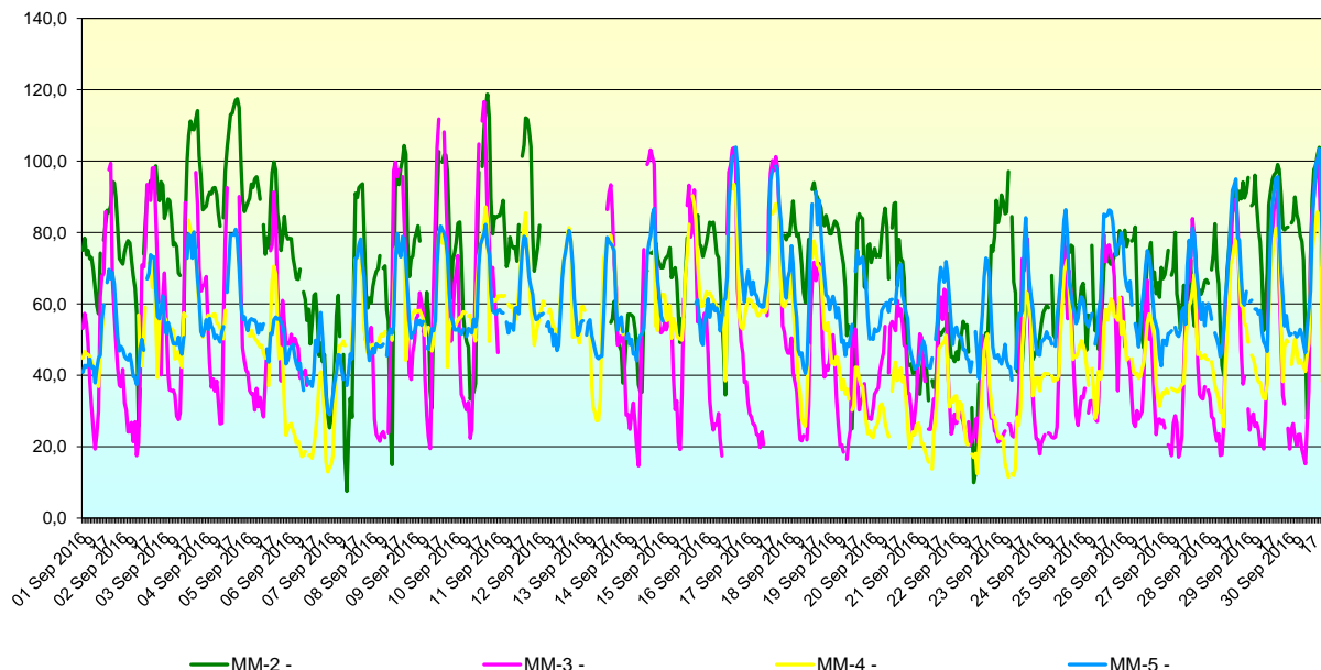
O3 ( \mu\text{g}/\text{m}^3 ), medii orare, perioada: Sep 2016
