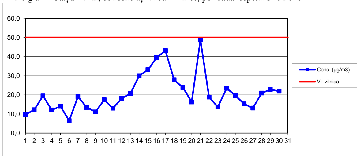
PM10 grav – Stația MM2, concentrații medii zilnice, perioada: septembrie 2016
