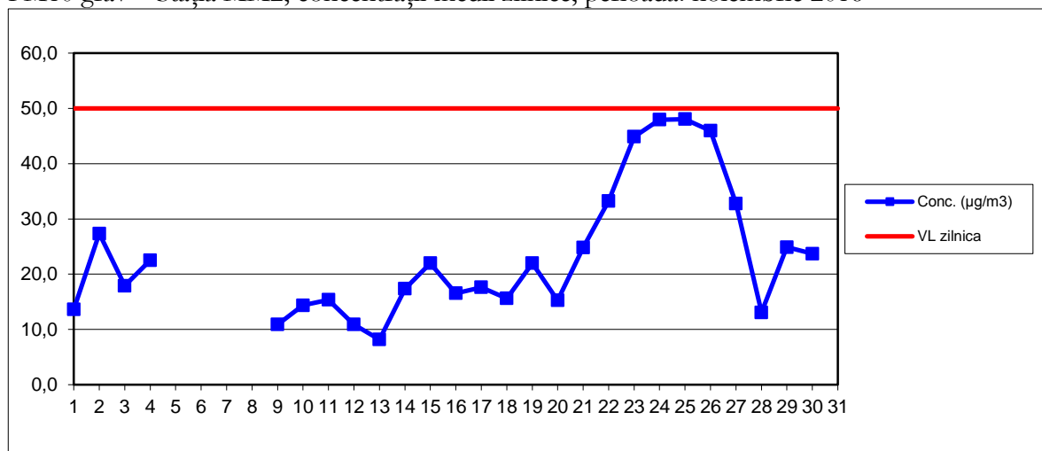
PM10 grav – Stația MM2, concentrații medii zilnice, perioada: noiembrie 2016
