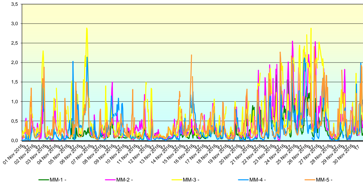
CO (mg/m3), medii orare, perioada: Nov 2016
