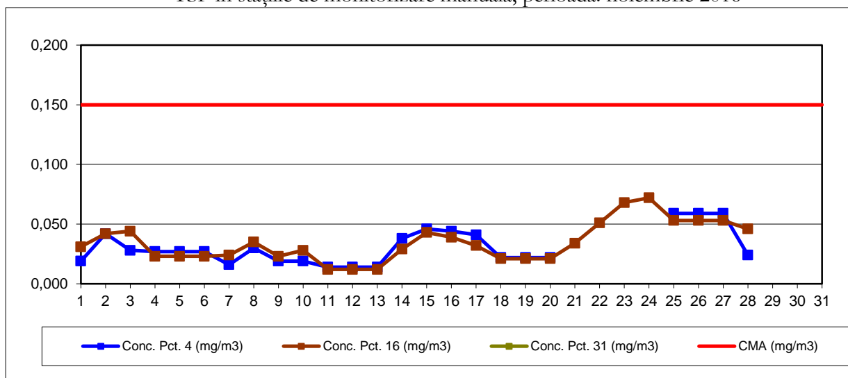
TSP în stațiile de monitorizare manuală, perioada: noiembrie 2016
