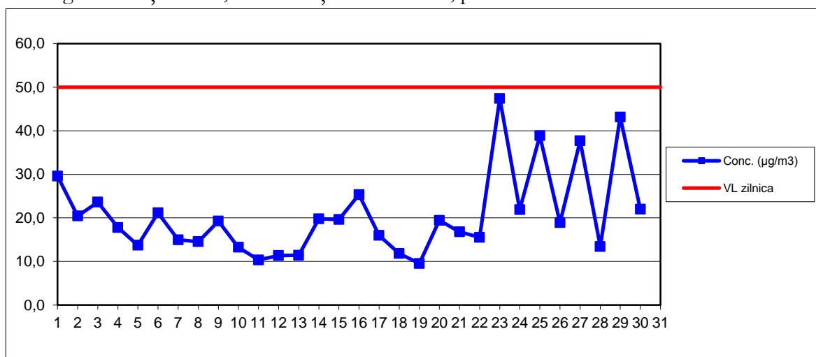
PM10 grav – Stația MM5, concentrații medii zilnice, perioada: noiembrie 2016
