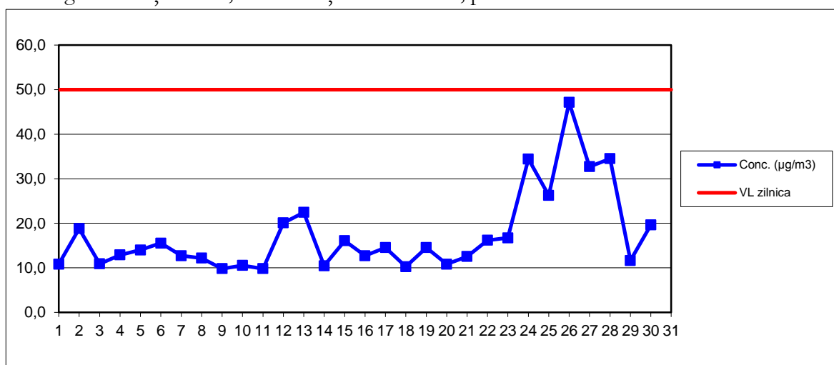
PM10 grav – Stația MM4, concentrații medii zilnice, perioada: noiembrie 2016
