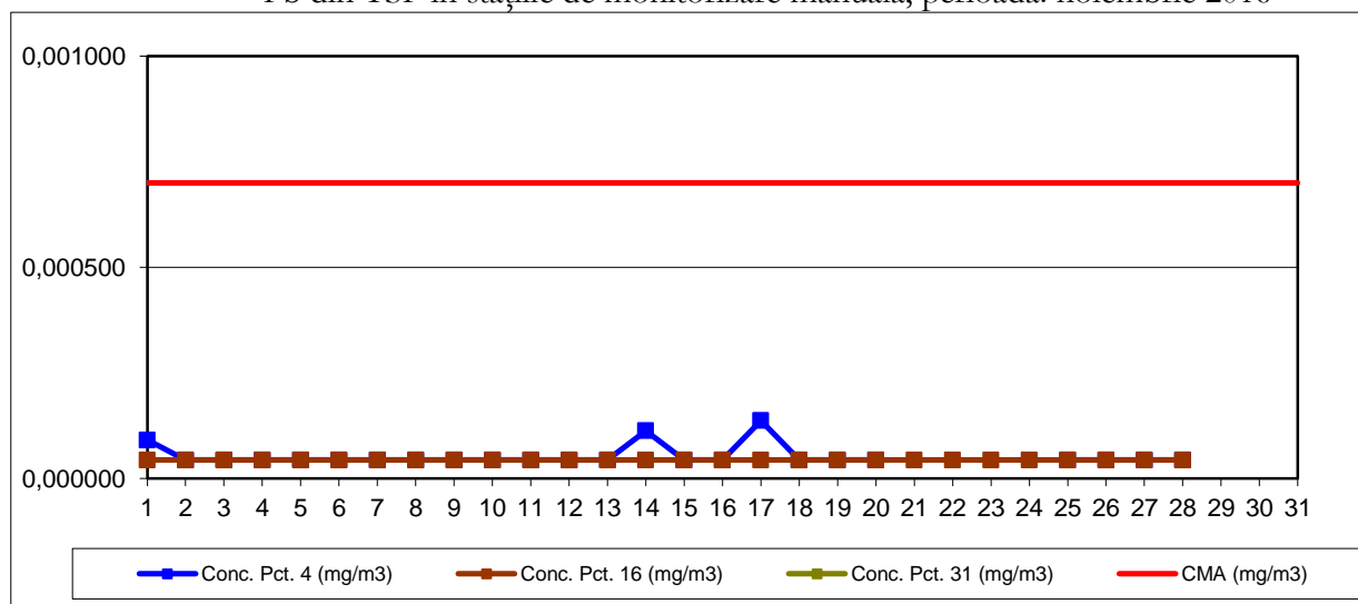
Pb din TSP in stațiile de monitorizare manuală, perioada: noiembrie 2016
