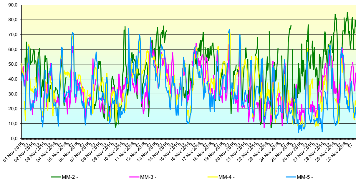
O3 (ug/m3), medii orare, perioada: Nov 2016
