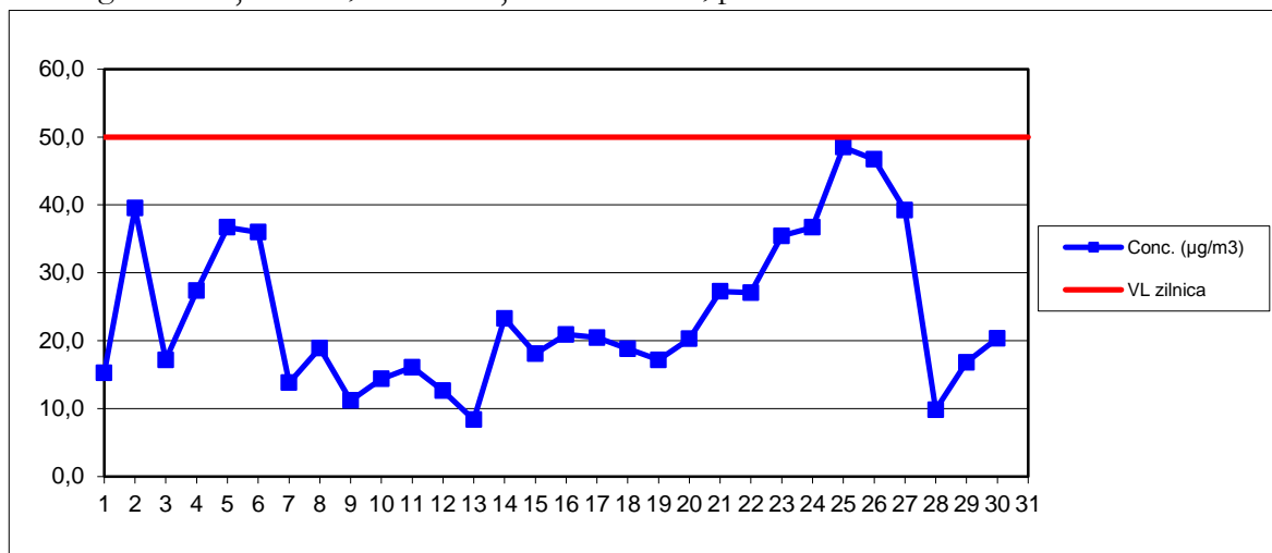
PM10 grav – Stația MM3, concentrații medii zilnice, perioada: noiembrie 2016
