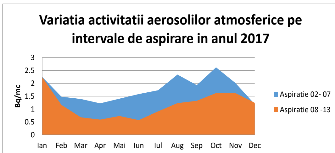
Figura IX.1.1.2.1. Variația medie anuală a activității Beta globală imediată a aerosolilor atmosferici în funcție de variația diurnă
