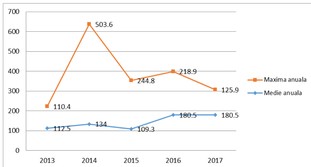
Figura IX.1.3.5. Variația mediilor și maximelor anuale ale activității beta globale a râului Tisa
