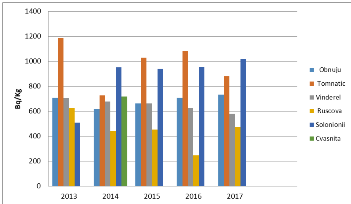
Figura IX.2.4.3. Nivelul activității K - 40 în sol necultivat din zona Repedea și Poienile de sub Munte în perioada 2012 - 2017
