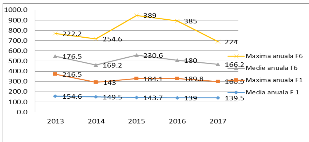
Figura IX.1.3.7. Variația mediilor și maximelor anuale ale activității beta globale a forajelor F 6 Sat Săsar și F 1 Sat Hideaga
