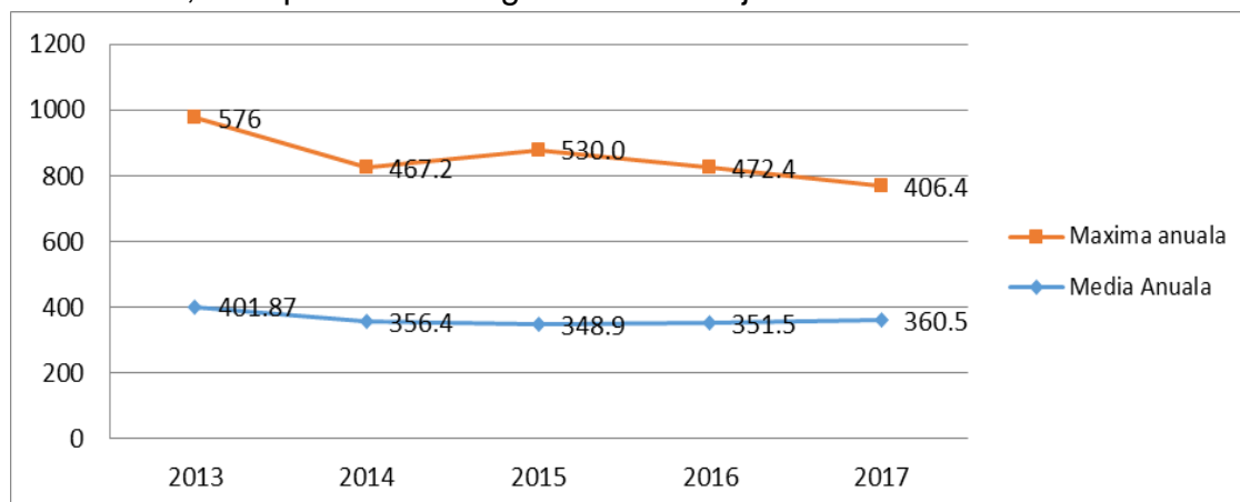
Figura IX.1.4.1. Activitatea specifică \beta -globală pentru sol necultivat din Baia Mare
