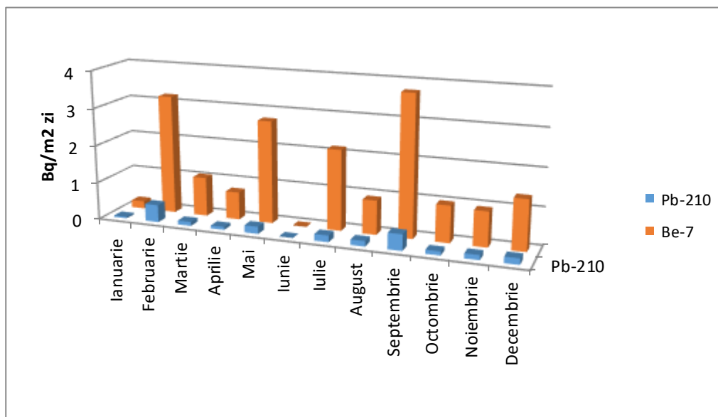
Figura IX.1.2.2. Variația activității specifice lunare a radionuclizilor naturali identificați în probele de depuneri atmosferice totale
