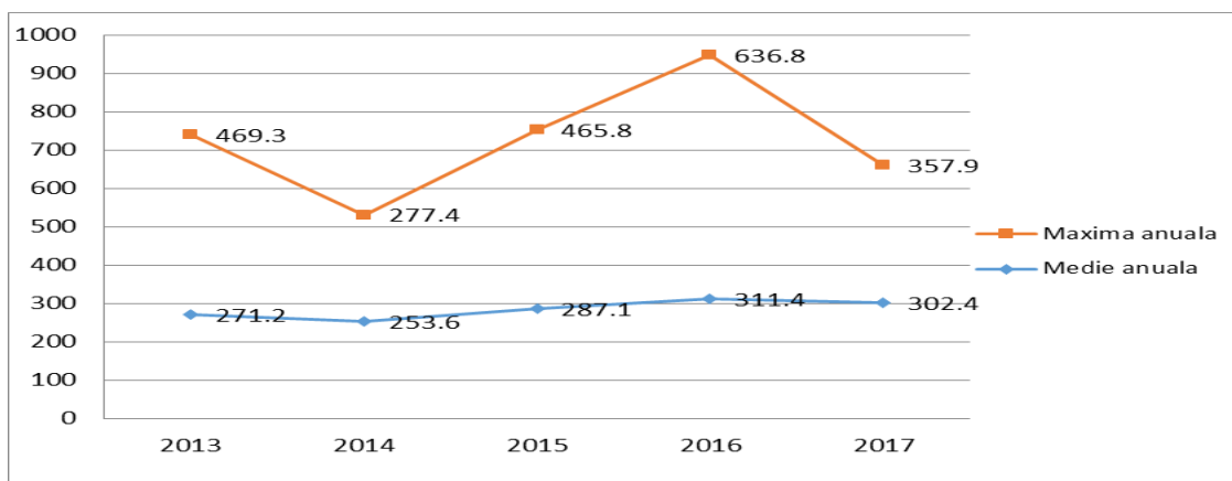
Figura IX.1.5.1. Activitatea specifică \beta -globală pentru vegetație spontană
