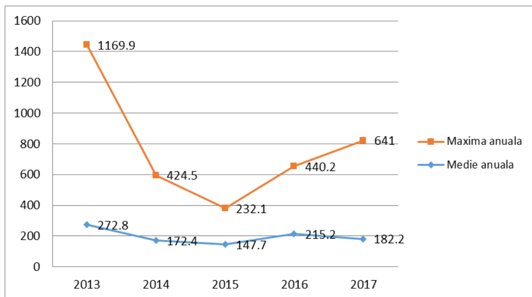
Figura IX.1.3.3. Variația mediilor și maximelor anuale ale activității beta globale a râului Someș
