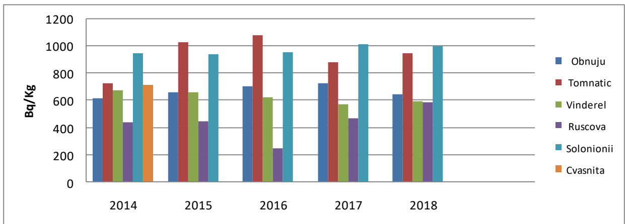
Figura IX.2.4.3. Nivelul activității K - 40 în sol necultivat din zona Repedeș și Poienile de sub Munte în perioada 2014 - 2018
