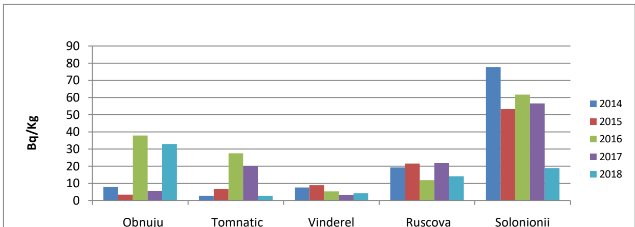
Figura IX.2.4.4. Nivelul activității Cs-137 în sol necultivat din zona Repedeș și Poienile de sub Munte în perioada 2014 - 2018
