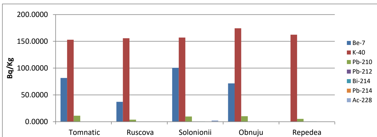
Figura IX.2.5.3. Nivelul activității radionuclizilor indentificati în vegetație spontană din zona Repedea și Poienile de sub Munte în anul 2018
