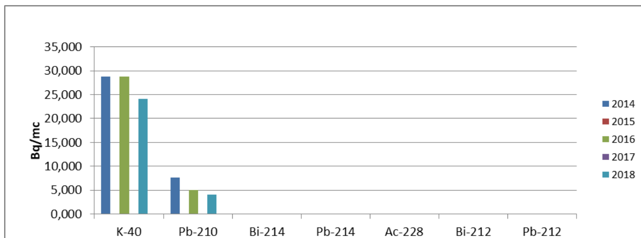
Figura IX.1.2.10. Evoluția activității celor mai frecvenți radionuclizi identificați pentru Baraj Firiza în perioada 2014 – 2018
