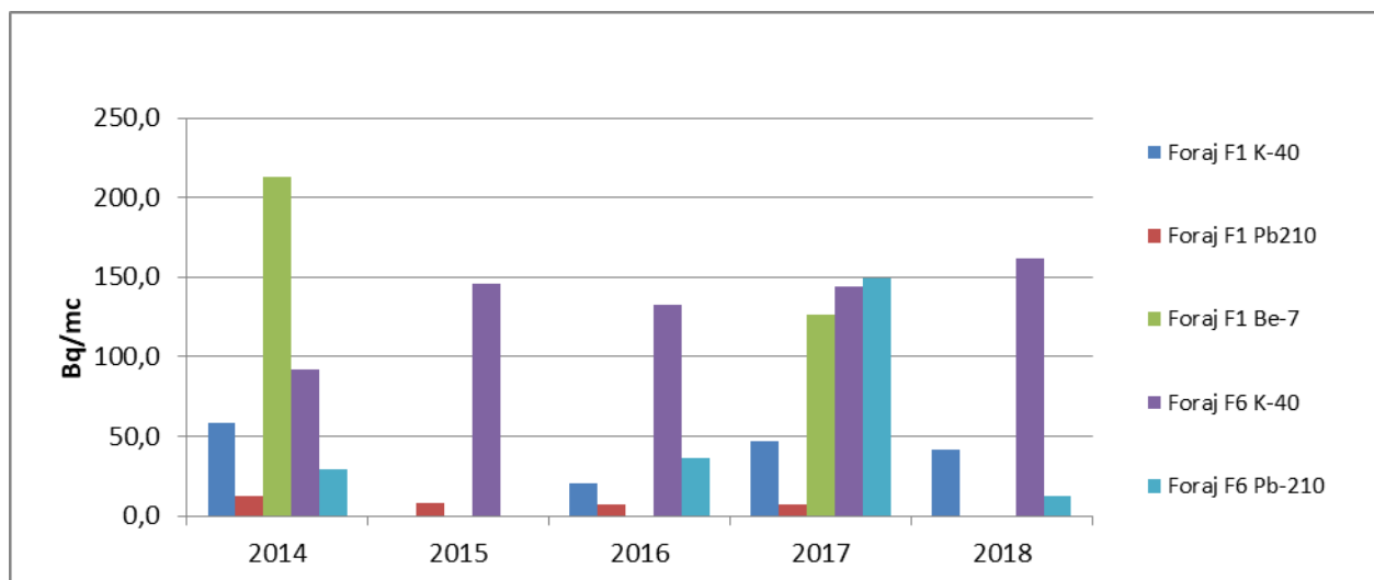
Figura IX.1.2.8. Evoluția activității celor mai frecvenți radionuclizi identificați pentru cele două foraje în perioada 2014 - 2018
