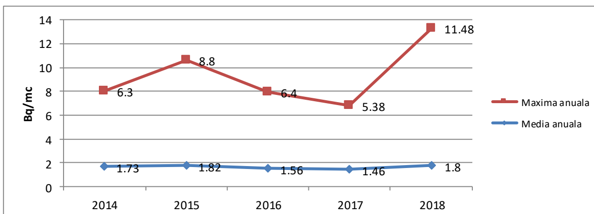
Figura IX.1.1.2.2. Variația mediilor și maximelor anuale ale activității Beta globale imediată a aerosolilor atmosferici
