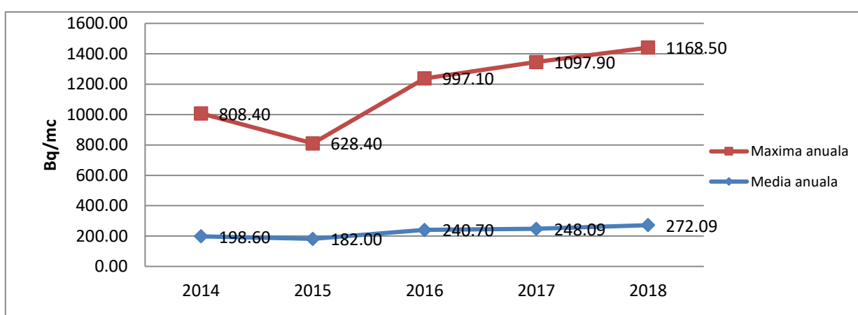
Figura IX.1.2.1. Variația mediilor și maximelor anuale ale activității beta globale a râului Săsar
