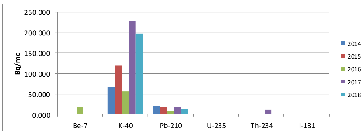
Figura IX.1.2.4. Evoluția activității celor mai frecvenți radionuclizi identificați pentru râul Someș în perioada 2014 - 2018
