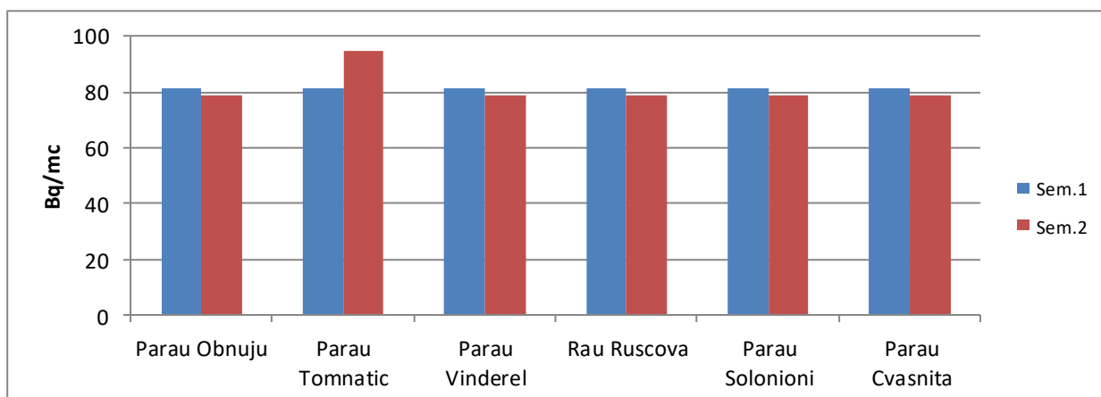
Figura IX.2.1.2. Măsurători \beta - globale pentru apa de suprafață în zona Repedea și Poienile de sub Munte în anul 2018
