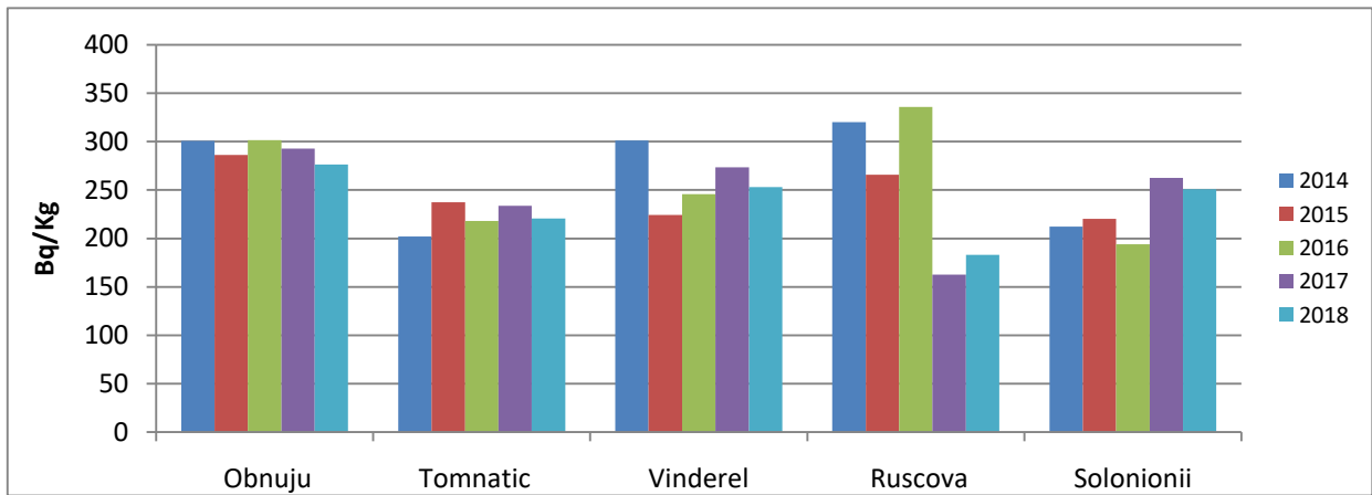
Figura IX.2.5.1. Activități \beta -globale în vegetație spontană din zona Repedea și Poienile de sub Munte în perioada 2014 – 2018
