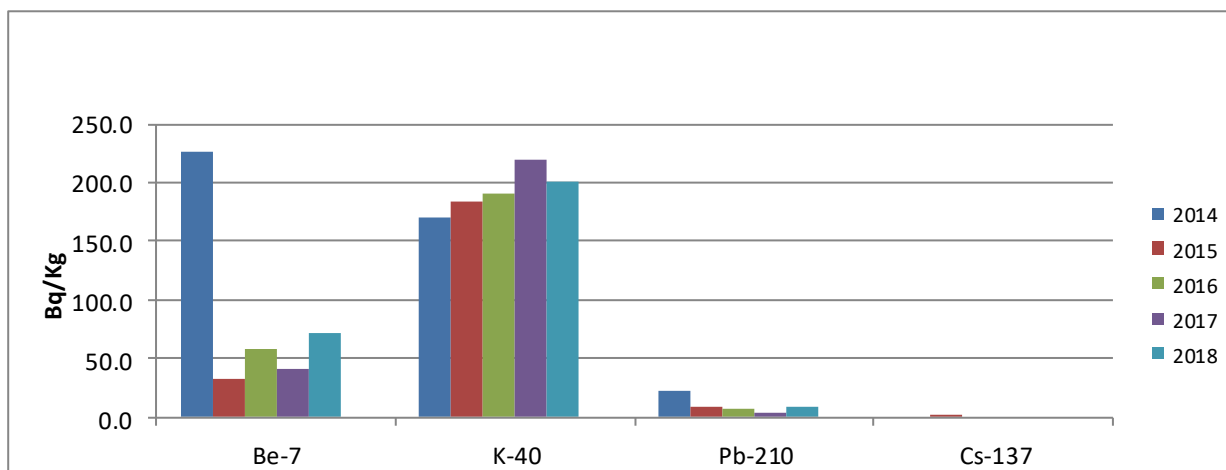
Figura IX.1.4.2. Evoluția activității celor mai frecvenți radionuclizi identificați pentru vegetația spontană
