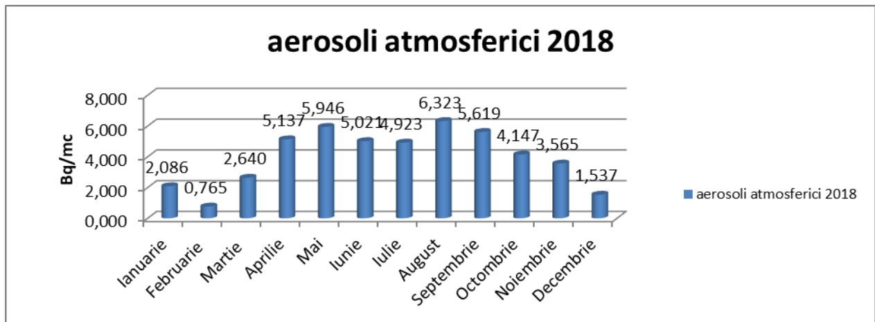
Figura IX.1.1.2.6. Variația activității lunare a radionuclidului Be-7 în probe de aerosoli atmosferici
