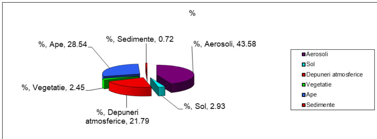
Figura IX.1.1. Structura prelevărilor de probe în anul 2018
