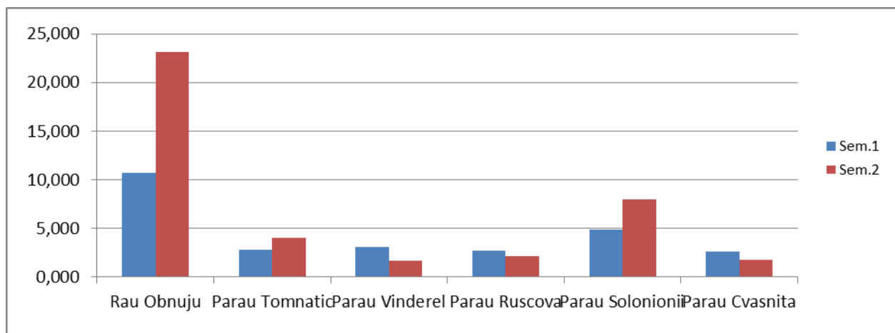
Figura IX.2.3.2. Nivelul activității Cs-137 în sedimente din zona Repedeș și Poienile de sub Munte în anul 2018
