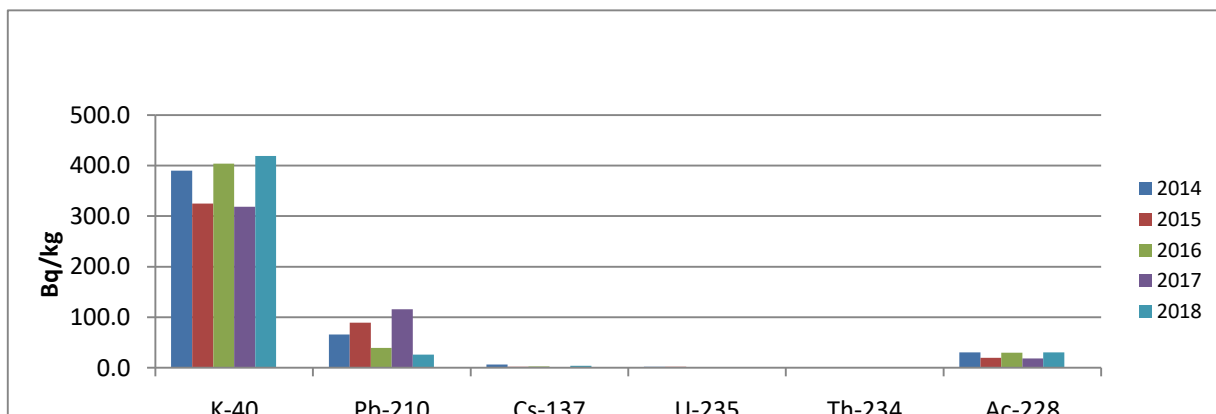
Figura IX.1.3.2. Evoluția activității celor mai frecvenți radionuclizi identificați pentru solul necultivat din Baia Mare
