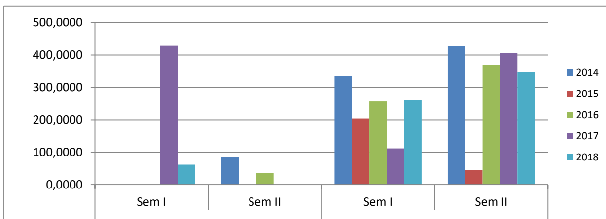
Figura IX.2.2.2. Nivelul activității K-40 în apa din fântâni, în zona Repedeș și Poienile de sub Munte în anul 2014 – 2018
