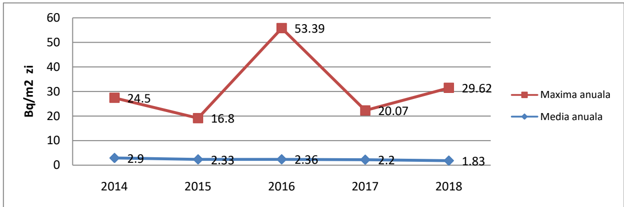
Figura IX.1.2.1. Variația mediilor și maximelor anuale ale activității beta Globale a depunerilor atmosferice totale
