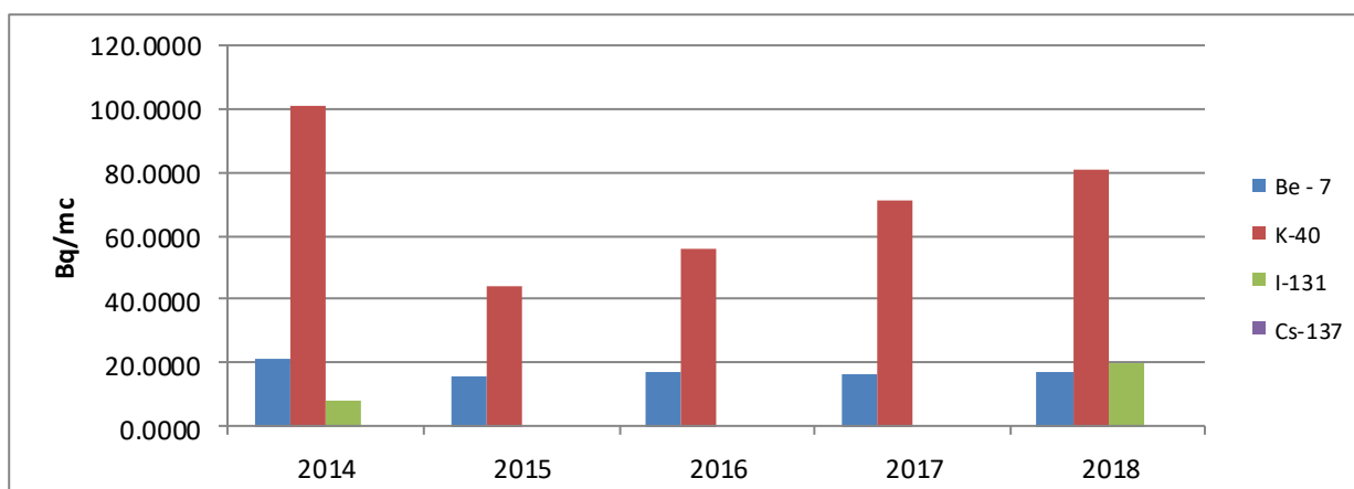
Figura IX.1.2.2. Evoluția activității celor mai frecvenți radionuclizi identificați pentru râul Săsar în perioada 2014 – 2018
