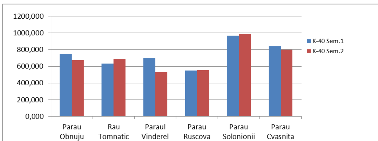
Figura IX.2.3.1. Nivelul activității K-40 în sedimente din zona Repedeș și Poienile de sub Munte în anul 2018
