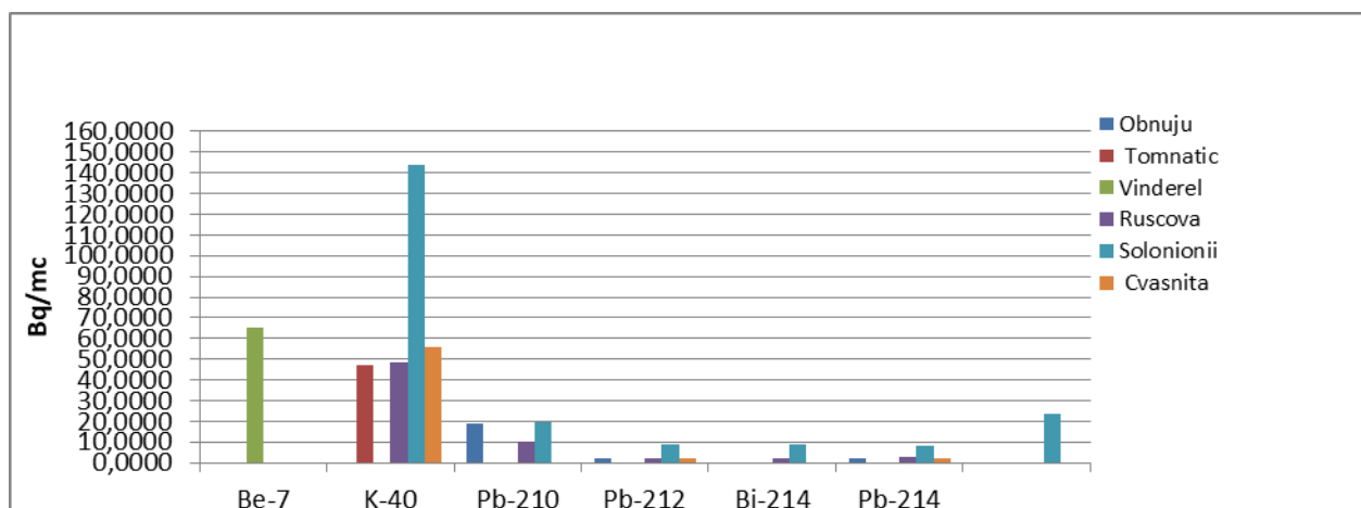
Figura IX.2.1.3. Nivelul activităților radionuclizilor identificați în apa de suprafață din zona Repedeș și Poienile de sub Munte în anul 2018
