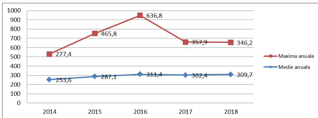
Figura IX.1.4.1. Activitatea specifică \beta -globală pentru vegetație spontană
