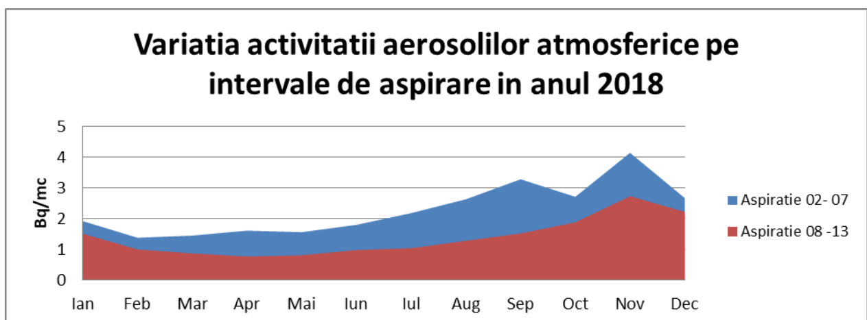
Figura IX.1.1.2.1. Variația medie anuală a activității Beta globală imediată a aerosolilor atmosferici în funcție de variația diurnă
