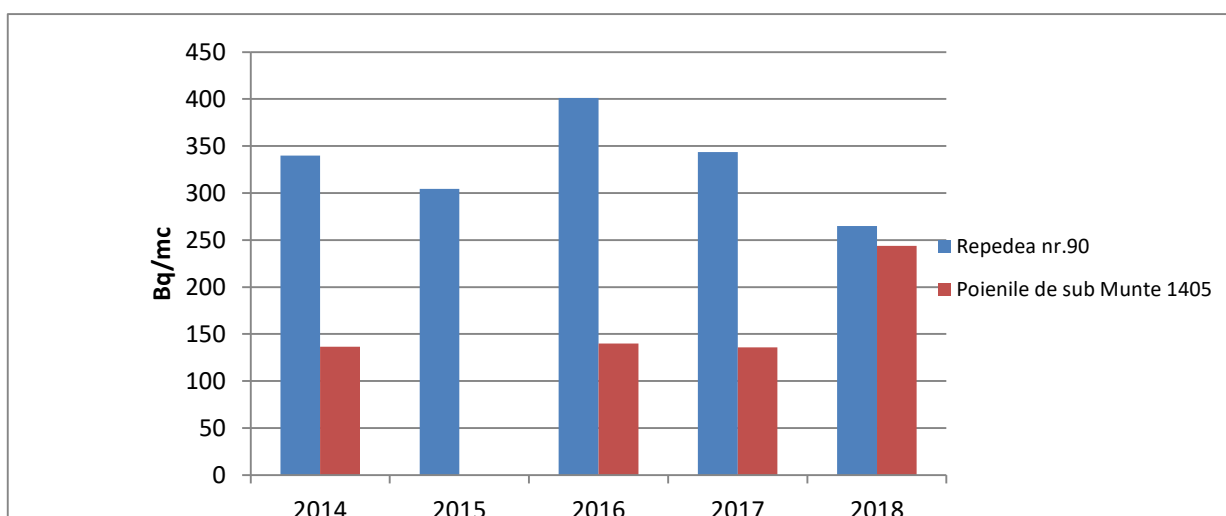
Figura IX.2.2.1. Activități \beta -globale imediate în fântânile monitorizate în zona Repedeș și Poienile de sub Munte în perioada 2014-2018
