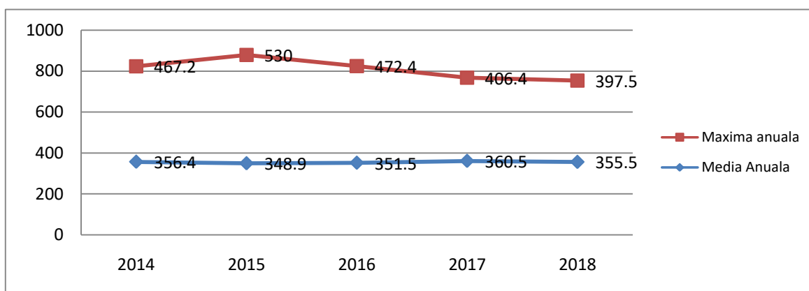
Figura IX.1.3.1. Activitatea specifică \beta -globală pentru sol necultivat din Baia Mare
