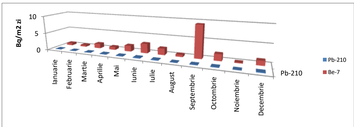
Figura IX.1.2.2. Variația activității specifice lunare a radionuclizilor naturali identificați în probele de depuneri atmosferice totale
