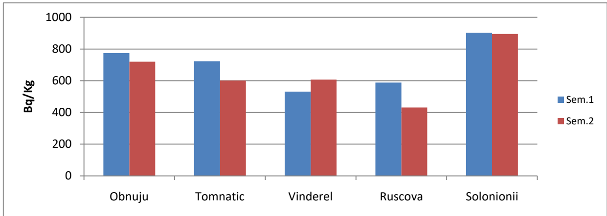
Figura IX.2.4.2. Activități \beta -globale în soluri din zona Repedeș și Poienile de sub Munte în anul 2018
