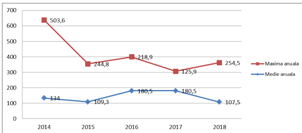
Figura IX.1.2.5. Variația mediilor și maximelor anuale ale activității beta globale a râului Tisa
