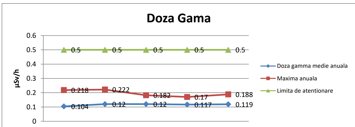
Figura IX.1.1.1.1. Variația mediilor și maximelor anuale ale debitului dozei gama
