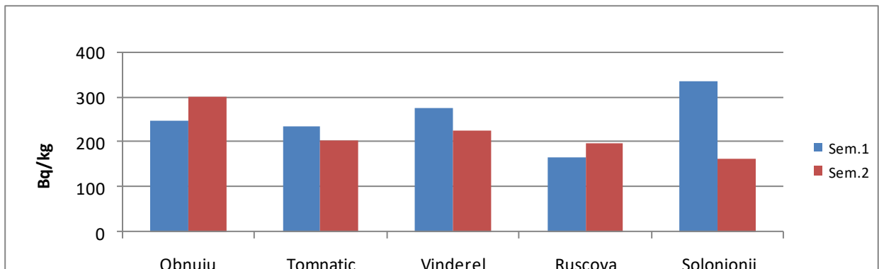
Figura IX.2.5.2. Activități \beta -globale în vegetație spontană din zona Repedea și Poienile de sub Munte în anul 2018
