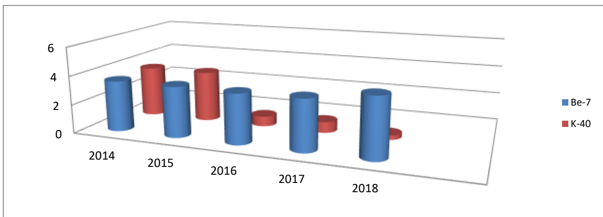
Figura IX.1.1.2.5. Evoluția activității Be-7 și K-40
