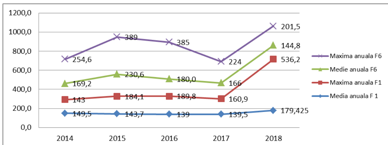
Figura IX.1.2.7. Variația mediilor și maximelor anuale ale activității beta globale a forajelor F 6 Sat Săsar și F 1 Sat Hideaga
