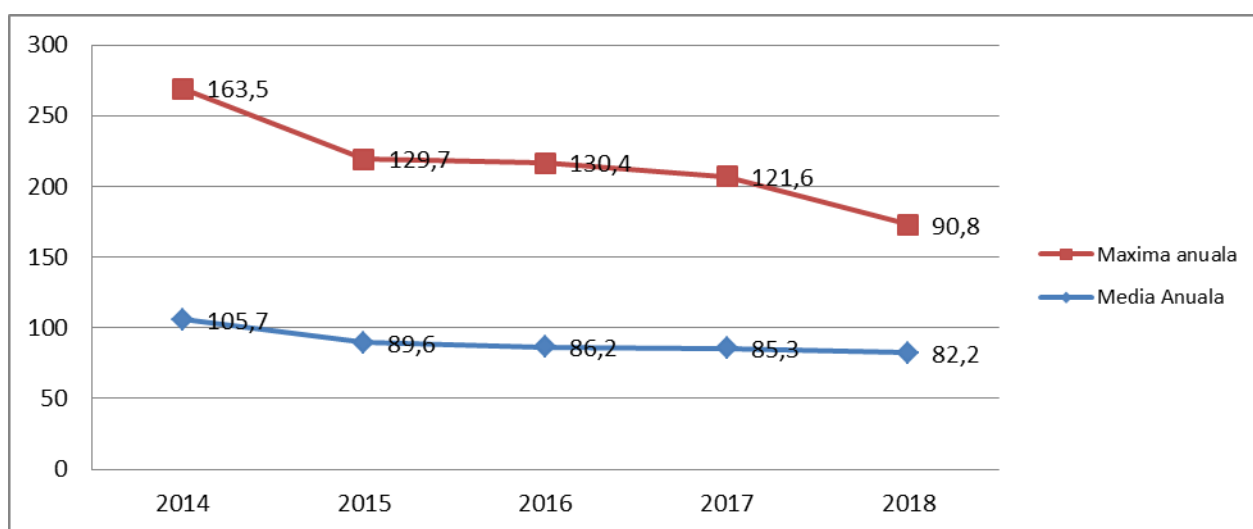
Figura IX.1.2.9. Variația mediilor și maximelor anuale ale activității beta globale Baraj Firiza
