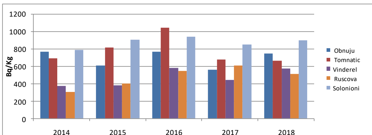
Figura IX.2.4.1. Activități \beta -globale în soluri din zona Repedeș și Poienile de sub Munte în perioada 2014 - 2018
