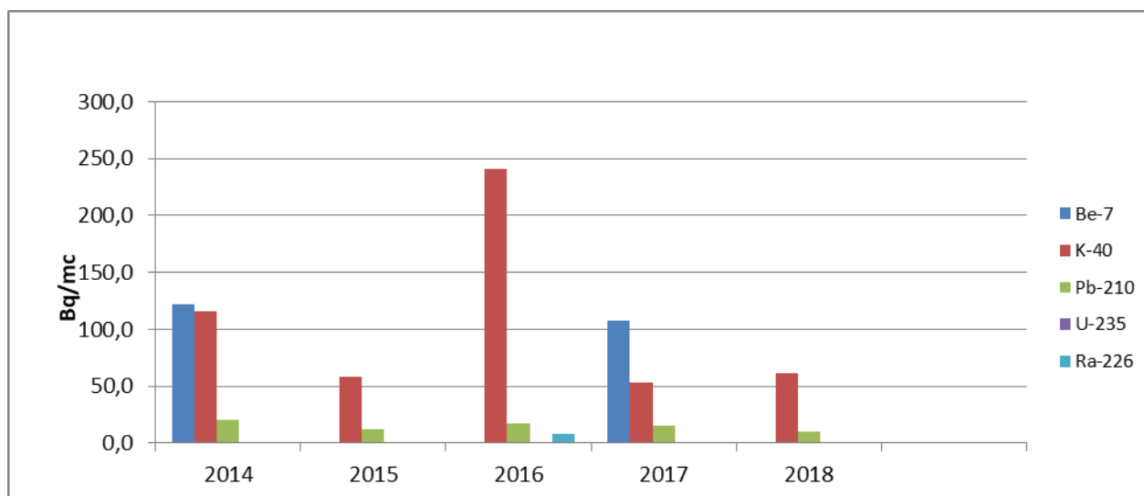
Figura IX.1.2.6. Evoluția activității celor mai frecvenți radionuclizi identificați pentru râul Tisa în perioada 2014-2018
