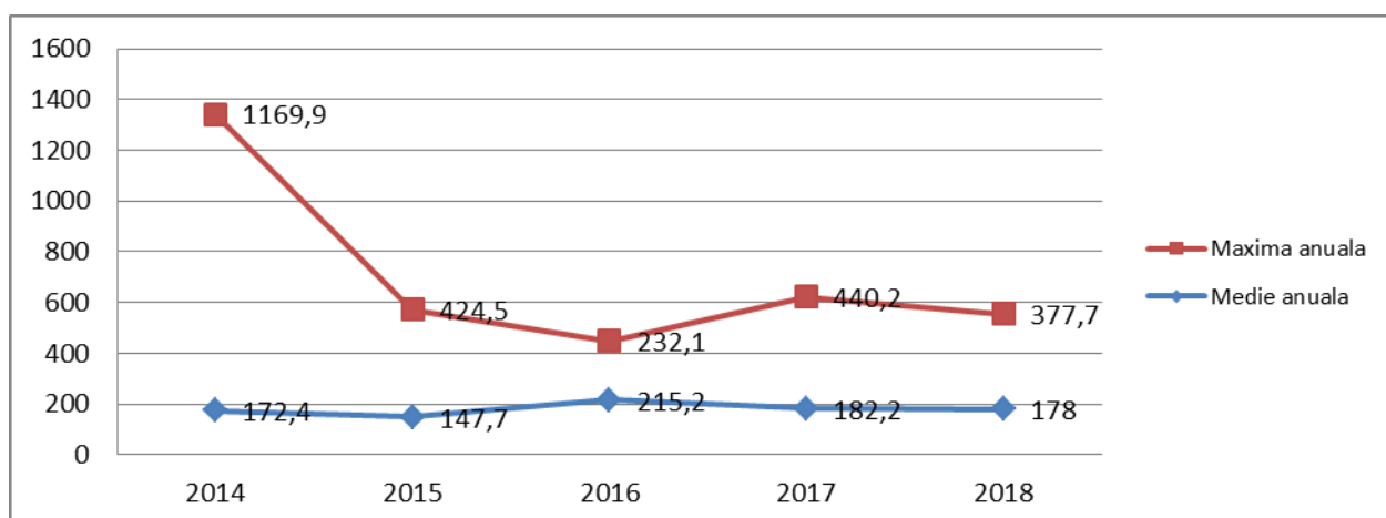
Figura IX.1.2.3. Variația mediilor și maximelor anuale ale activității beta globale a râului Someș
