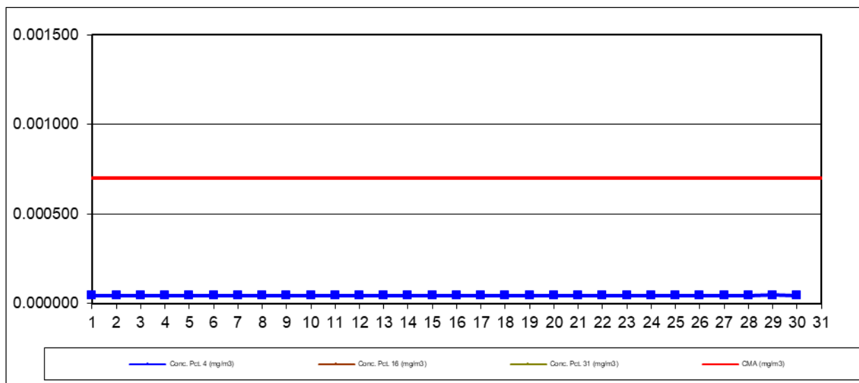
Evoluția indicatorului Cd din TSP in stațiile de monitorizare manuală.
