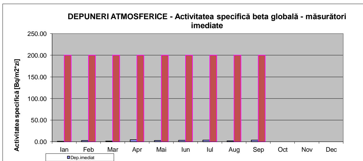
Fig. 1.3.4. Activitatea beta globală pentru depuneri atmosferice
