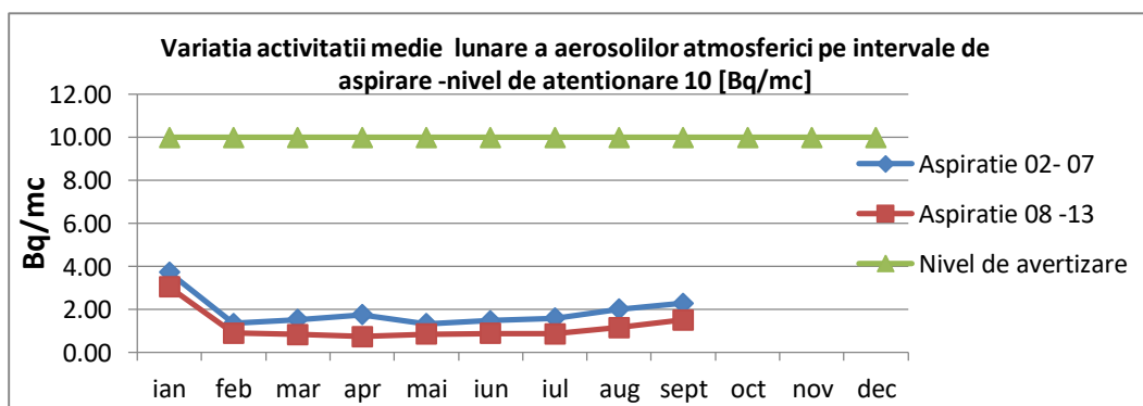
Fig. 1.3.1. Activitatea beta globală pentru aerosoli atmosferici
