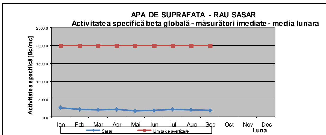
Fig. 1.4.5. Activitatea beta globală imediată pentru apa de suprafață din Râul Săsar (Pod Catedrala).
