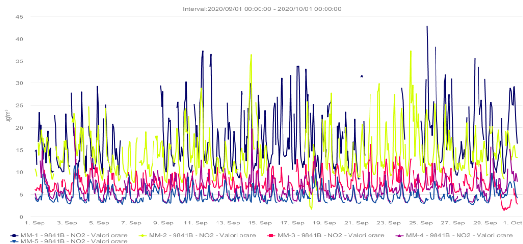
Evoluția indicatorului NO 2 – medii orare
