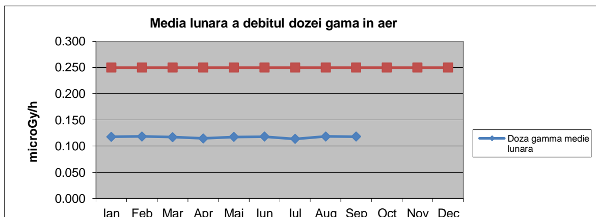
Fig. 1.3.3. Debitul dozei gamma în aer
