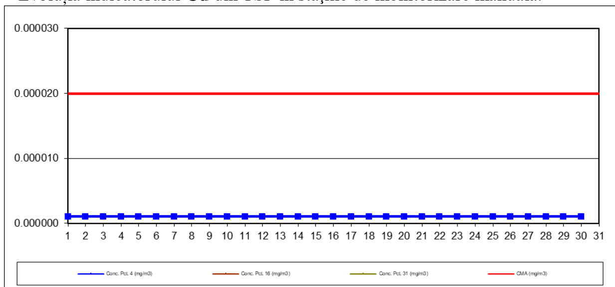
Evoluția indicatorului Cd din TSP in stațiile de monitorizare manuală.
