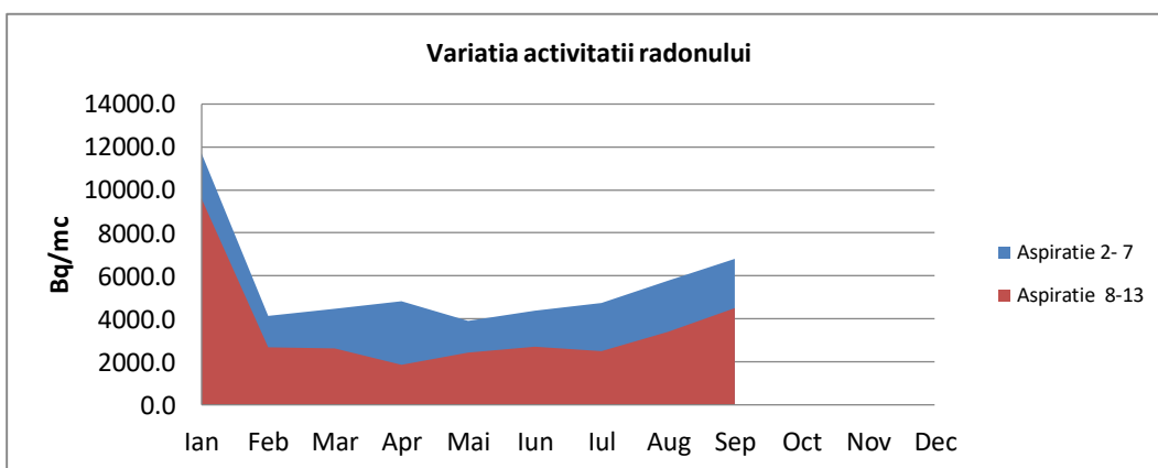
Fig. 1.3.2. Activitatea calculată a Radonului
