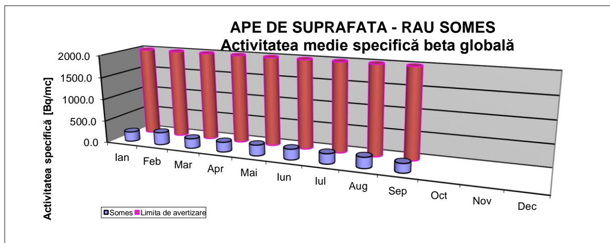
Fig. 1.3.6. Activitatea beta globală măsurată retard la 5 zile pentru apa de suprafață - Râul Someș
