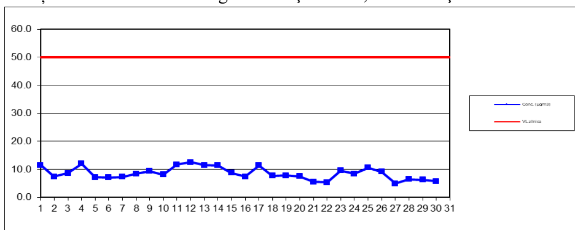
Evoluția indicatorului PM10 grav – Stația MM4, concentrații medii zilnice
