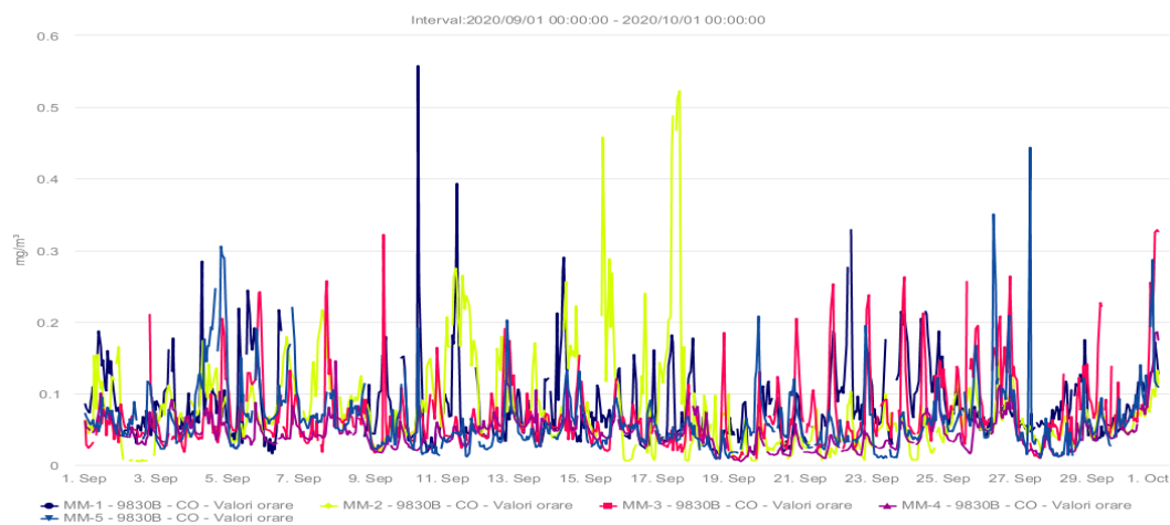
Evoluția indicatorului CO – medii orare
