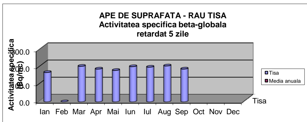
Fig. 1.3.7. Activitatea beta globală măsurată retard la 5 zile pentru apa de suprafață - Râul Tisa
