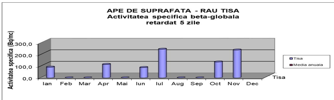
Fig. 2.3.7. Activitatea beta globală măsurată retard la 5 zile pentru apa de suprafață - Râul Tisa
