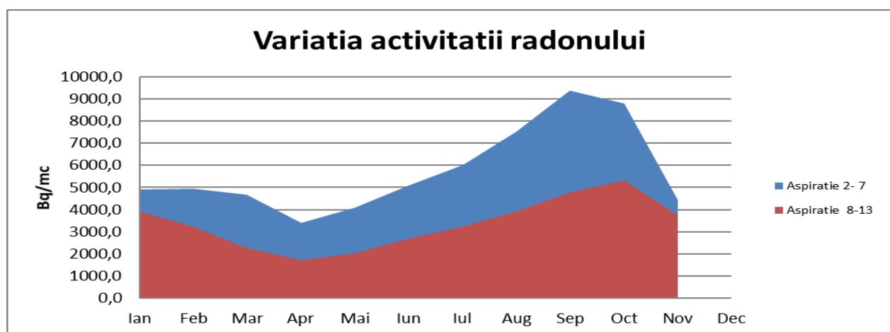
Fig. 2.3.2. Activitatea calculată a Radonului
