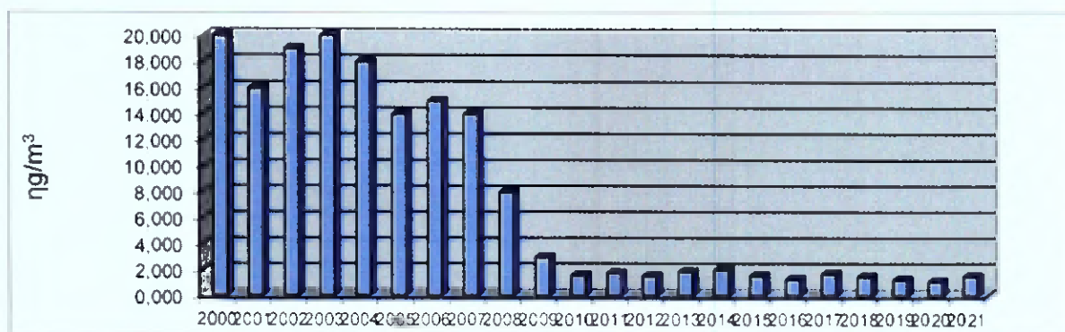
Concentrații de Cd (din TSP) în aer - stații manuale medii anuale - Baia Mare în perioada 2000 – 2021
