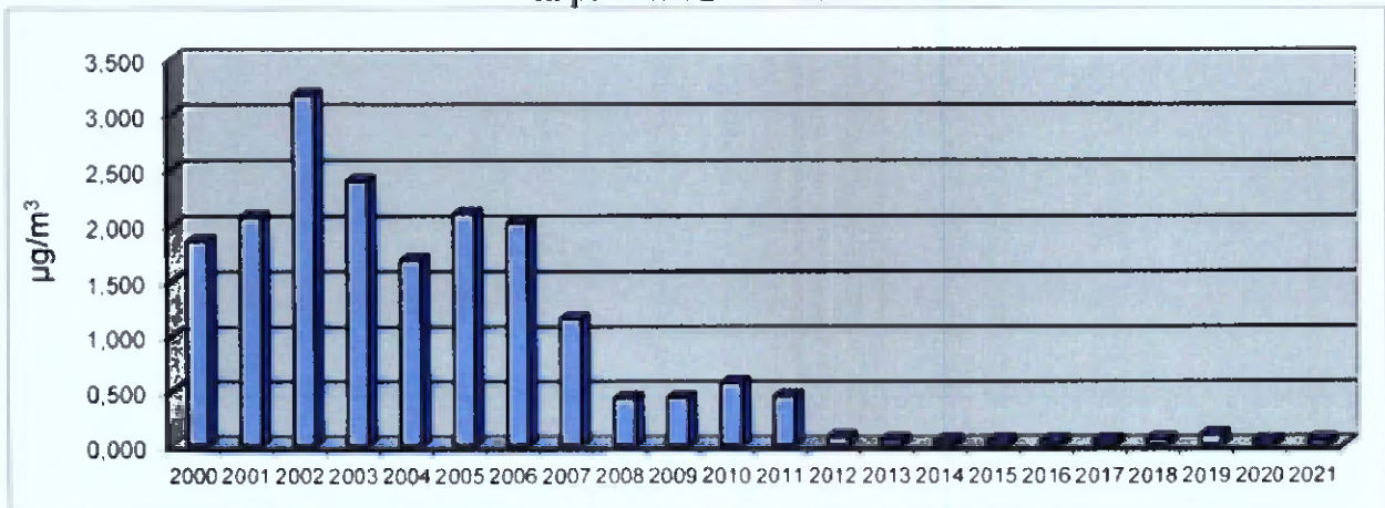
Evoluția concentrației de Pb (din TSP) în aer - stații manuale medii anuale - Baia Mare în perioada 2000 - 2021
