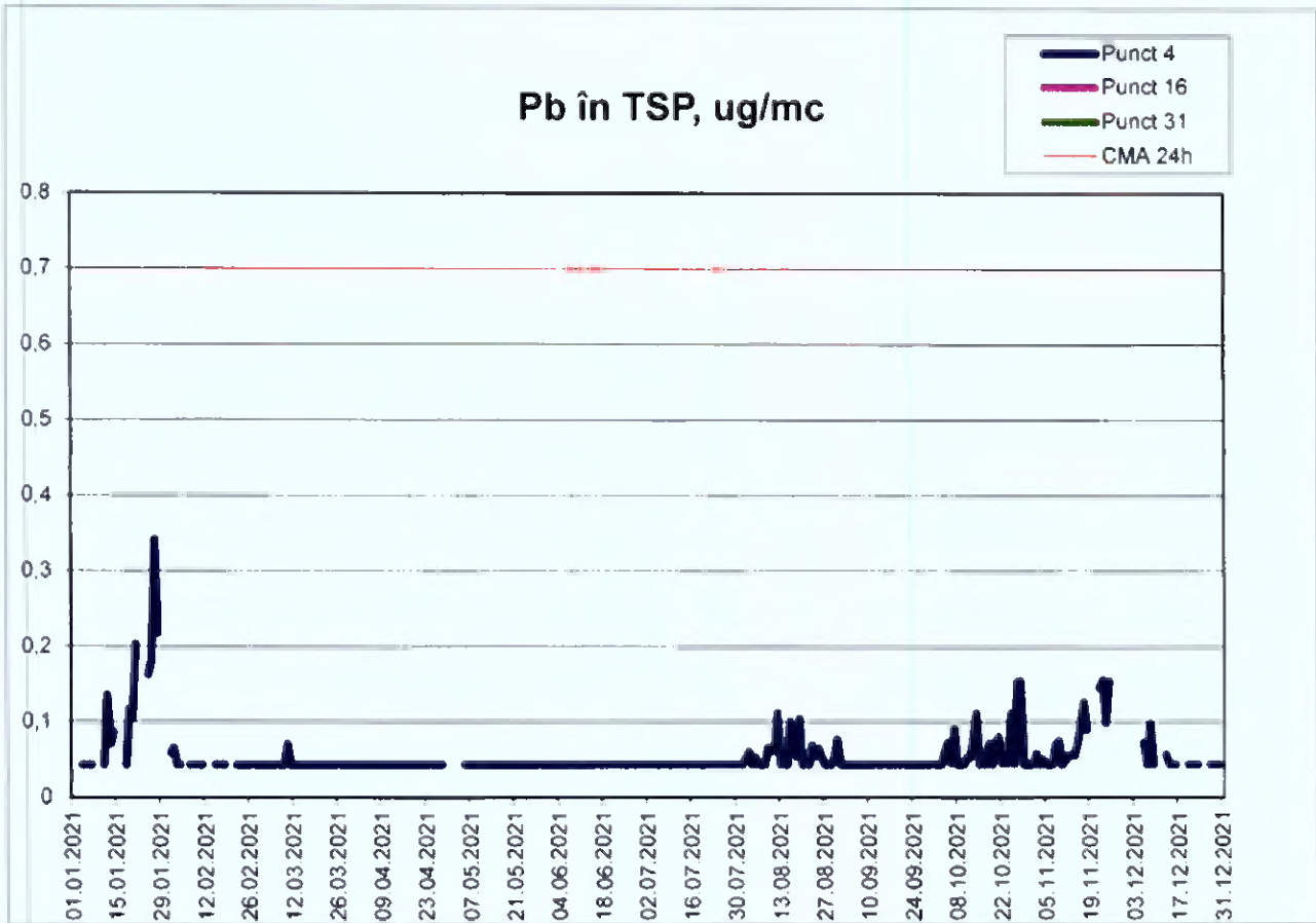
Evoluția concentrației de Pb (din TSP) în aer - stații manuale medii zilnice - Baia Mare - anul 2021
