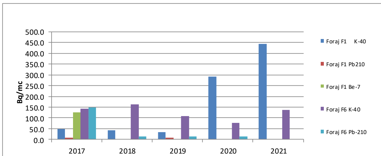
Figura IX.1.2.8. Evoluția activității celor mai frecvenți radionuclizi identificați pentru cele două foraje în perioada 2017 – 2021
