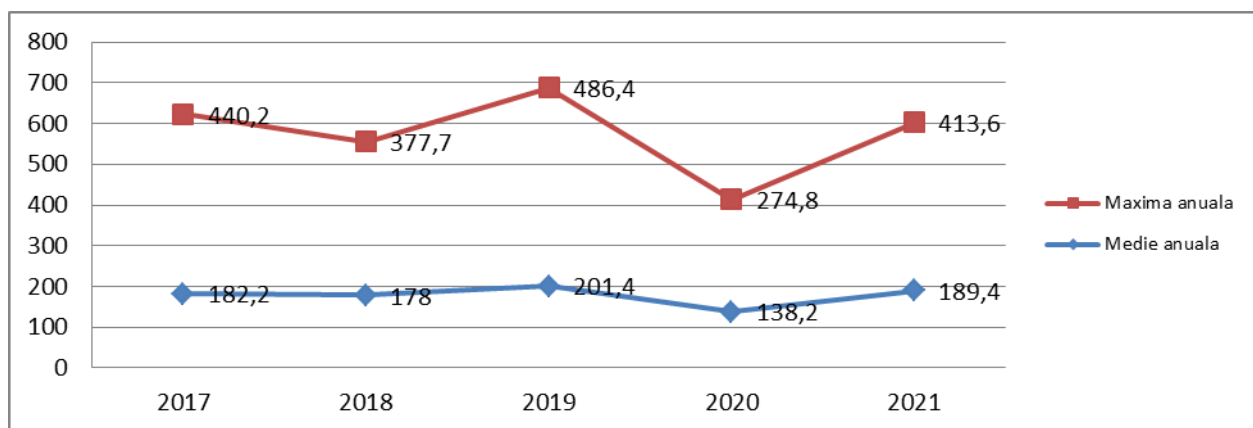
Figura IX.1.2.3. Variația mediilor și maximelor anuale ale activității beta globale a râului Someș
