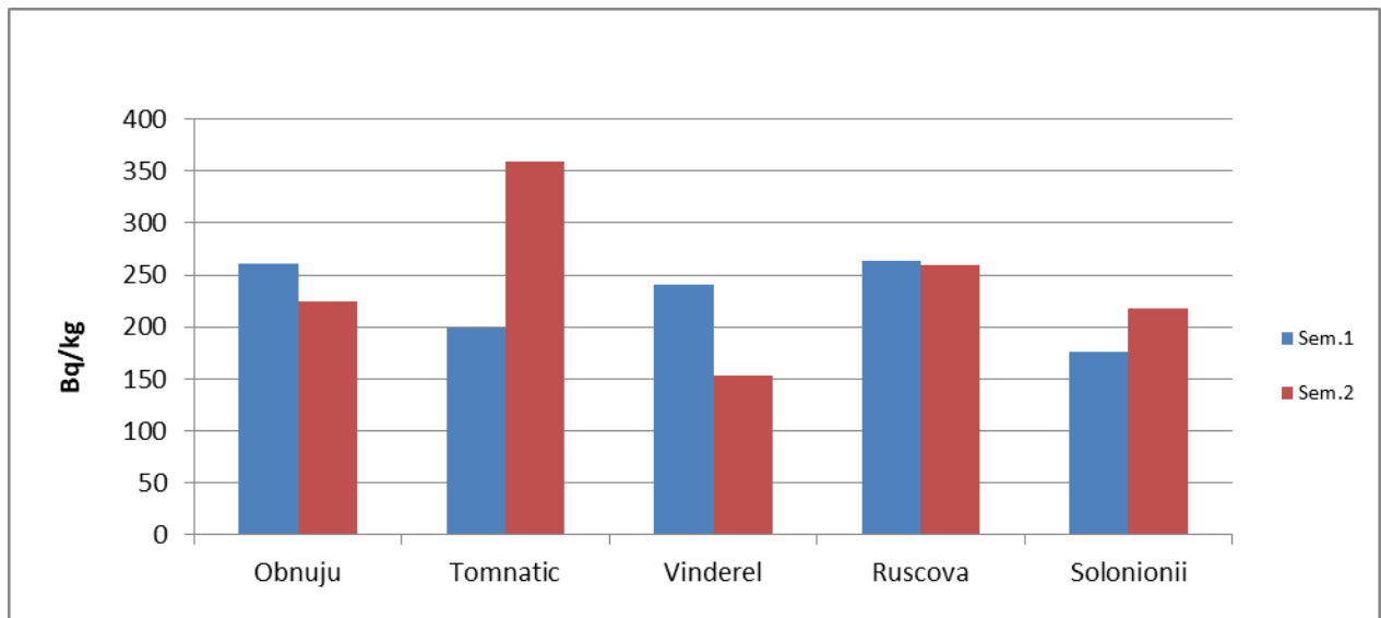
Figura IX.2.5.2. Activități \beta -globale în vegetație spontană din zona Repedeș și Poienile de sub Munte în anul 2021
