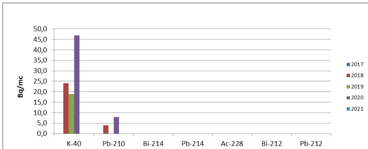
Figura IX.1.2.10. Evoluția activității celor mai frecvenți radionuclizi identificați pentru Baraj Firiza în perioada 2017 – 2021
