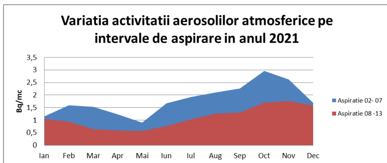
Figura IX.1.1.2.1. Variația medie anuală a activității Beta globală imediată a aerosolilor atmosferici în funcție de variația diurnă
