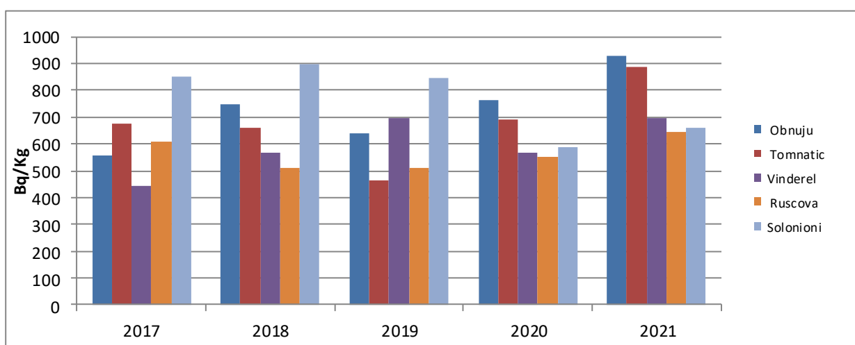
Figura IX.2.4.1. Activități \beta -globale în soluri din zona Repedeș și Poienile de sub Munte în perioada 2017 - 2021
