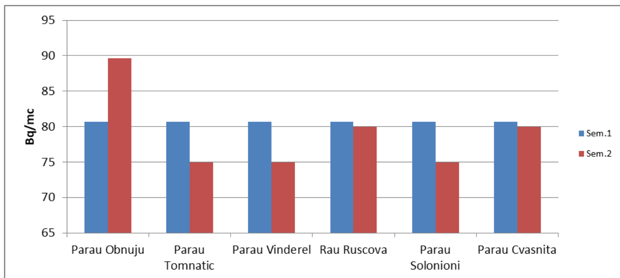
Figura IX.2.1.2. Măsurători \beta - globale pentru apa de suprafață în zona Repedea și Poienile de sub Munte în anul 2021
