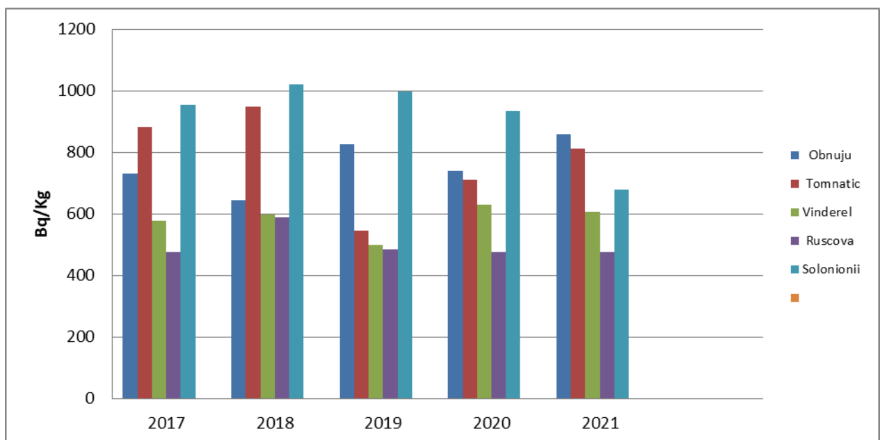
Figura IX.2.4.3. Nivelul activității K - 40 în sol necultivat din zona Repedeș și Poienile de sub Munte în perioada 2017 - 2021
