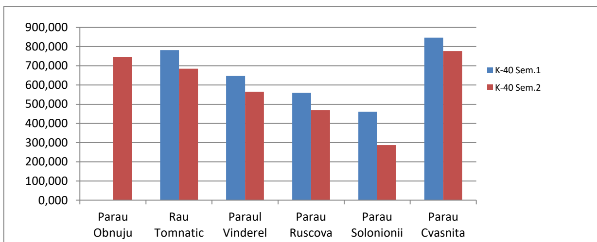
Figura IX.2.3.1. Nivelul activității K-40 în sedimente din zona Repedea și Poienile de sub Munte în anul 2021
