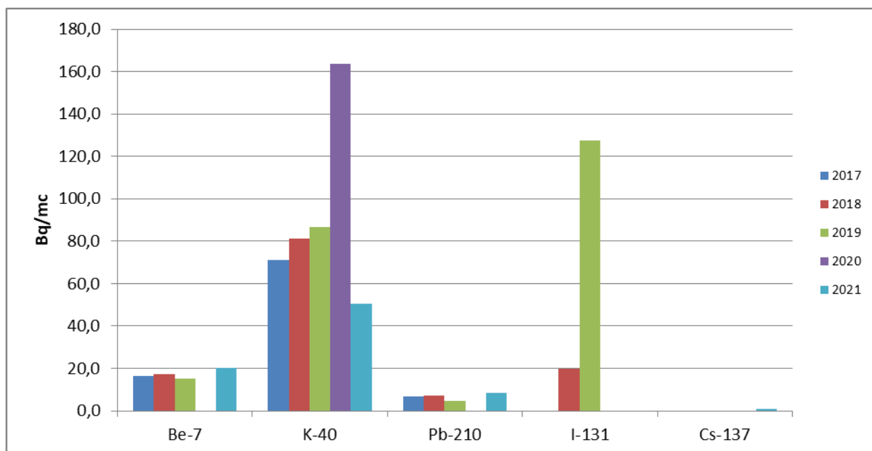
Figura IX.1.2.2. Evoluția activității celor mai frecvenți radionuclizi identificați pentru râul Săsar în perioada 2017 – 2021
