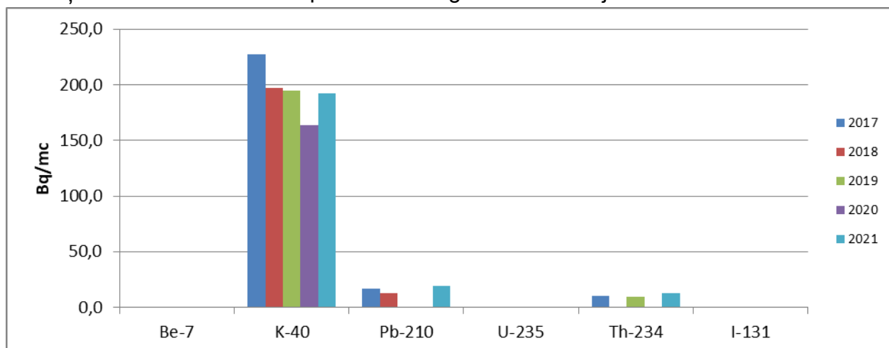
Figura IX.1.2.4. Evoluția activității celor mai frecvenți radionuclizi identificați pentru râul Someș în perioada 2017 - 2021
