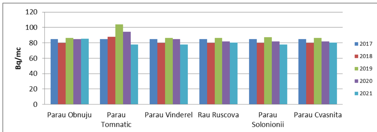
Figura IX.2.1.1. Activitatea \beta -globală pentru apa de suprafață în zona Repedea și Poienile de sub Munte
