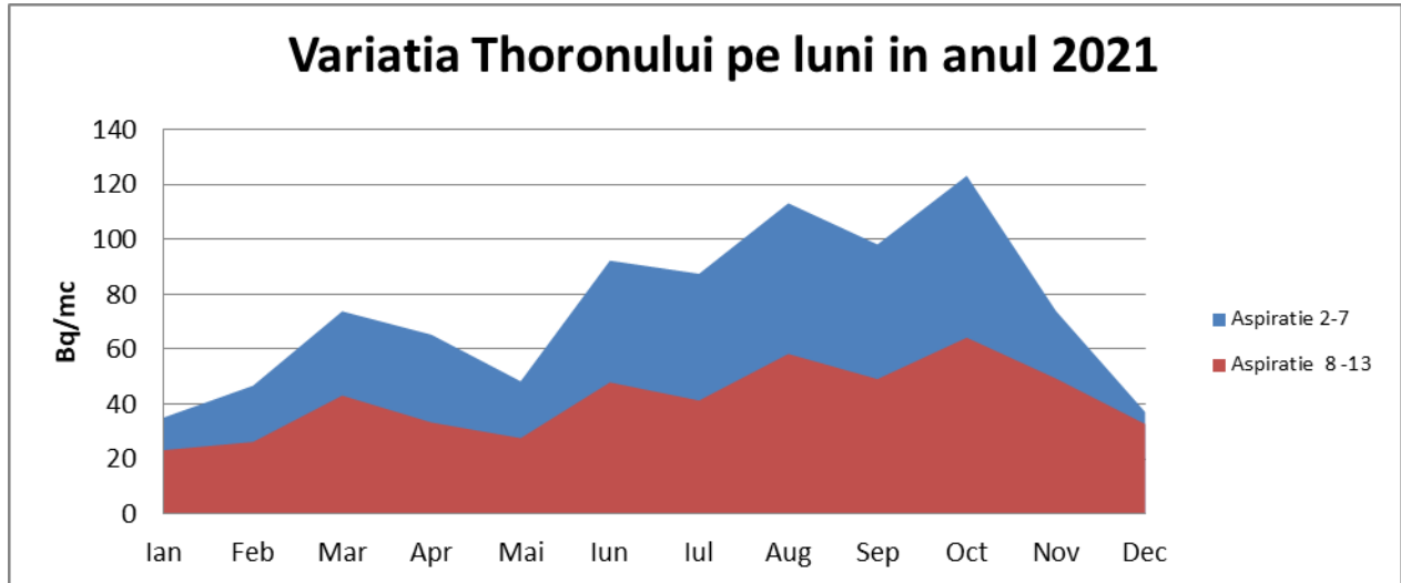
Figura IX.1.1.2.4. Variația activităților specifice medii anuală a toronului din atmosferă în funcție de variația diurnă
