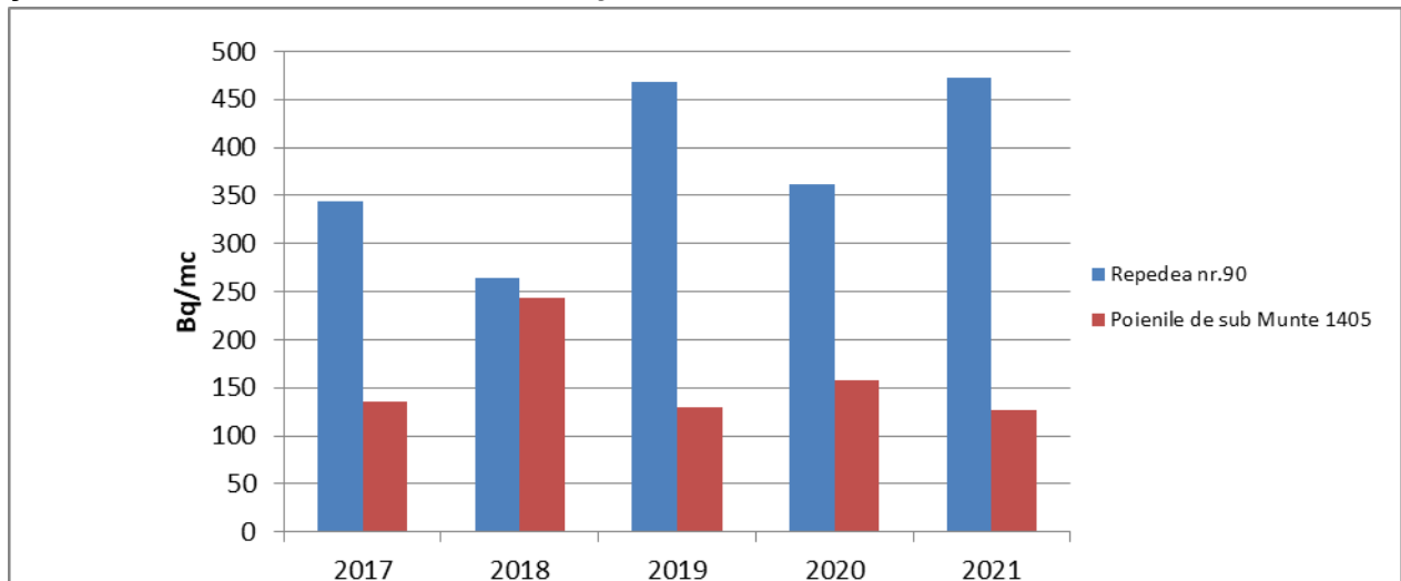
Figura IX.2.2.1. Activități \beta -globale imediate în fântânile monitorizate în zona Repedea și Poienile de sub Munte în perioada 2017-2021
