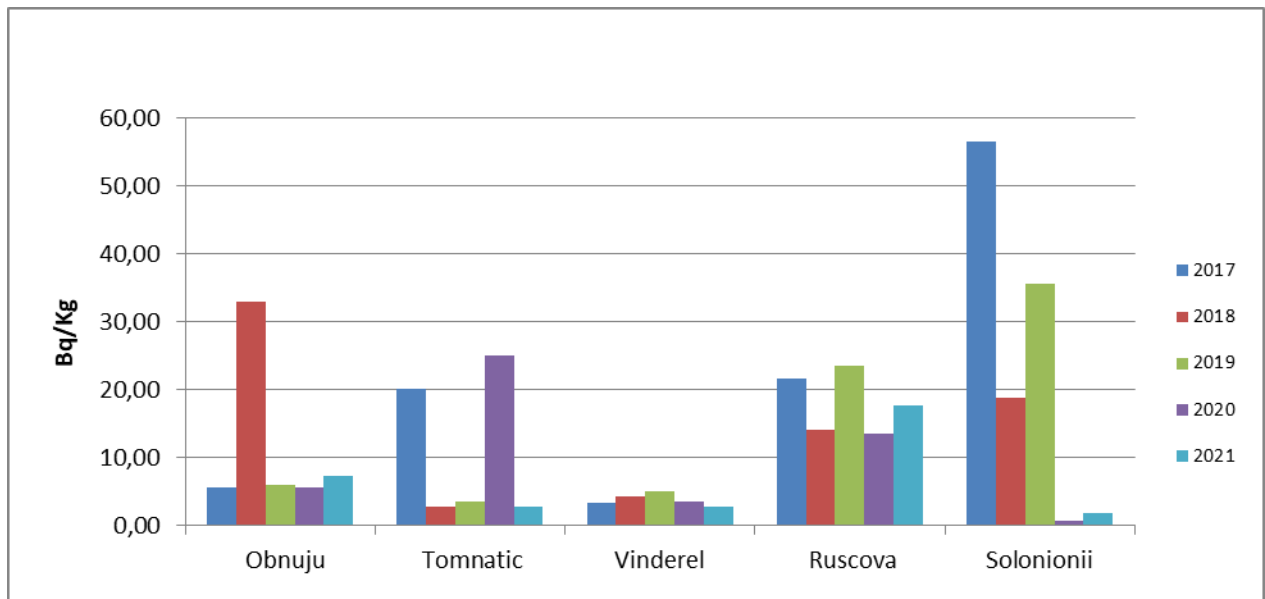
Figura IX.2.4.4. Nivelul activității Cs-137 în sol necultivat din zona Repedeș și Poienile de sub Munte în perioada 2017 - 2021
