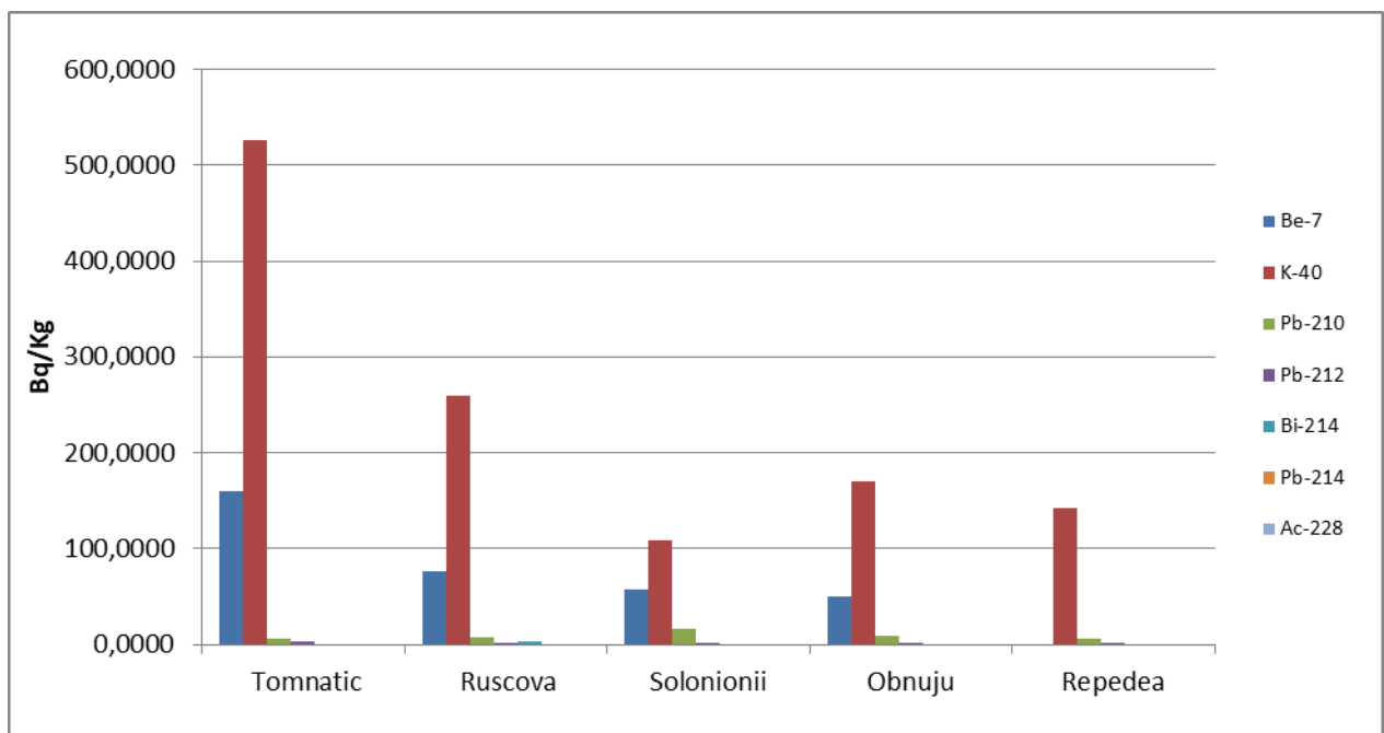
Figura IX.2.5.3. Nivelul activității radionuclizilor indentificati în vegetație spontană din zona Repedeș și Poienile de sub Munte în anul 2021
