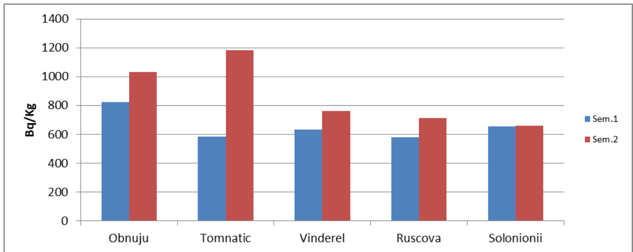
Figura IX.2.4.2. Activități \beta -globale în soluri din zona Repedeș și Poienile de sub Munte în anul 2021
