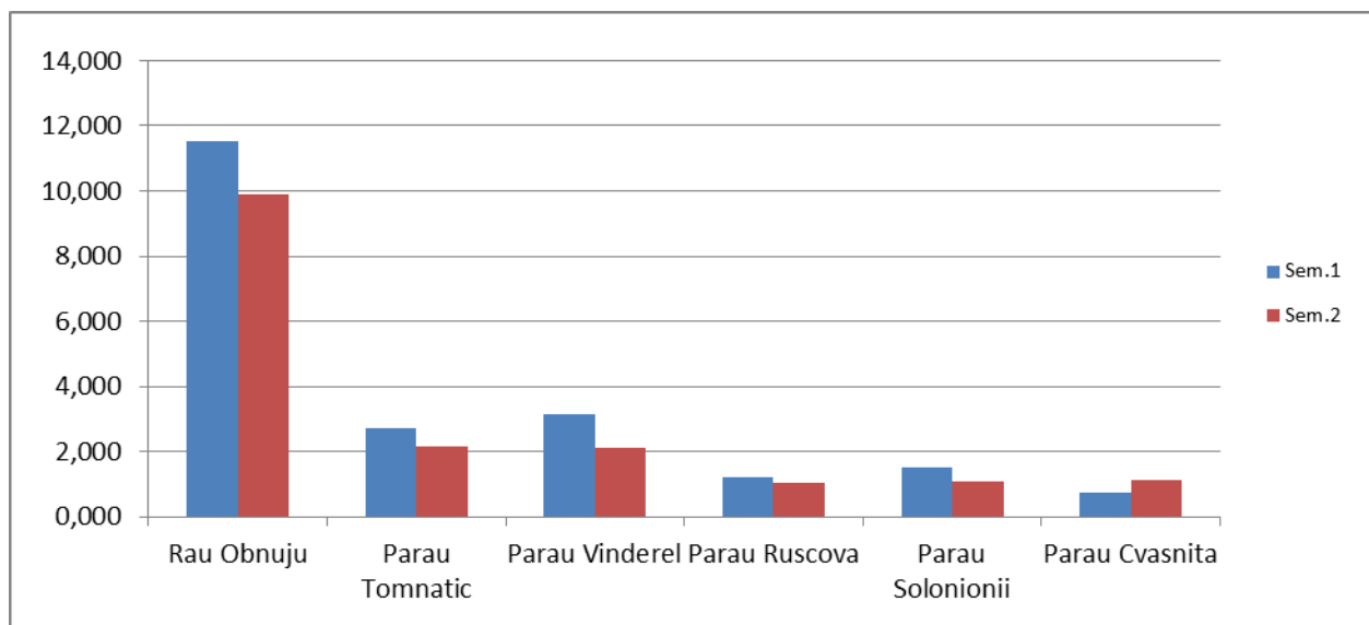
Figura IX.2.3.2. Nivelul activității Cs-137 în sedimente din zona Repedeș și Poienile de sub Munte în anul 2021
