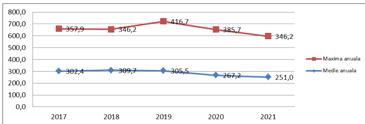
Figura IX.1.4.1. Activitatea specifică \beta -globală pentru vegetație spontană
