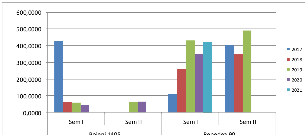
Figura IX.2.2.2. Nivelul activității K-40 în apa din fântâni, în zona Repedea și Poienile de sub Munte în anul 2017 – 2021
