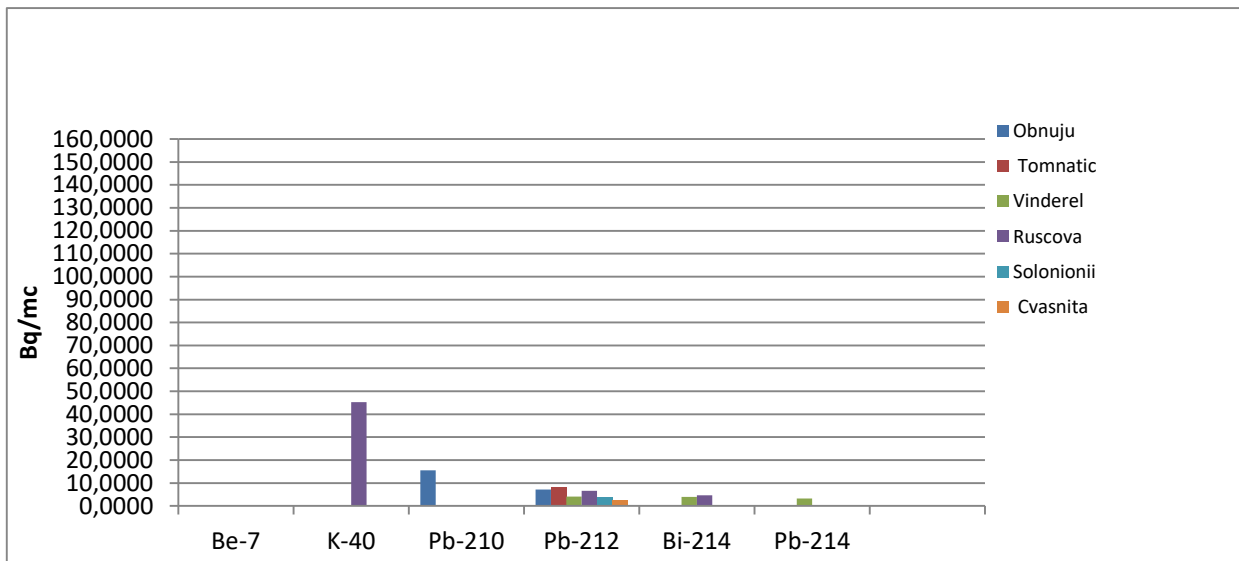
Figura IX.2.1.3. Nivelul activităților radionuclizilor identificați în apa de suprafață din zona Repedea și Poienile de sub Munte în anul 2021
