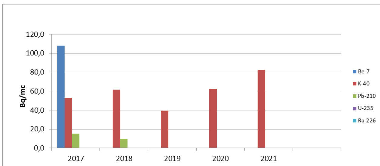
Figura IX.1.2.6. Evoluția activității celor mai frecvenți radionuclizi identificați pentru râul Tisa în perioada 2017-2021
