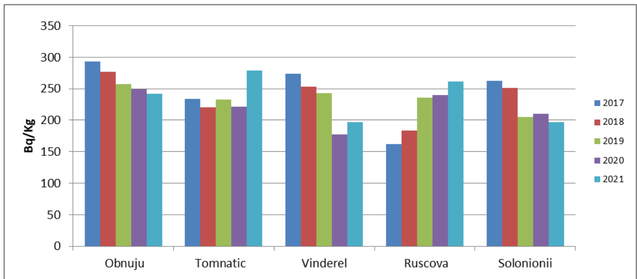
Figura IX.2.5.1. Activități \beta -globale în vegetație spontană din zona Repedeș și Poienile de sub Munte în perioada 2017 – 2021
