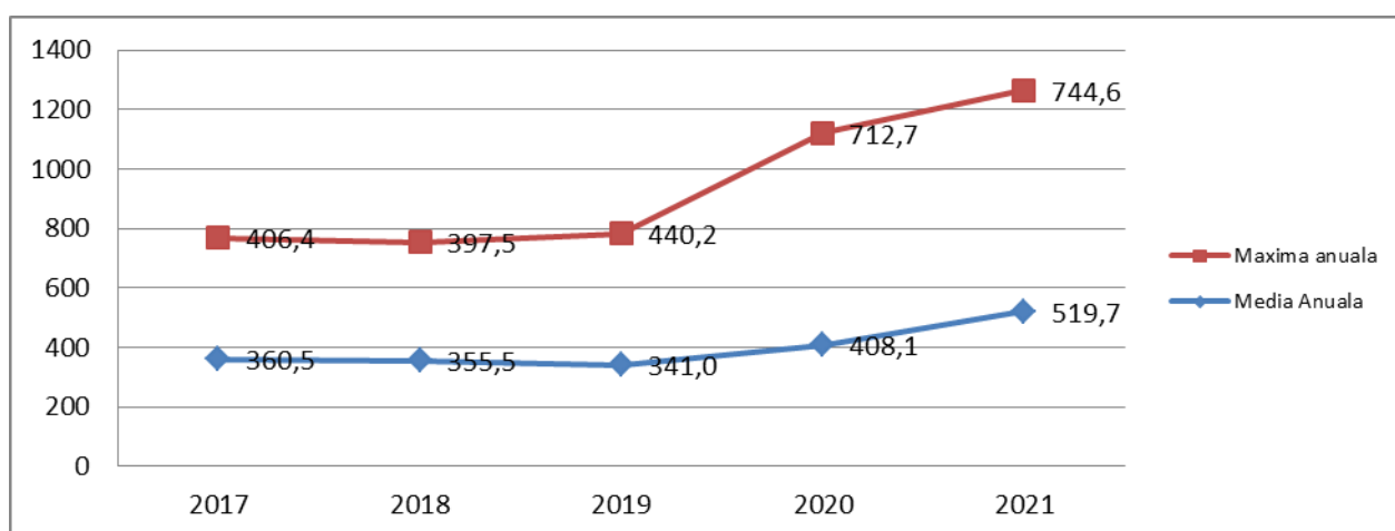
Figura IX.1.3.1. Activitatea specifică \beta -globală pentru sol necultivat din Baia Mare
