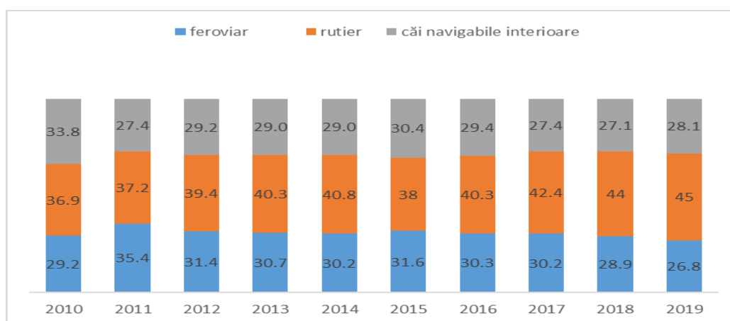
Figura X.1.3.2.2. Ponderea fiecărui mod de transport în transportul de mărfuri (Sursa: http://www.insse.ro/cms/files/Web_IDD_BD_ro/index.htm )
