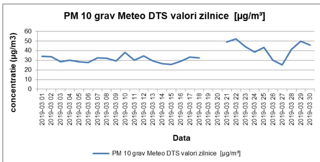
Graficul nr. 8- Concentrații pulberi în suspensie- fracția PM 10 (CMA=50 (µg/m 3 ))
