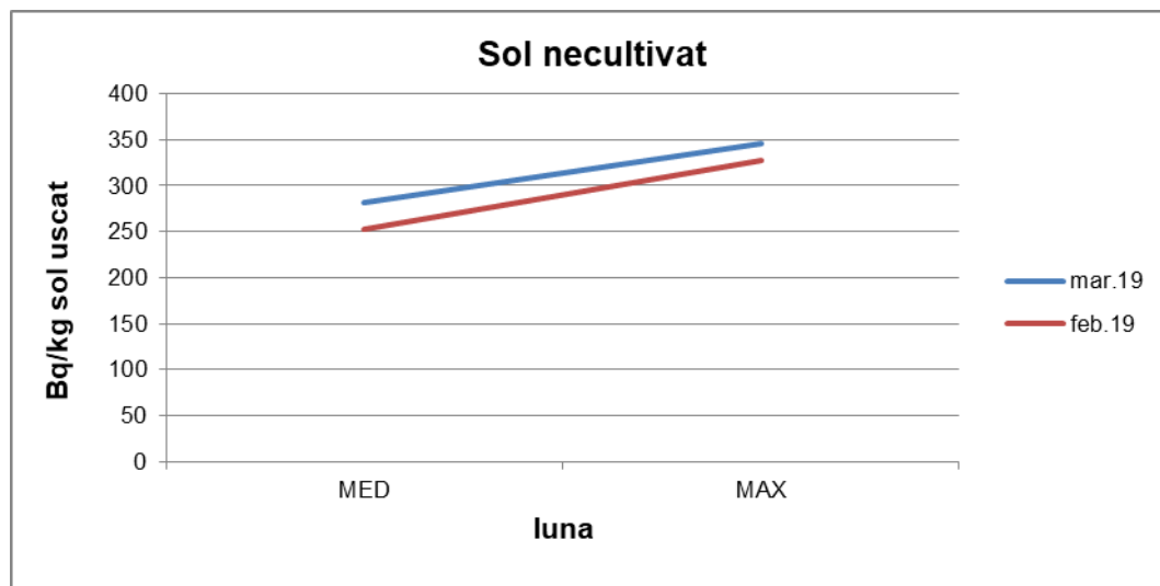
Graful nr. 14. - Valorile radioactivității artificiale în probele de sol necultivat
