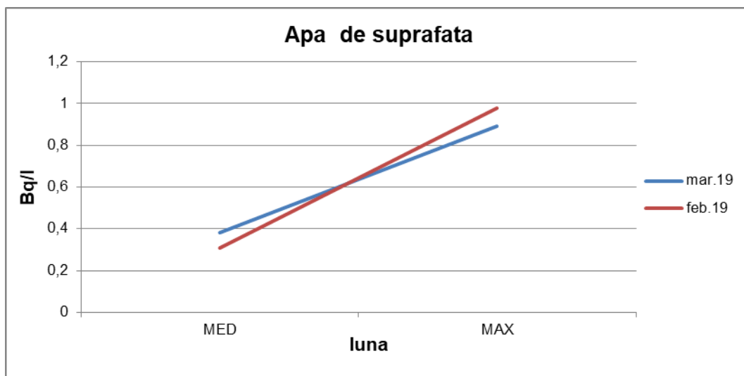
Graficul nr. 13.- Evoluția radioactivității pentru apa de suprafață (fluviul Dunărea)
