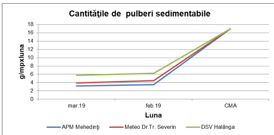
Graficul nr.7. – Concentrații lunare de pulberi sedimentabile
