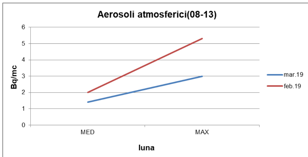
Graficul nr. 11.- Aerosoli atmosferici (măsurători imediate) - activitate specifică beta globală - intervalul 08-13
