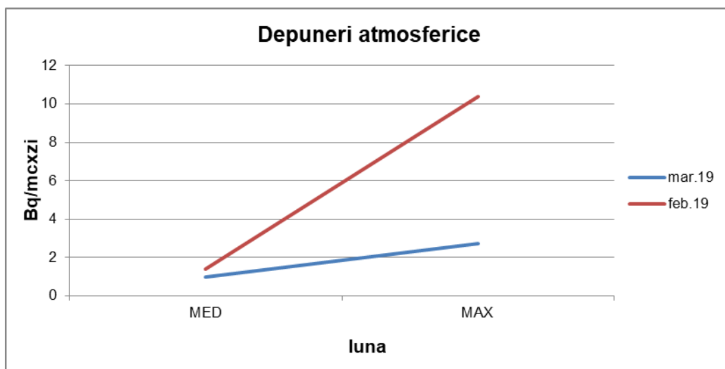
Graficul nr. 12. - Evoluția radioactivității artificiale depuneri atmosferice
