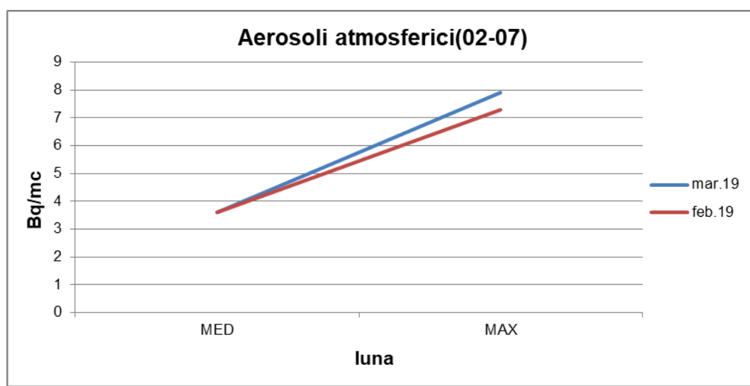
Graficul nr. 10.- Aerosoli atmosferici (măsurători imediate) - activitate specifică beta globală - intervalul 02-07
