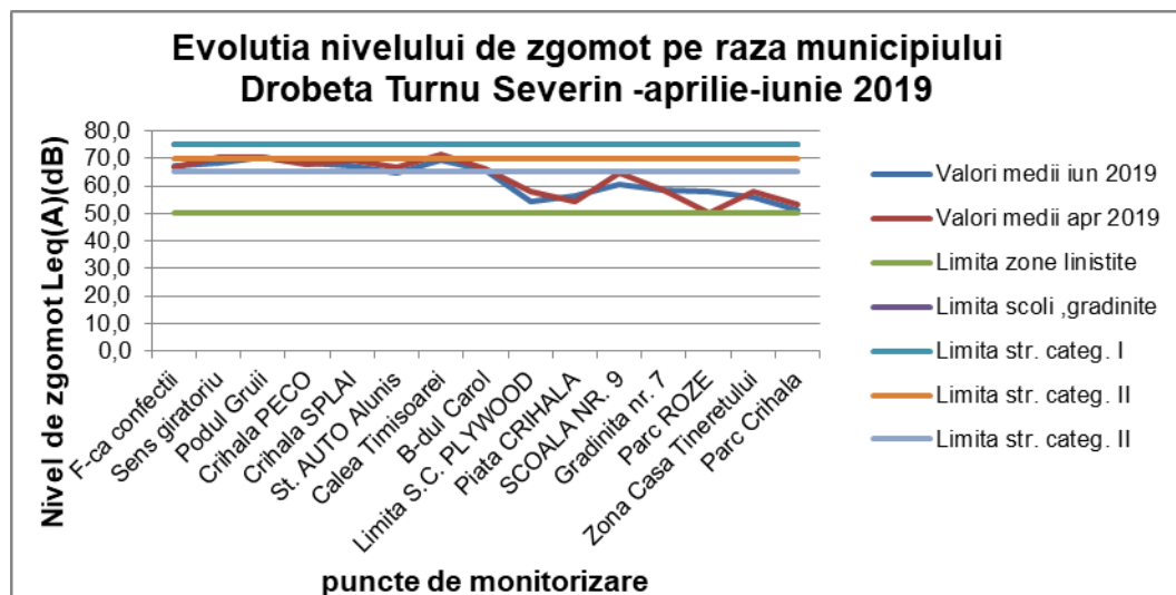
Graficul nr.14. – Nivelul de zgomot în Drobeta Turnu Severin
