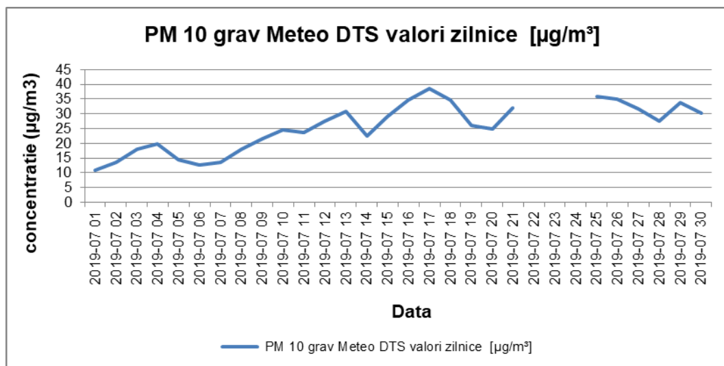
Graficul nr. 12. - Concentrații pulberi in suspensie-fracția PM 10
