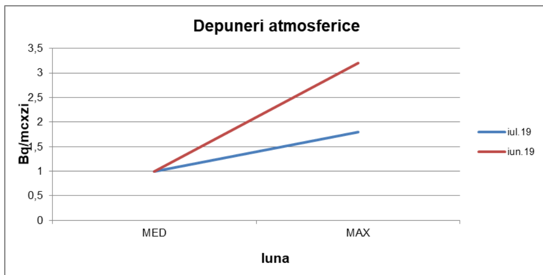
Graficul nr. 16. - Evoluția radioactivității artificiale depuneri atmosferice
