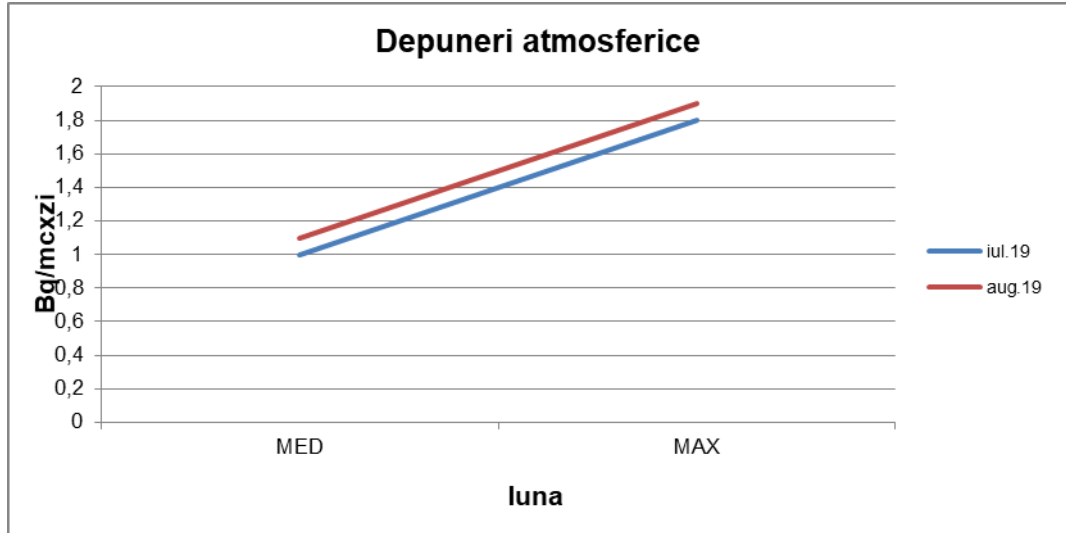
Graficul nr. 14. - Evoluția radioactivității artificiale depuneri atmosferice
