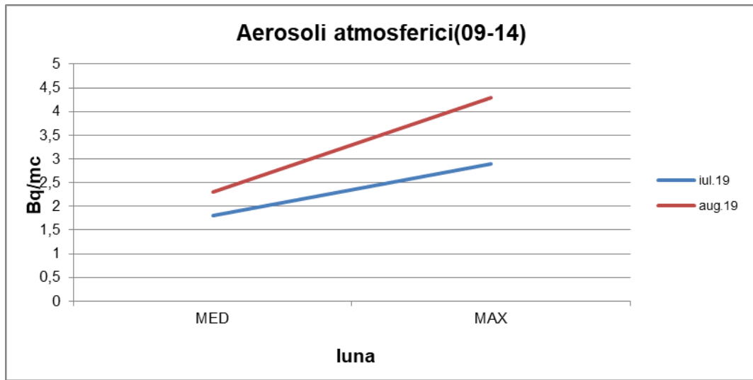
Graficul nr. 13.- Aerosoli atmosferici (măsurători imediate) - activitate specifică beta globală - intervalul 09-14
