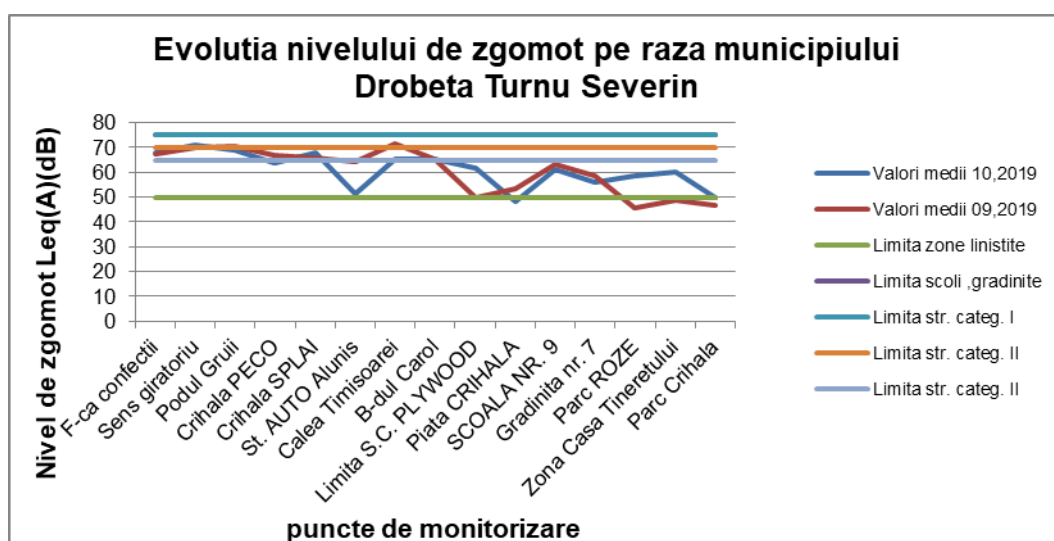
Graficul nr.13. – Nivelul de zgomot în Drobeta Turnu Severin
