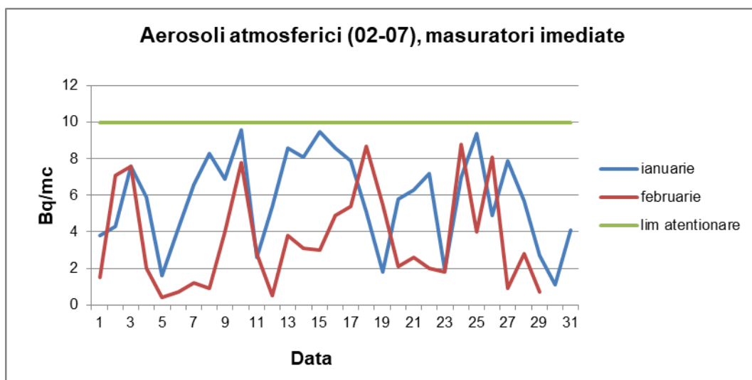
Graficul nr. 15.- Aerosoli atmosferici - activitate specifică beta globală - intervalul 02-07
