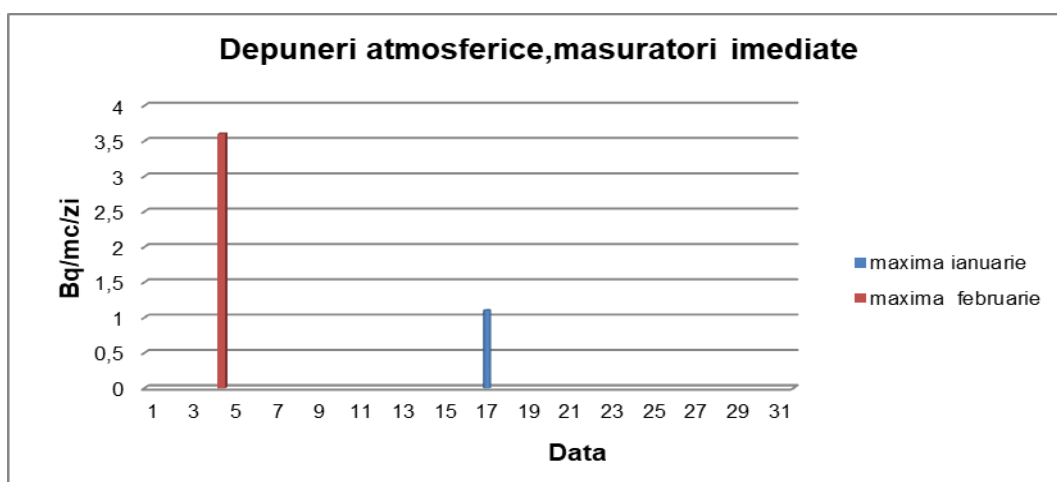
Graficul nr. 17.- Depuneri atmosferice imediate - activitate specifică beta globală
