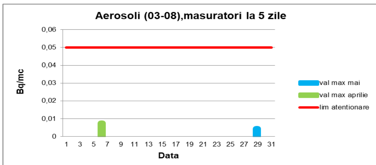
Graficul nr. 17.- Aerosoli atmosferici - activitate specifică beta globală - intervalul 03-08
