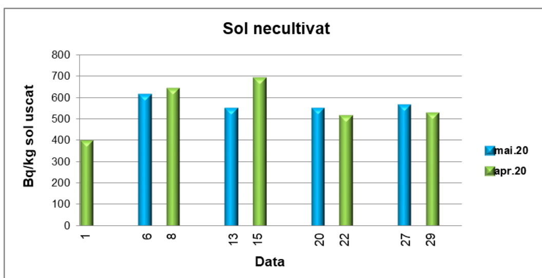
Graficul nr. 23.- sol necultivat - activitate specifică beta globală
