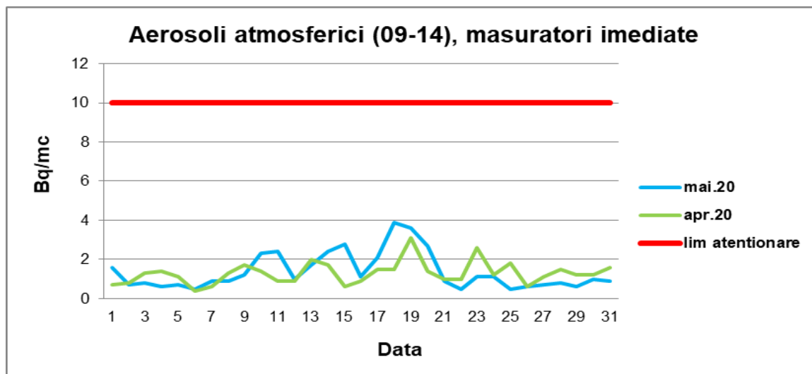
Graficul nr. 16.- Aerosoli atmosferici - activitate specifică beta globală - intervalul 09-14
