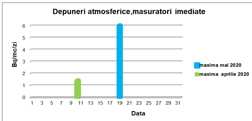
Graficul nr. 19.- Depuneri atmosferice imediate - activitate specifică beta globală
