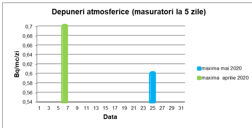
Graficul nr. 20.- Depuneri atmosferice– măsurători la 5 zile - activitate specifică beta globală
