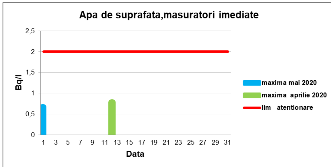
Graficul nr. 21.- apa de suprafață - activitate specifică beta globală
