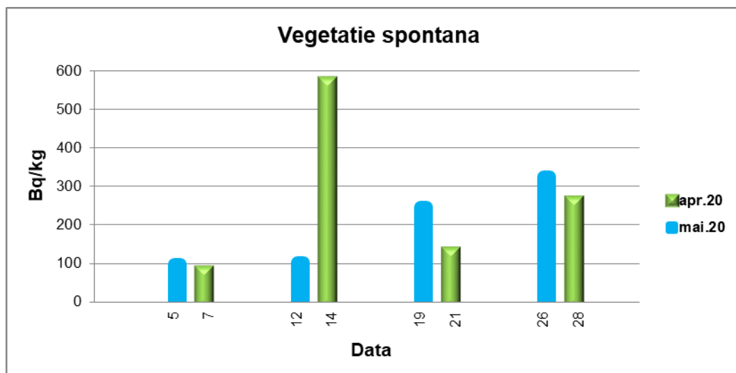
Graficul nr. 24.- Valorile radioactivității artificiale în probele de vegetația spontană
