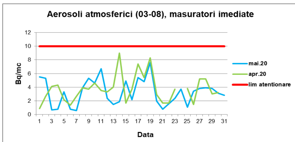
Graficul nr. 15.- Aerosoli atmosferici - activitate specifică beta globală - intervalul 03-08
