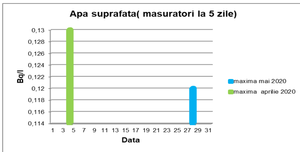
Graficul nr. 22.- apa de suprafață - activitate specifică beta globală
