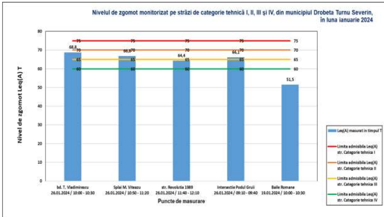
Graficul nr. 15- Nivelul de zgomot urban pe străzi de categorie tehnică I, II, III și IV, în municipiul Drobeta Turnu Severin, în luna ianuarie 2024
