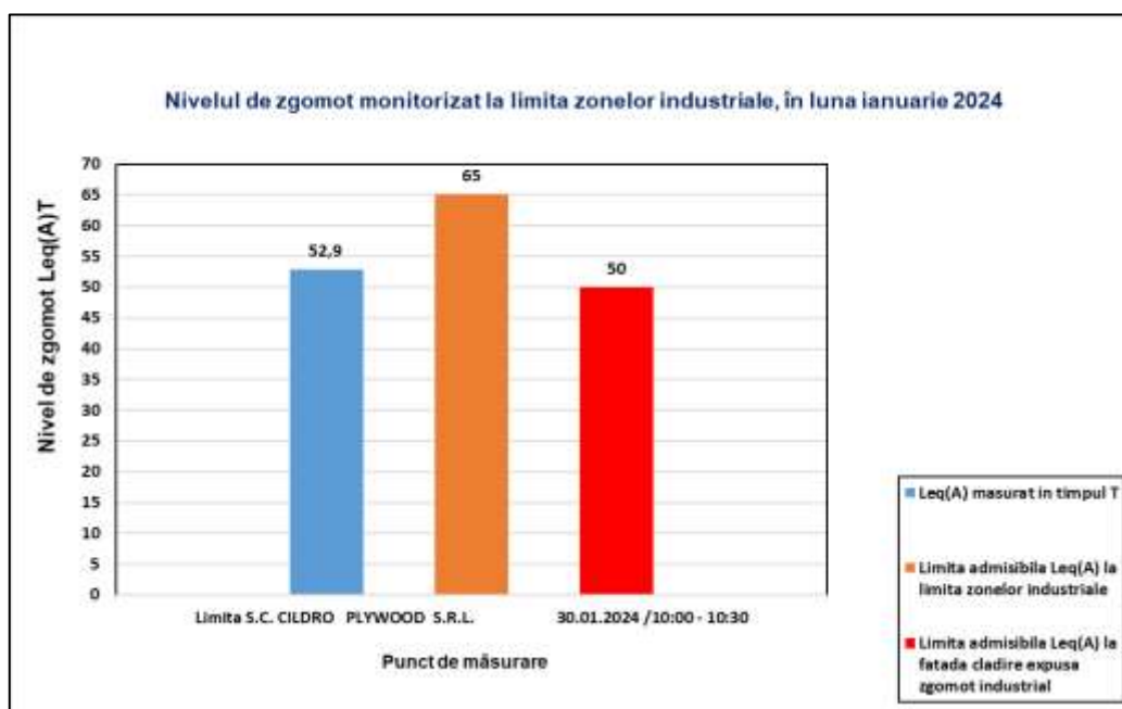
Graficul nr. 17-Nivelul de zgomot la limita zonelor industriale, din municipiul Drobeta Turnu Severin, în luna ianuarie 2024
