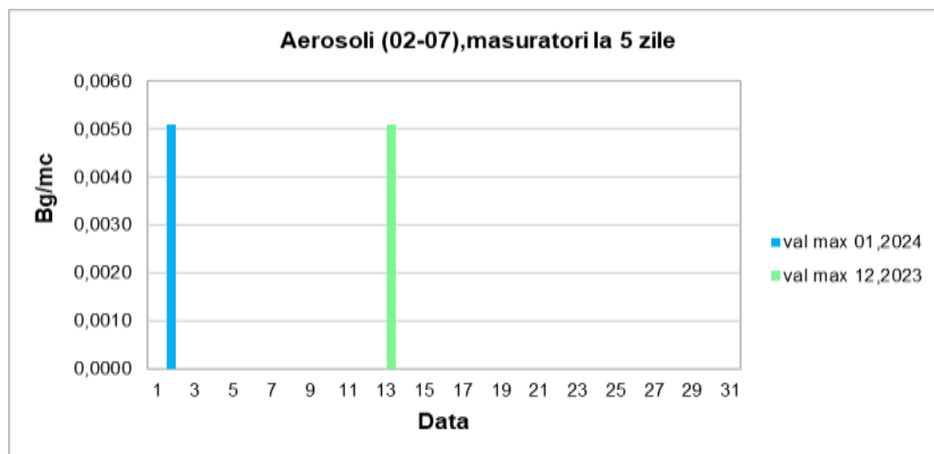
Graficul nr. 6.- Aerosoli atmosferici - activitate specifică beta globală - intervalul 02-07
