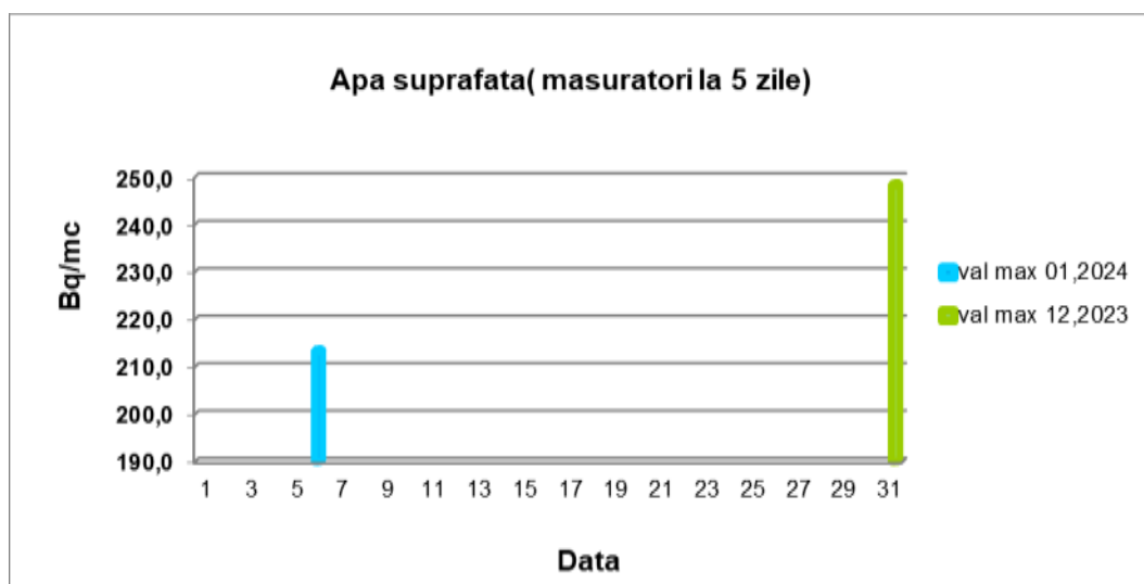
Graficul nr. 11.- apa de suprafață - activitate specifică beta globală
