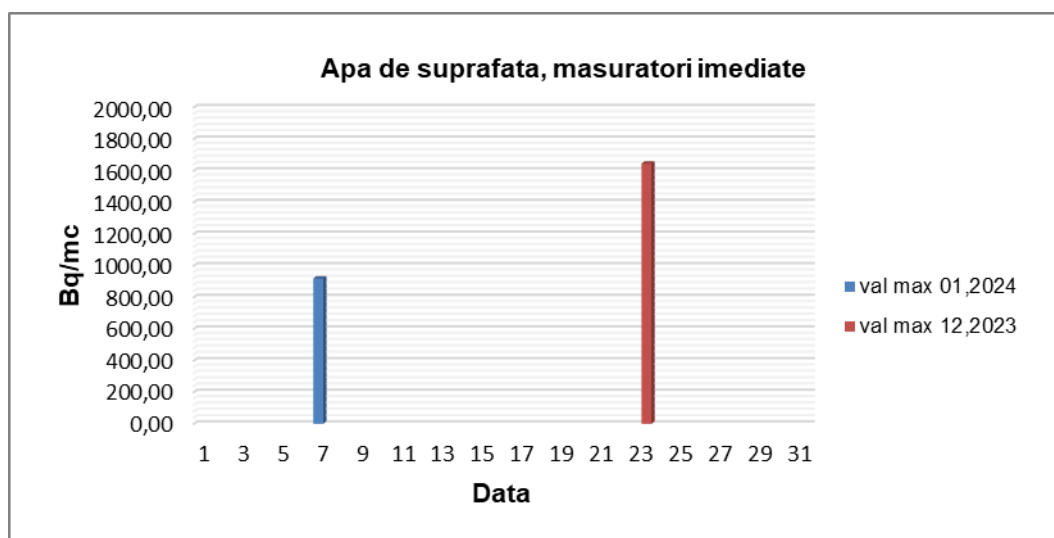
Graficul nr. 10.- Apa de suprafață - activitate specifică beta globală
