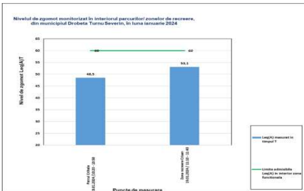
Graficul nr. 16-Nivelul de zgomot în interiorul parcurilor / zonelor de recreere, de pe raza municipiului Drobeta Turnu Severin, în luna ianuarie 2024
