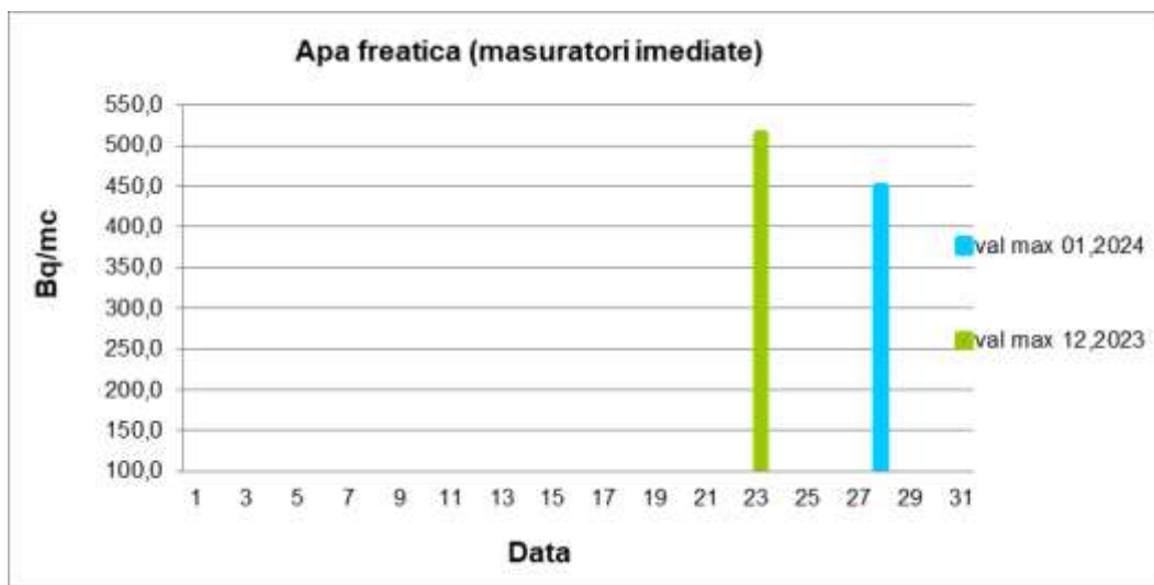
Graficul nr. 12.- apa freatică - activitate specifică beta globală
