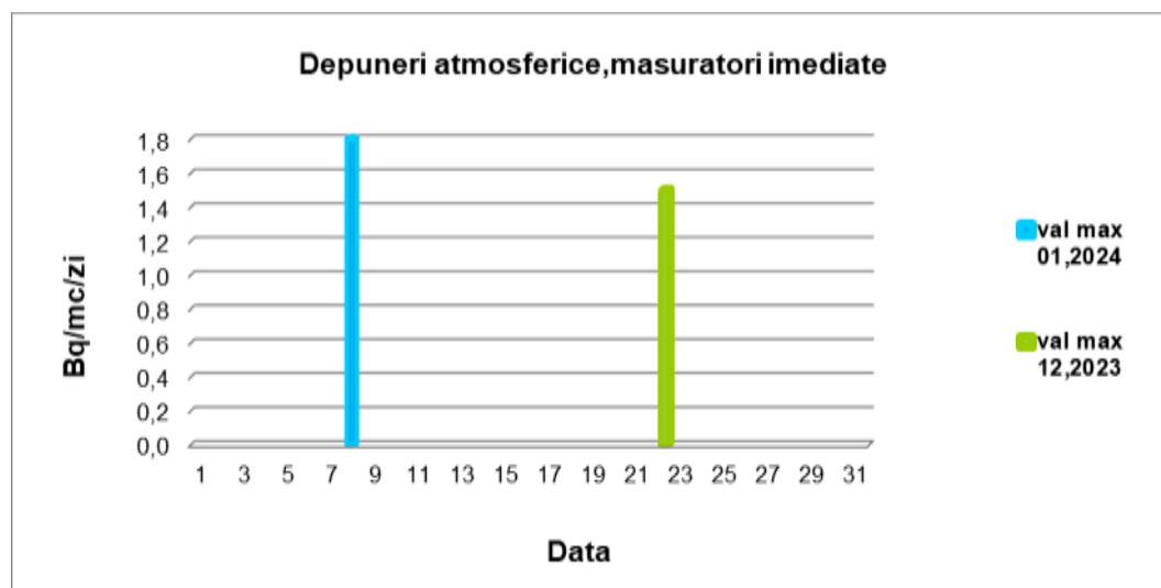
Graficul nr. 8- Depuneri atmosferice imediate - activitate specifică beta globală
