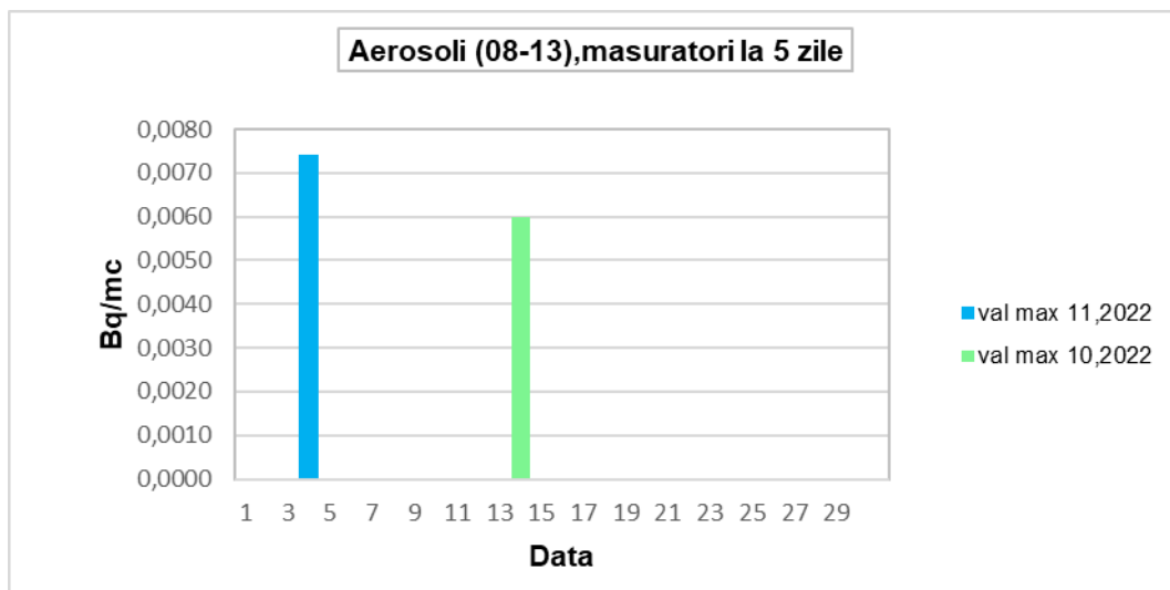
Graficul nr. 22.- Aerosoli atmosferici - activitate specifică beta globală - intervalul 08-13
