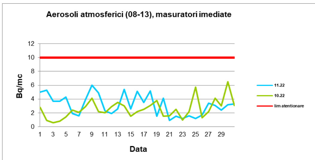
Graficul nr. 20.- Aerosoli atmosferici - activitate specifică beta globală - intervalul 08-13
