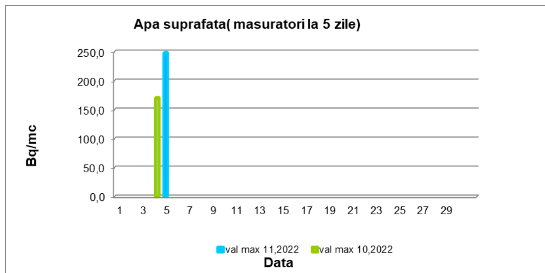
Graficul nr. 26.- apa de suprafață - activitate specifică beta globală
