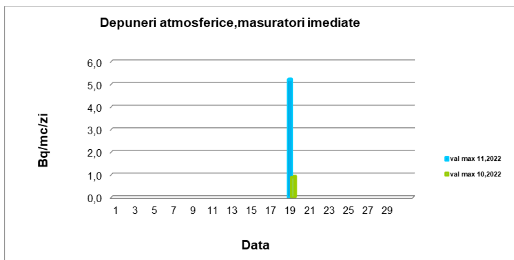
Graficul nr. 23- Depuneri atmosferice imediate - activitate specifică beta globală
