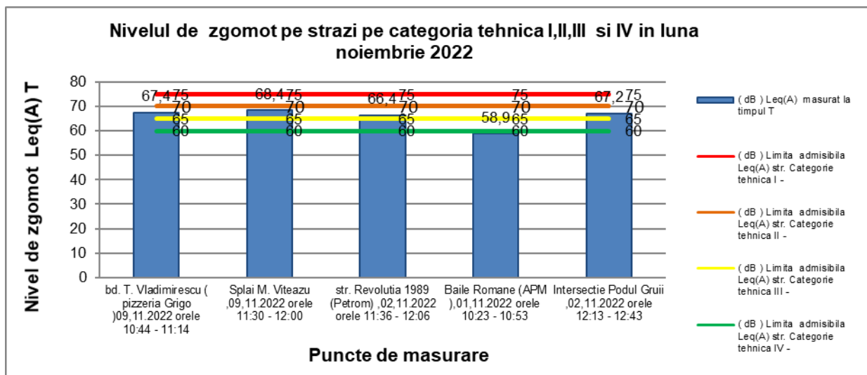
Graficul nr. 16-. Nivel de zgomot urban pe strazi de categorie tehnică I, II, III si IV în municipiul Drobeta Turnu Severin
