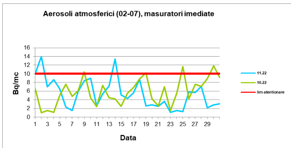
Graficul nr. 19.- Aerosoli atmosferici - activitate specifică beta globală - intervalul 02-07
