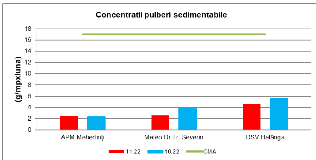
Graficul nr. 14 -Concentrațiile pulberilor sedimentabile
