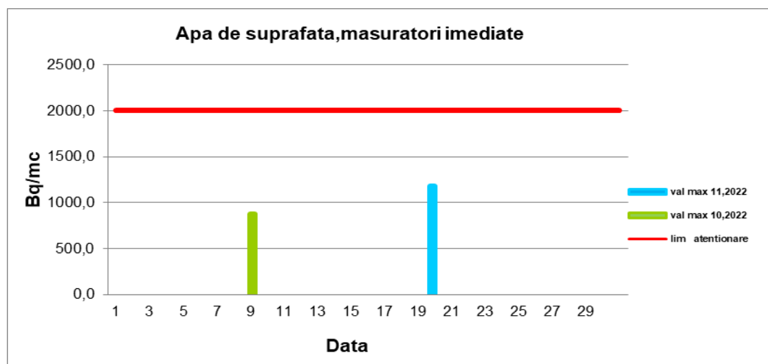
Graficul nr. 25.- Apa de suprafață - activitate specifică beta global
