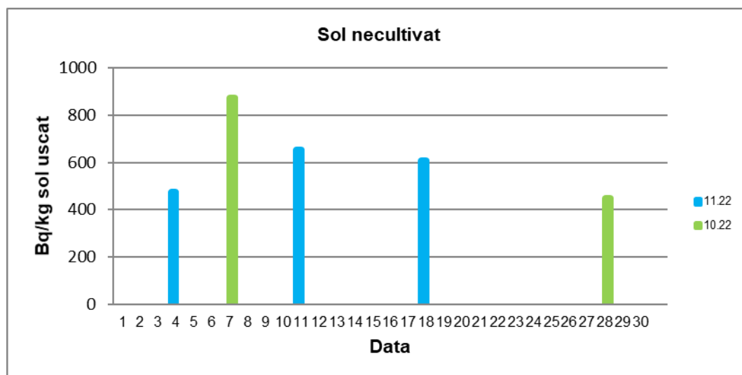
Graficul nr. 29- sol necultivat - activitate specifică beta globală
