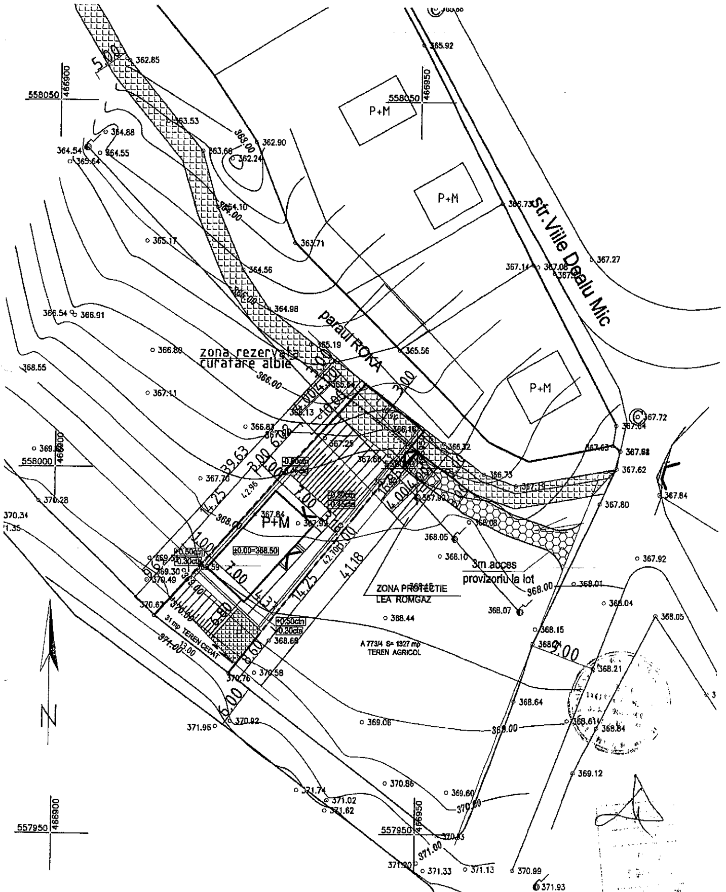
PLAN DE SITUATIE sc.1:500
