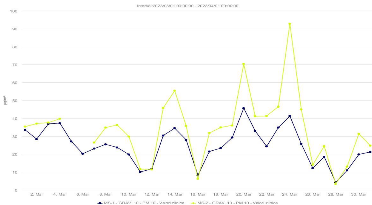
Evoluția valorilor medii zilnice ale indicatorului particule în suspensie, PM 10 gravimetric, la stațiile de monitorizare din județul Mureș
