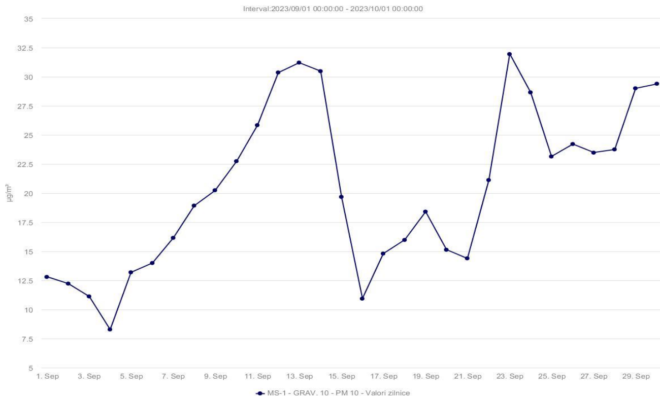
Evoluția valorilor medii zilnice ale indicatorului particule în suspensie, PM 10 gravimetric, la stația MS-1 din județul Mureș
