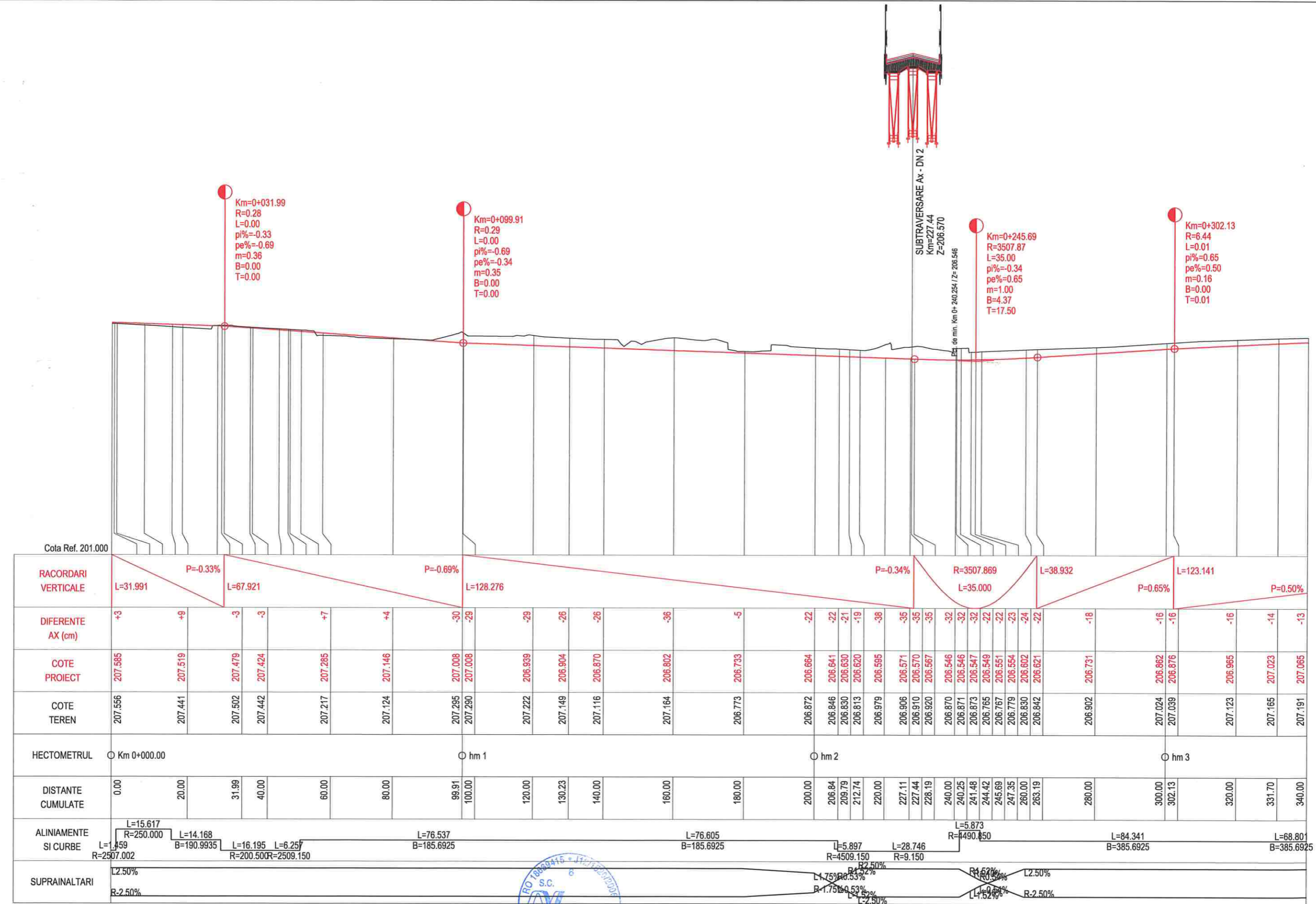
PROFIL LONGITUDINAL Ax - Bretea 2 DE LA 0.000 LA 340.000 SCARA : ORIZ 1 :1000 VERT 1 :100
