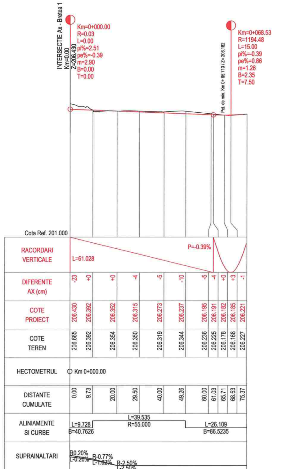
PROFIL LONGITUDINAL Str. Nordului DE LA 0.000 LA 75.372 SCARA : ORIZ 1 :1000 VERT 1 :100
