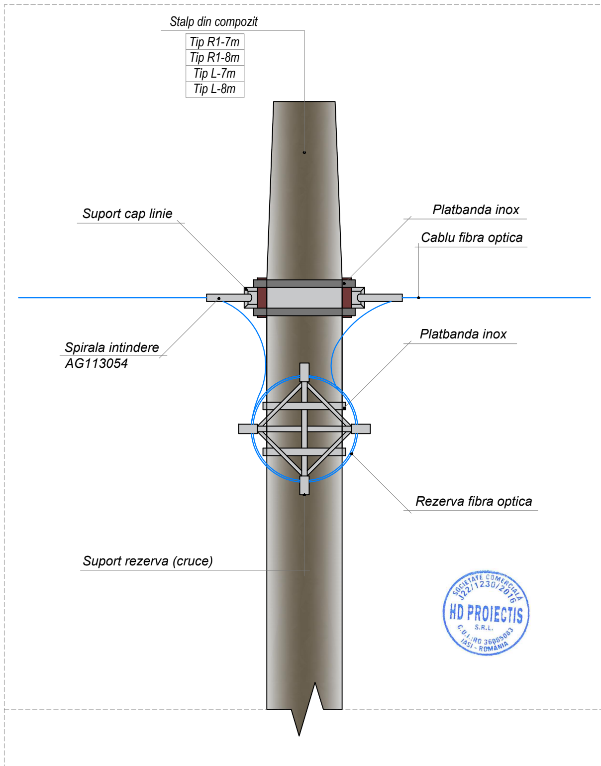
detaliu stalp din compozit cu rezerva de fibra optica
