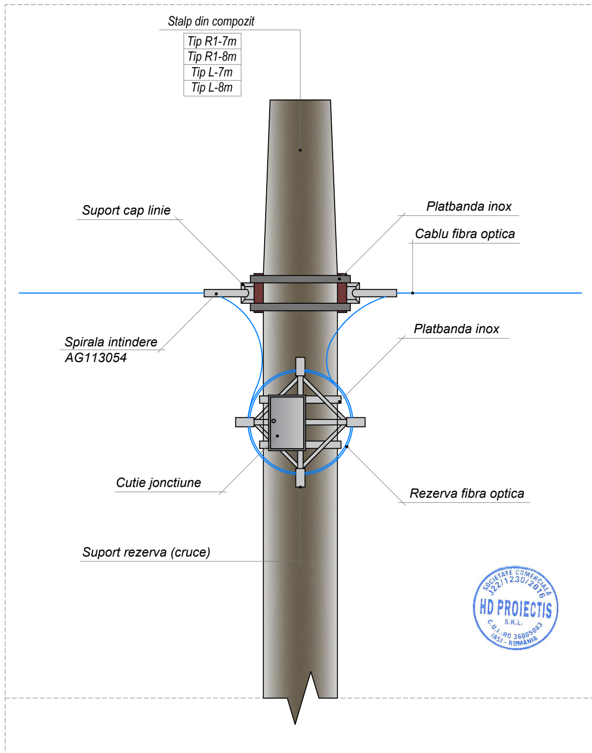
detaliu stalp din compozit cu rezerva de fibra optica si cutie de jonctiune
