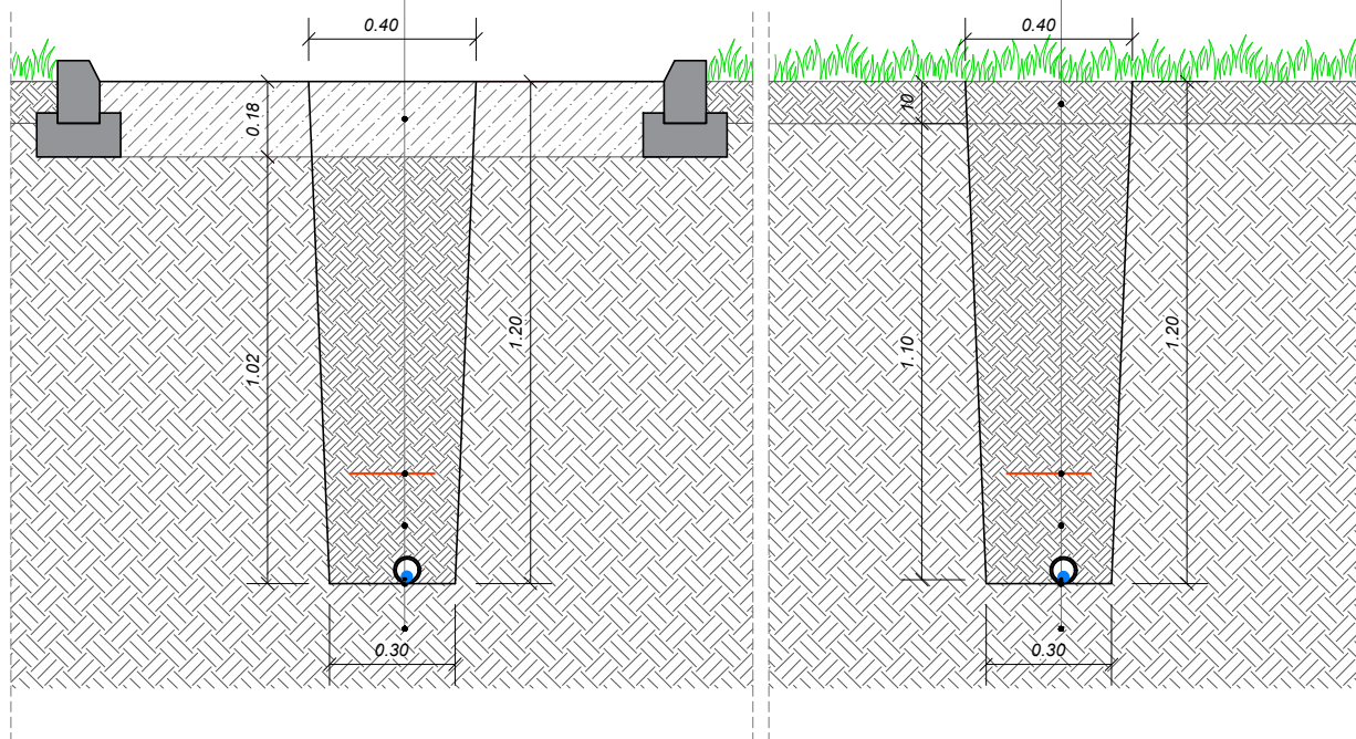
SECTIUNE TRANSVERSALA PRIN SANT IN TROTUAR
