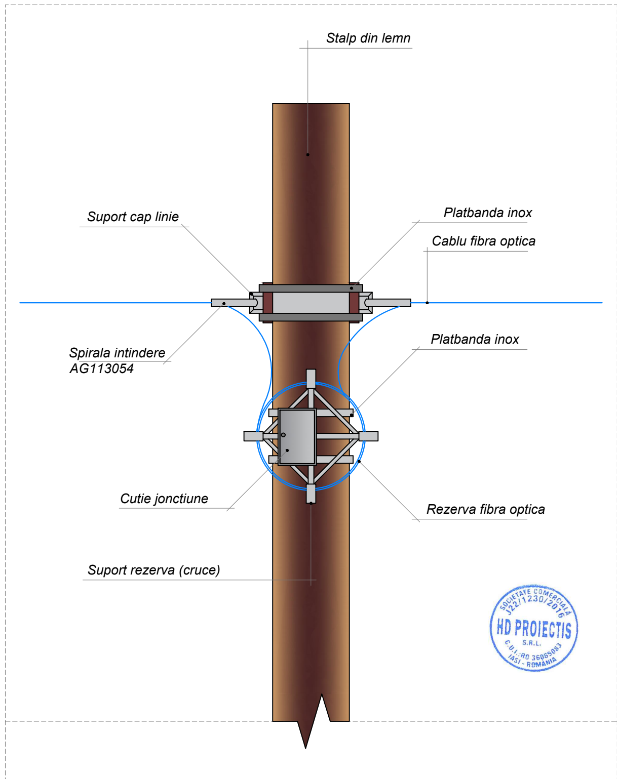
detaliu stalp din lemn cu rezerva de fibra optica si cutie de jonctiune
