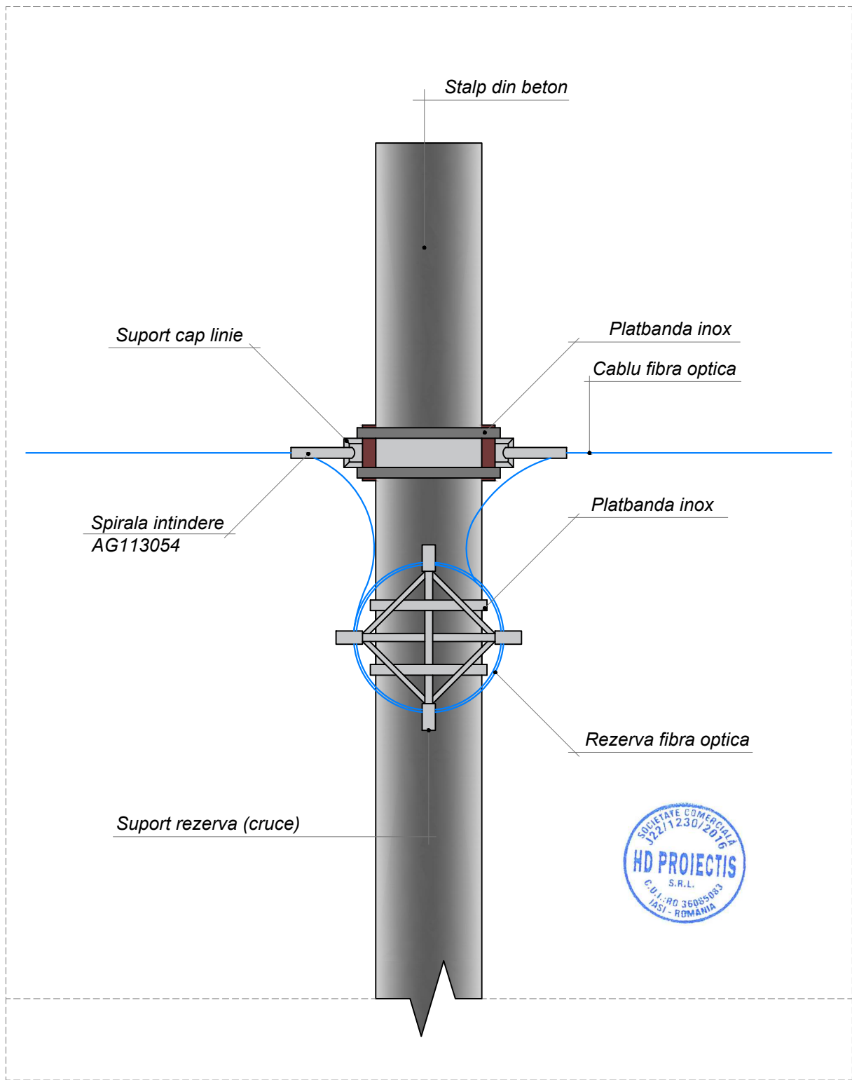
detaliu stalp din lemn cu rezerva de fibra optica
