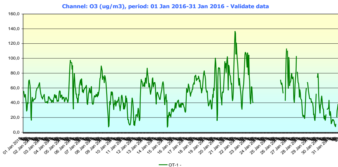
Fig. 1.3. Evoluție valori maxime zilnice ale mediilor pe 8 ore pentru ozon- luna ianuarie 2016
