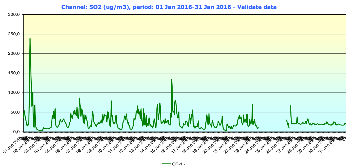
Fig. 1.2 Evoluție valori medii orare SO 2 la stația automata din județul Olt – luna ianuarie 2016
