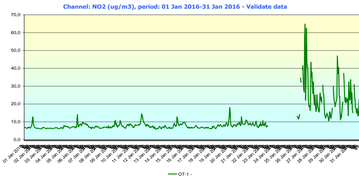
Fig. 1.4 Evoluție valori medii orare \text{NO}_2 la stația automată din județul Olt – luna ianuarie 2016
