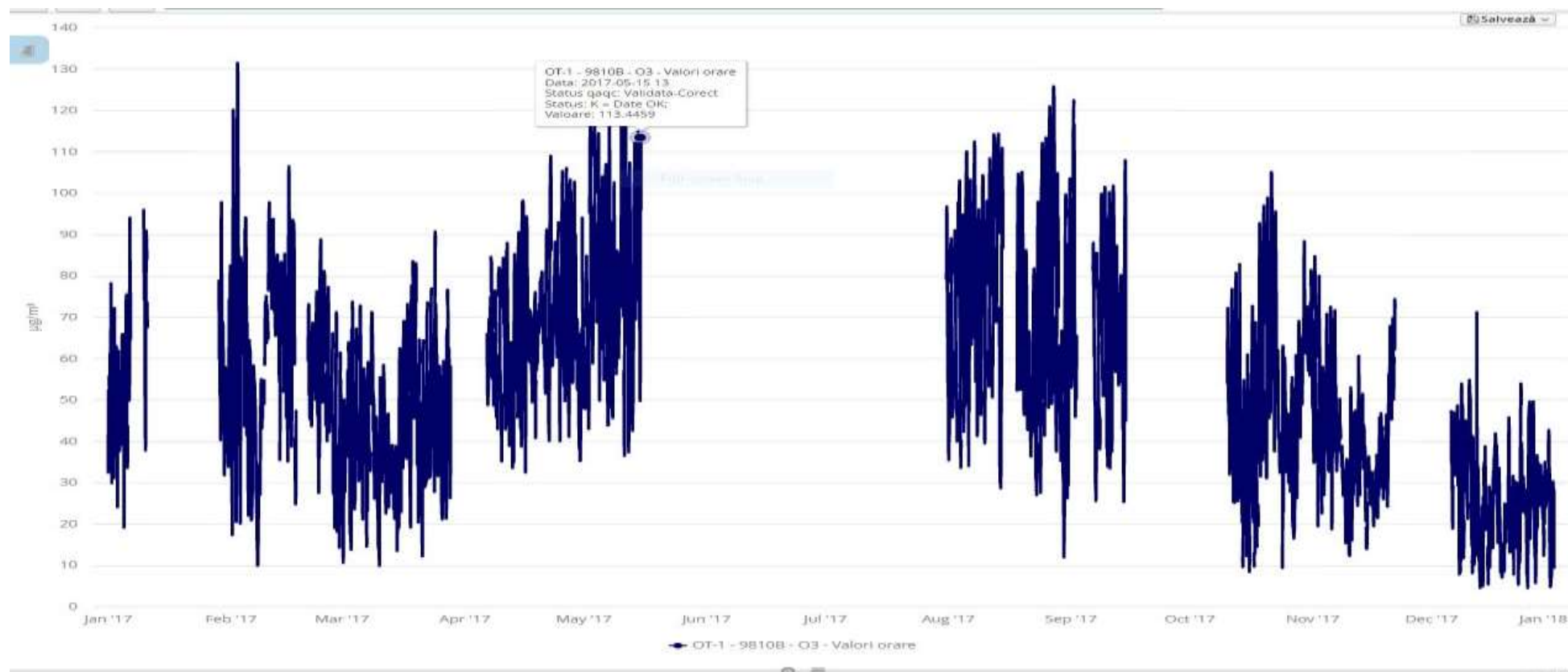
Fig.1.3.1 Evoluția concentrațiilor orare la indicatorul monoxid de carbon în anul 2017
