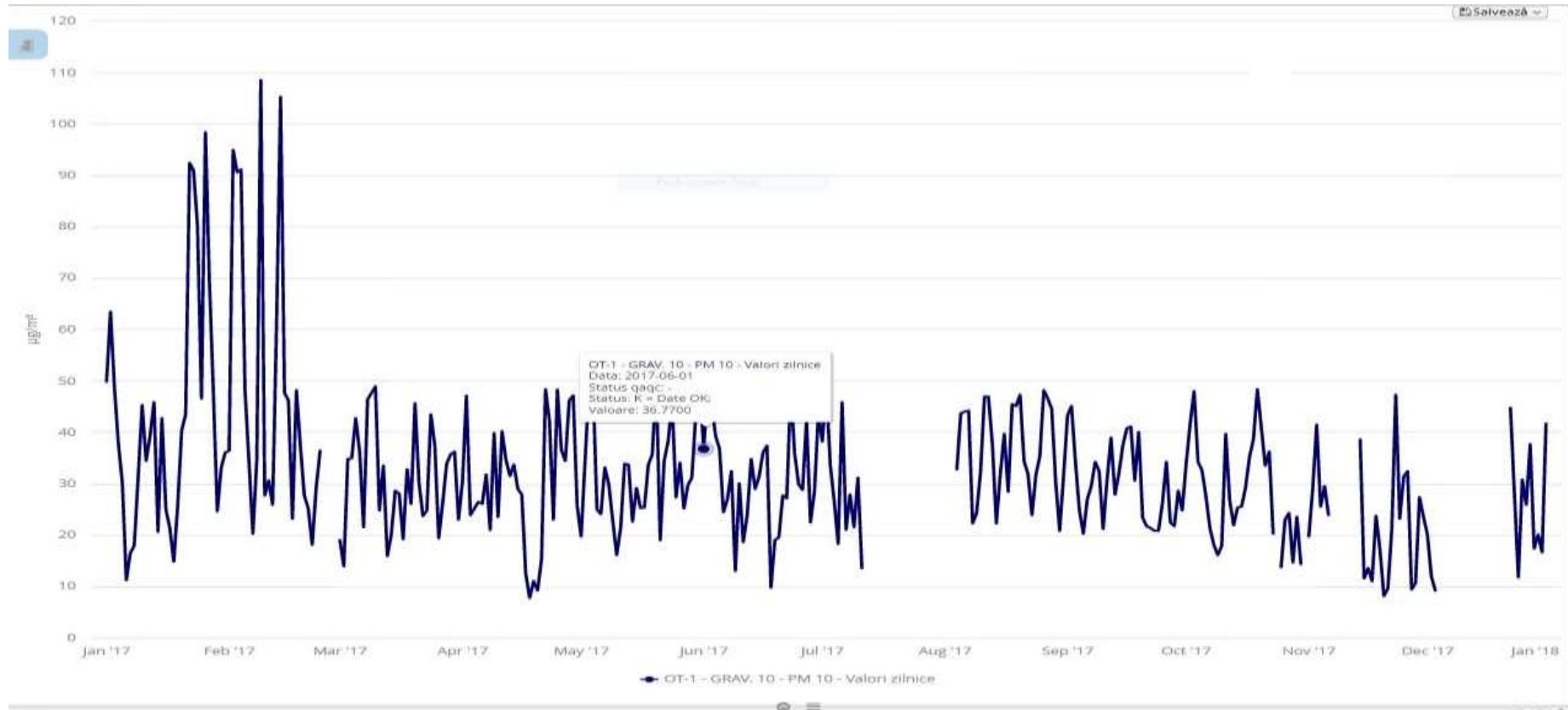
Fig. 1.4.1. Evoluția concentrațiilor medii zilnice la pulberi PM10 determinate gravimetric în anul 2017
