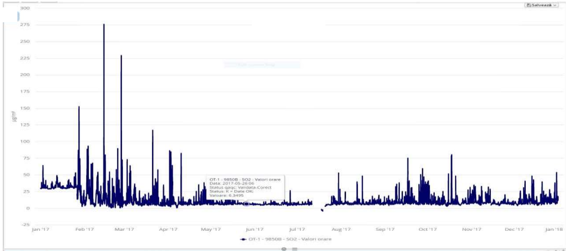
Fig. 1.1.2. Concentrații medii orare de NO 2 în anul 2017
