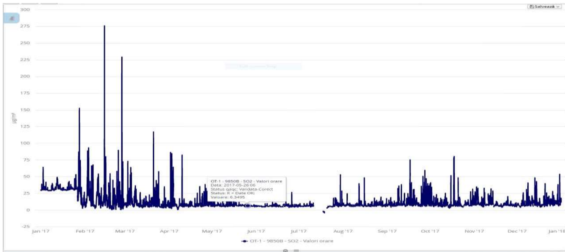
Fig. 1.1.1. Concentrații medii orare de SO 2 în anul 2017
