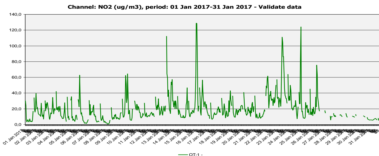
Fig. 1.4 Evoluție valori medii orare \text{NO}_2 la stația automată din județul Olt – luna ianuarie 2017
