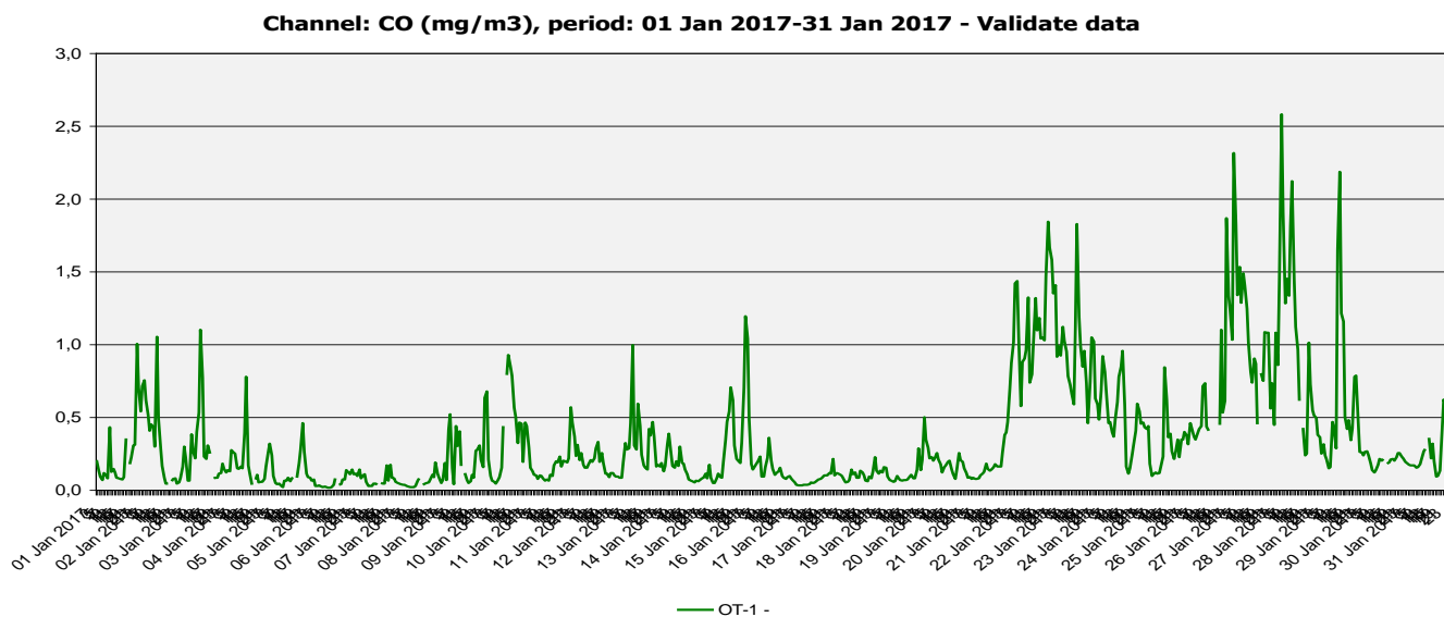
Fig. 1.5. Evoluție valori medii orare pentru CO - luna ianuarie 2017
