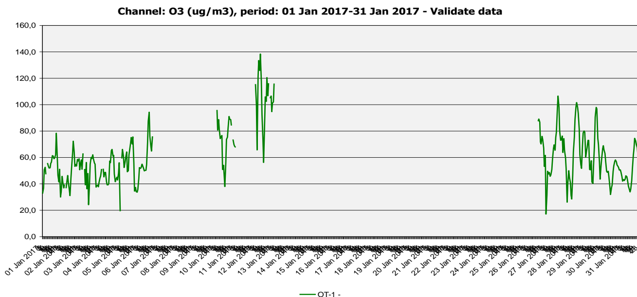
Fig. 1.3. Evoluție valori medii orare pentru ozon - luna ianuarie 2017
