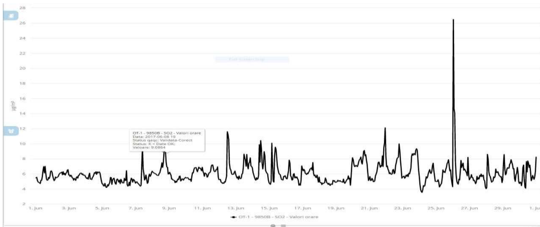
Fig. 1.2 Evoluție valori medii orare SO 2 la stația automata din județul Olt – luna iunie 2017
