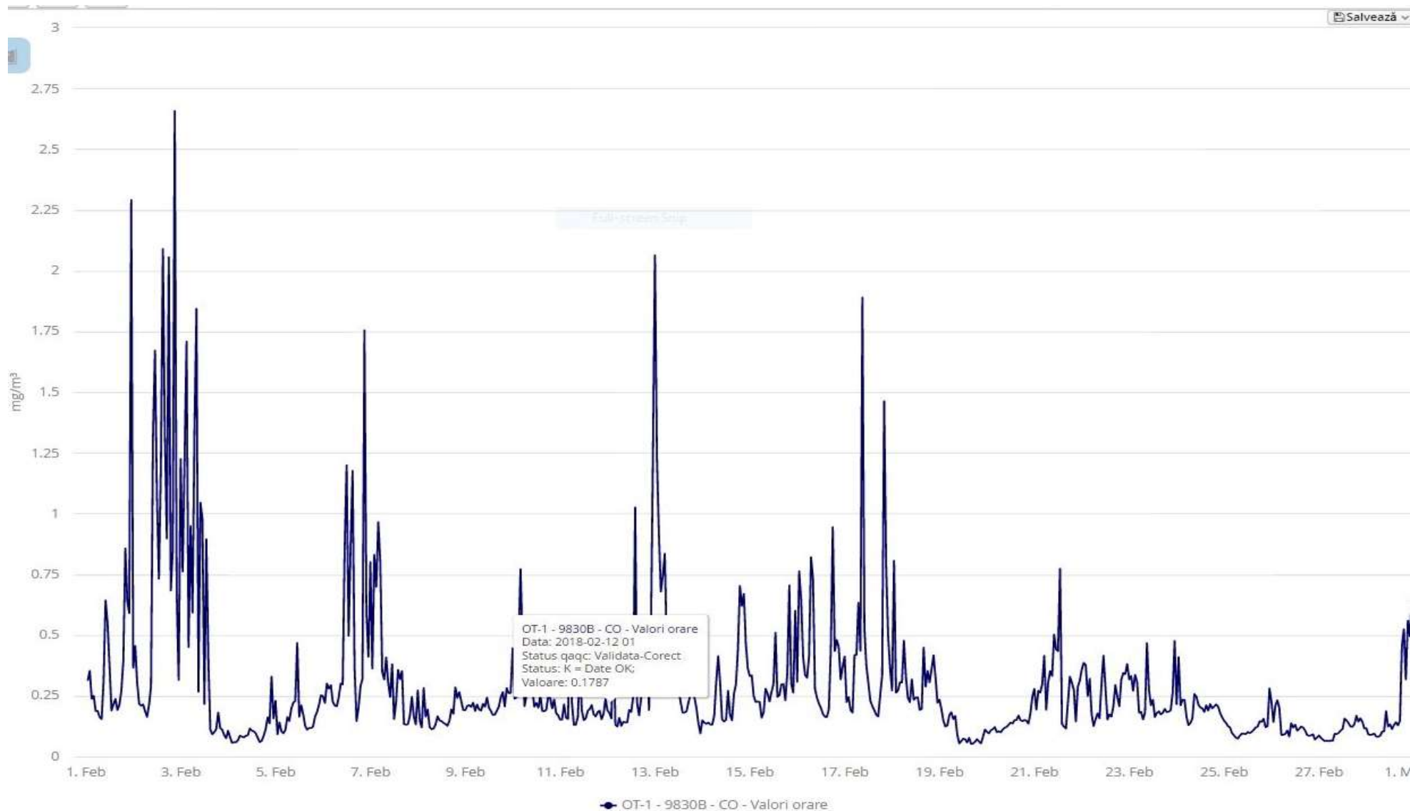
Fig. 1.4 Evoluție valori medii orare pentru CO - luna februarie 2018
