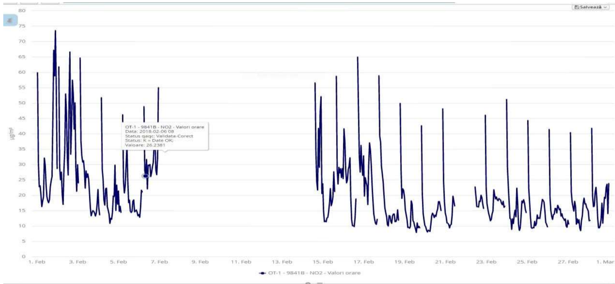
Fig. 1.3 Evoluție valori medii orare NO 2 la stația automată din județul Olt – luna februarie 2018 (lipsă date în perioada 7-15 februarie, cauza: analizorul de NO 2 defect ).
