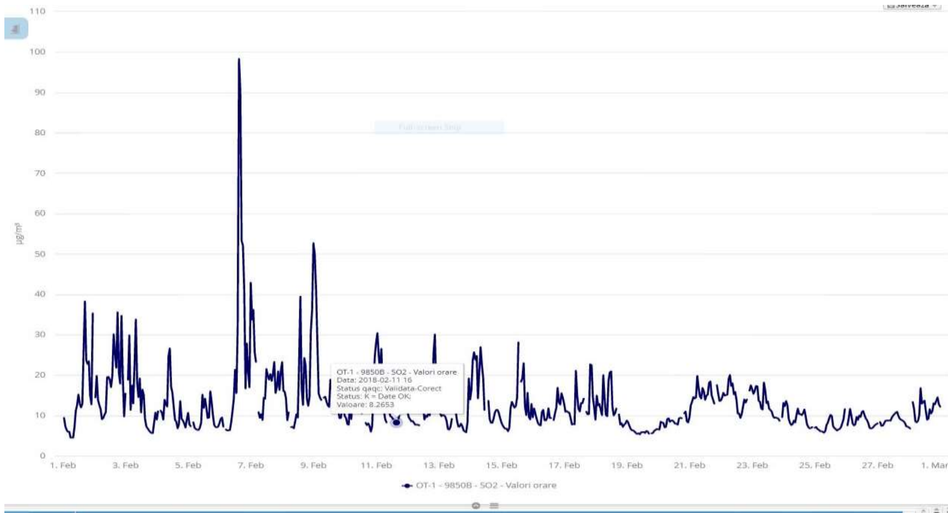
Fig. 1.2 Evoluție valori medii orare SO 2 la stația automată din județul Olt – luna februarie 2018.
