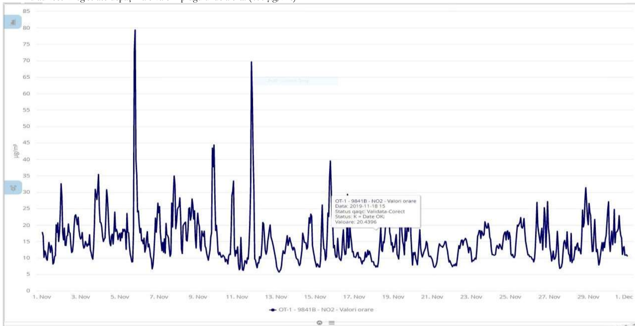
Fig. 1.4. Evoluția valorilor medii orare pentru dioxidul de azot NO 2 pentru luna noiembrie 2019
