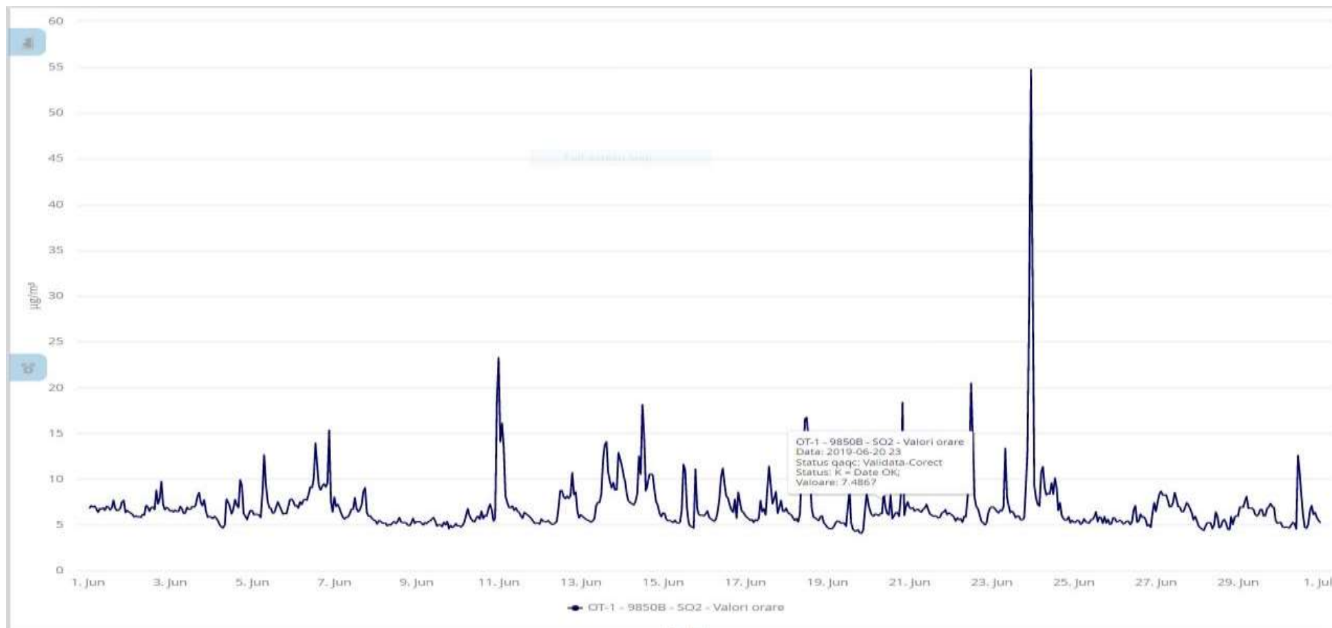
Fig. 1.3 Evoluție valori medii orare SO 2 la stația automata din județul Olt – luna iunie 2019.
