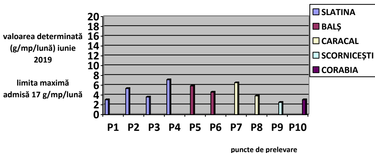
Fig. 1.9. Valori determinate pulberi sedimentabile
