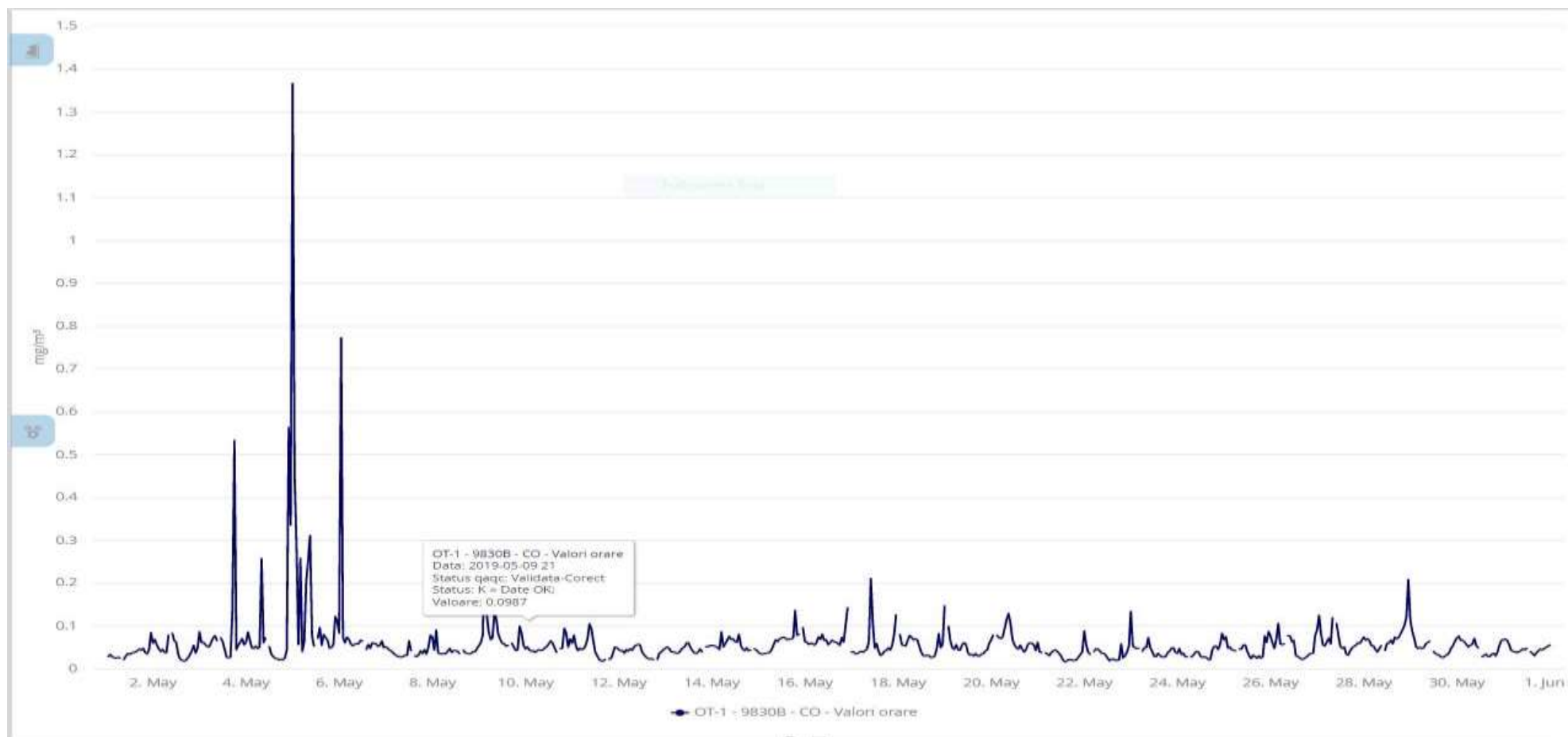
Fig. 1.5 Evoluție valori medii orare pentru CO - luna mai 2019
