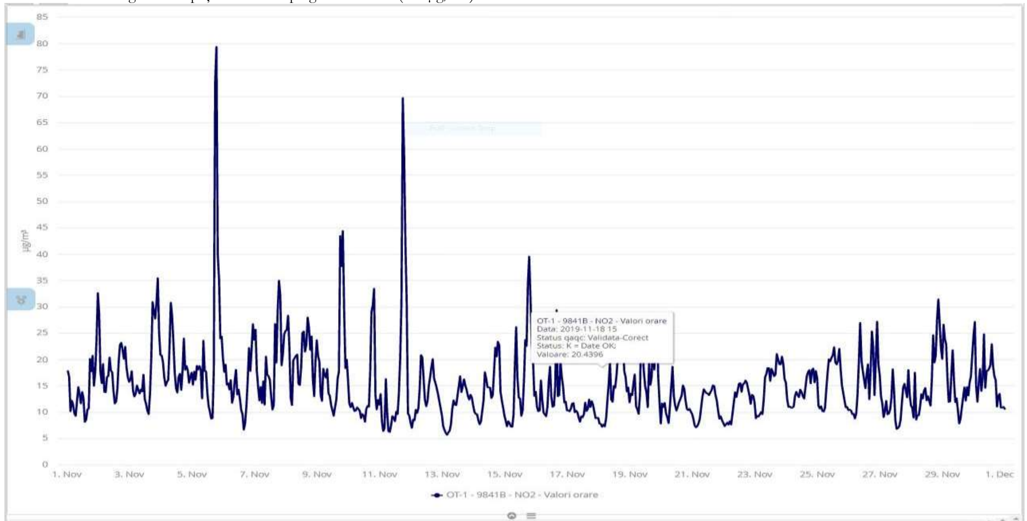
Fig. 1.4. Evoluția valorilor medii orare pentru dioxidul de azot NO 2 pentru luna noiembrie 2019
