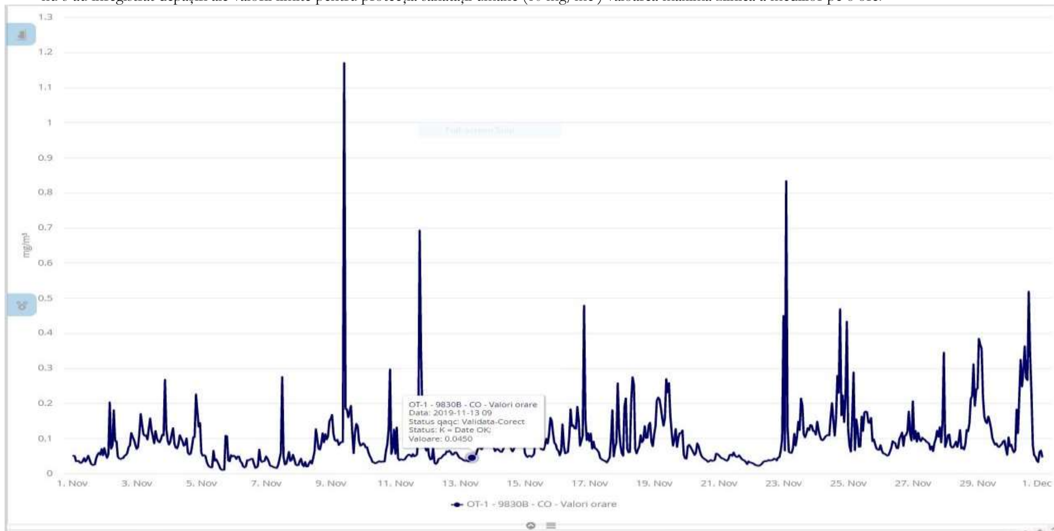
Fig. 1.5 Evoluție valori medii orare pentru CO - luna noiembrie 2019
