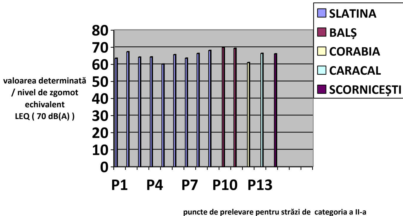
Fig. 1.11 Determinări sonometrice pe străzi de categoria a II-a
