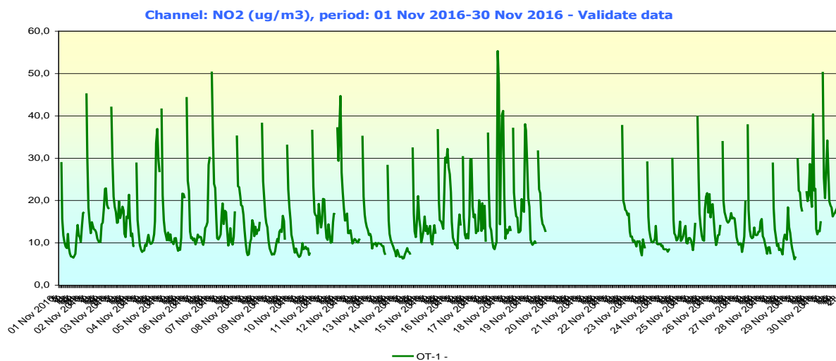
Fig. 1.4 Evoluție valori medii orare NO 2 la stația automată din județul Olt – luna noiembrie 2016 În perioada 21-23 noiembrie 2016 lipsă achiziție date pentru NO 2 .
