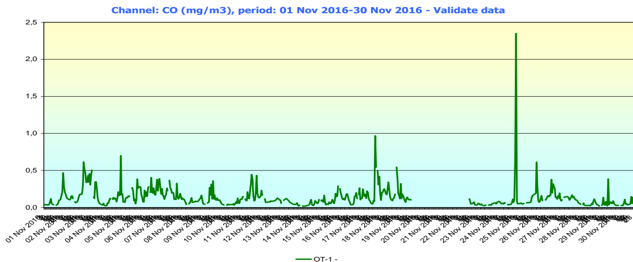
Fig. 1.3. Evoluție valori medii orare pentru CO - luna noiembrie 2016 În perioada 21-23 noiembrie 2016 lipsă achiziție date pentru CO.
