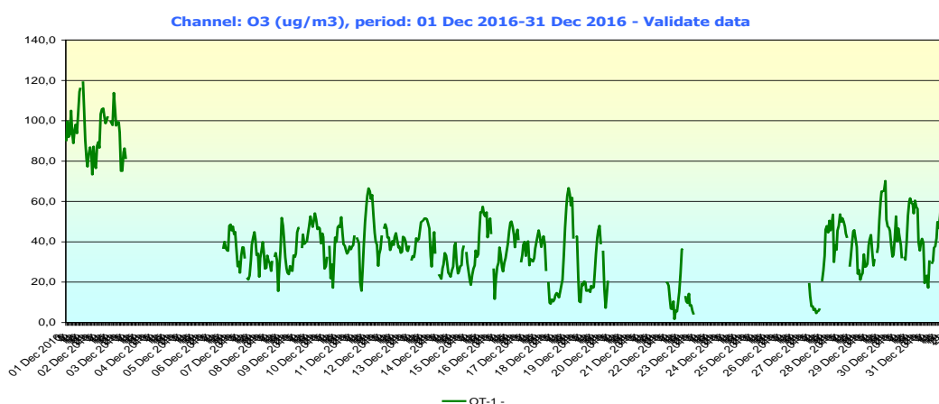
Fig. 1.3. Evoluție valori maxime zilnice ale mediilor pe 8 ore pentru ozon- luna decembrie 2016
