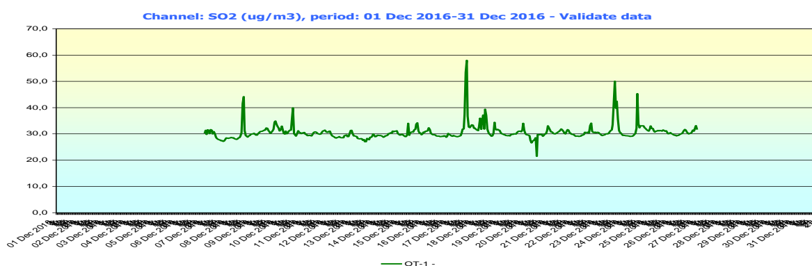
Fig. 1.2 Evoluție valori medii orare SO 2 la stația automata din județul Olt – luna decembrie 2016 În perioada 1-8 decembrie și 28-31 decembrie 2016 lipsă achiziție date.
