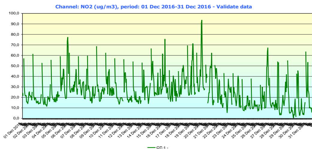
Fig. 1.4 Evoluție valori medii orare \text{NO}_2 la stația automată din județul Olt – luna decembrie 2016
