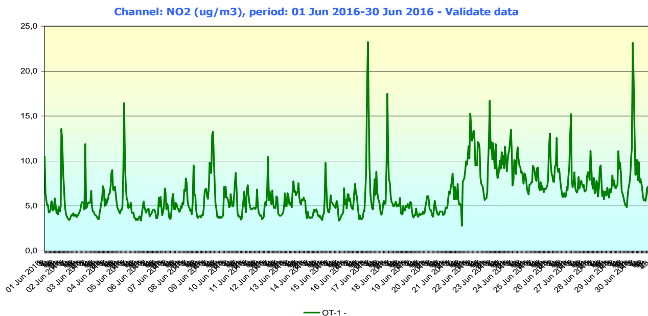
Fig. 1.4 Evoluție valori medii orare \text{NO}_2 la stația automată din județul Olt – luna iunie 2016
