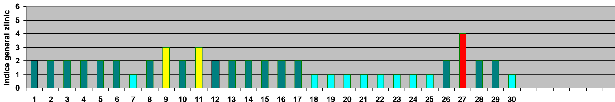
Fig.1.2. Evoluția indicelui general de calitate a aerului în luna NOIEMBRIE 2022 la stația OT-1 (Slatina, Aleea Grădiște F.N.)
