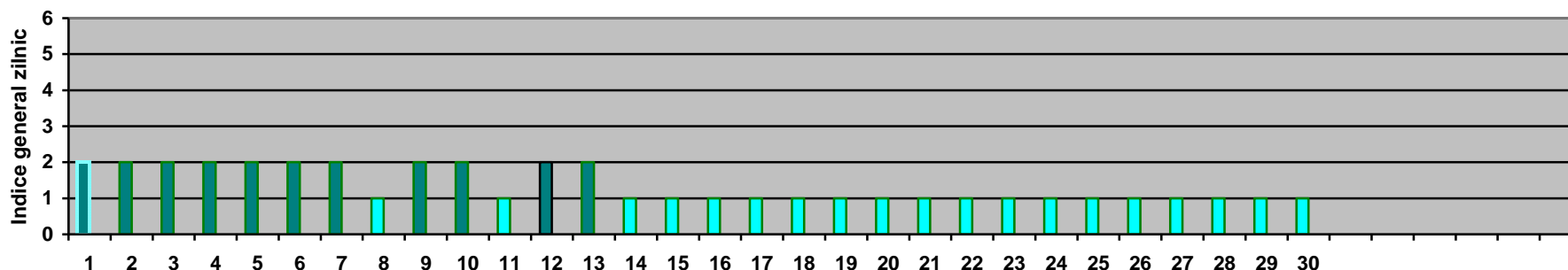
Fig.1.3 Evoluția indicelui zilnic general de calitate a aerului în luna NOIEMBRIE 2022 la stația OT-2 (Slatina, Aleea Muncii, nr 4)
