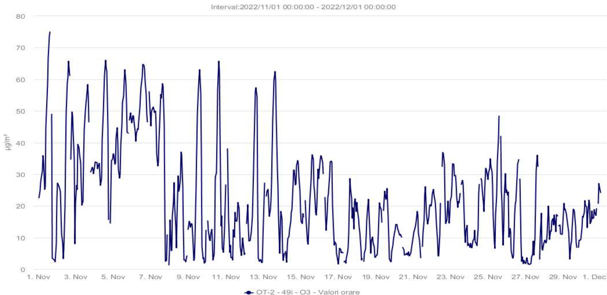
Fig. 1.7. Evoluție valori medii orare pentru O_3 - luna NOIEMBRIE 2022
