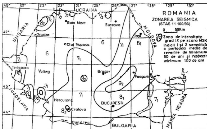
Fig. 3. Zonarea seismică a teritoriului României Intensități pe scara MSK, conform SR 11100–1:93 Zonarea seismică.
