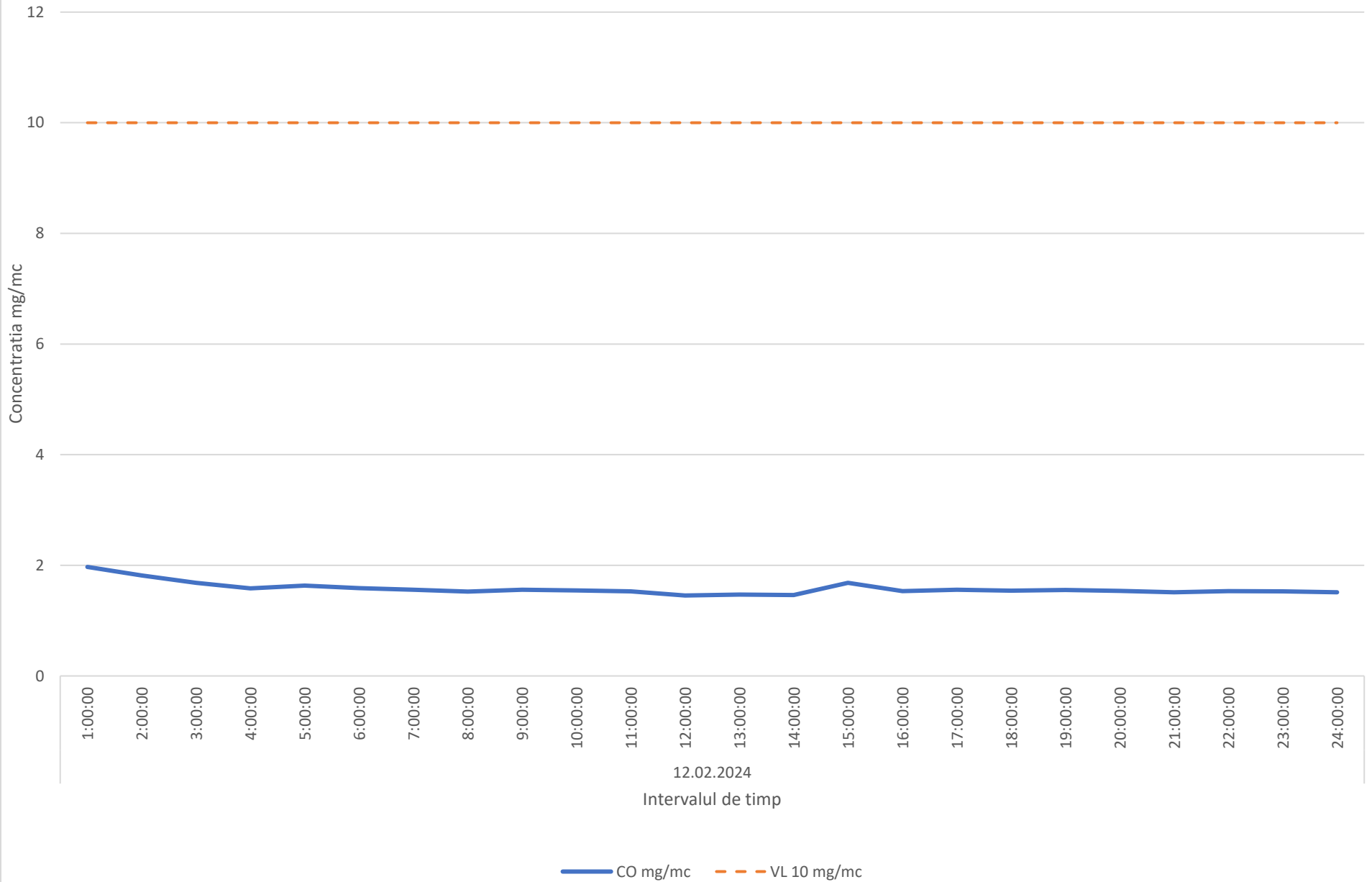
Variatia mediilor orare ale indicatorului CO in data de 12.02.2024 - Parcul Central, Municipiul Ploiesti
